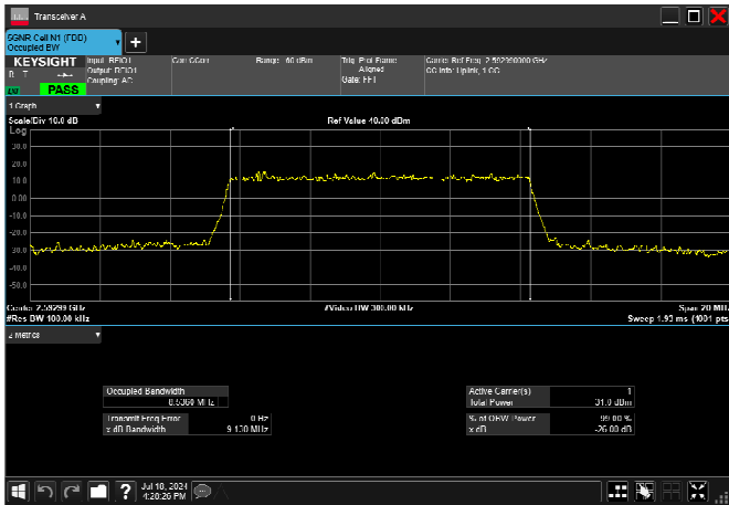
n41_10MHz_30kHz_2592.99MHz_CP-OFDM QPSK_RB24@0 8.573MHz
