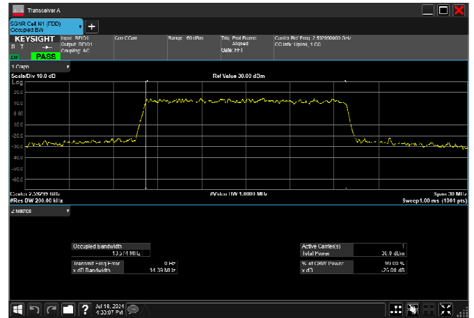
n41_20MHz_30kHz_2592.99MHz_DFT-s-OFDM \pi/2 BPSK_RB50@0 18.100MHz
