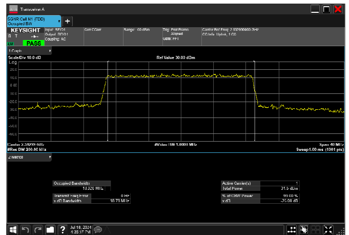
n41_20MHz_30kHz_2592.99MHz_DFT-s-OFDM 16 QAM_RB50@0 18.020MHz
