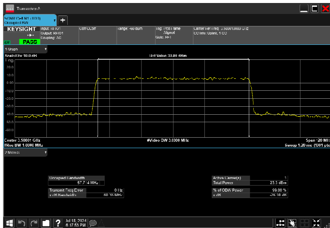
n77_1_70MHz_30kHz_3500MHz_DFT-s-OFDM QPSK_RB180@0 66.678MHz
