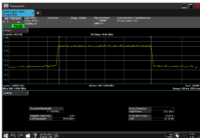
n77_3_80MHz_30kHz_3840MHz_DFT-s-OFDM QPSK_RB216@0 77.138MHz
