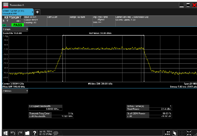
n78_1_15MHz_30kHz_3500MHz_DFT-s-OFDM QPSK_RB36@0 13.458MHz
