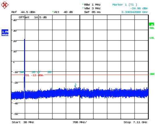
10MHz_High_QPSK_50@0 -24.96dBm
