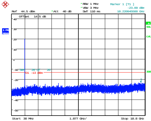
20MHz_Middle_QPSK_1@0 -23.09dBm
