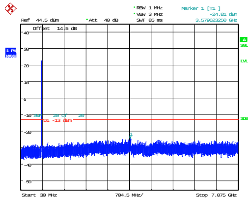
5MHz_Middle_QPSK_25@0 -24.81dBm
