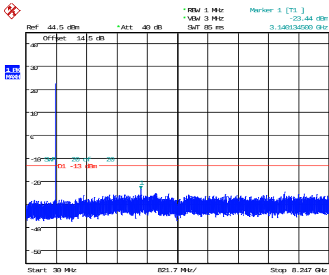
1.4MHz_Low_QPSK_1@0 -23.44dBm
