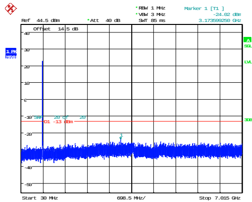
5MHz_Low_QPSK_25@0 -24.02dBm
