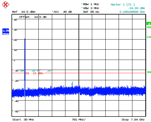
10MHz_Low_QPSK_50@0 -24.93dBm
