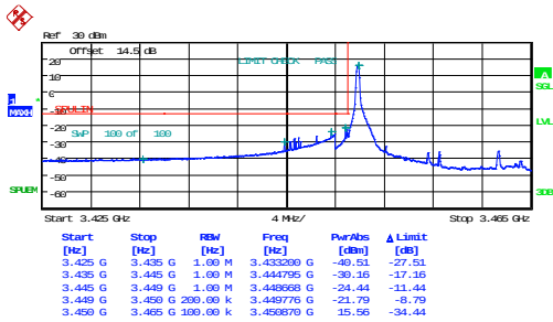
1_15MHz_Low_QPSK_1@0
