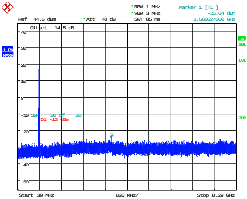
10MHz_Low_QPSK_50@0 -25.04dBm
