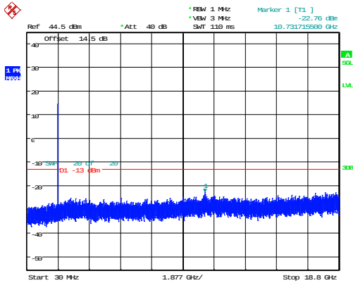
10MHz_Middle_QPSK_50@0 -22.76dBm
