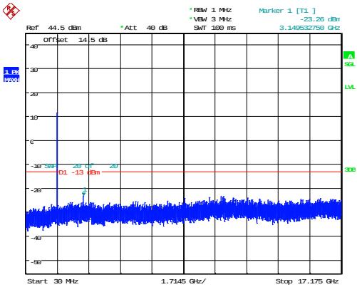
15MHz_Low_QPSK_75@0 -23.26dBm
