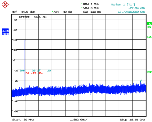
10MHz_Low_QPSK_1@0 -22.34dBm
