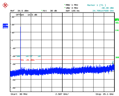
20MHz_Low_QPSK_1@0 -30.39dBm
