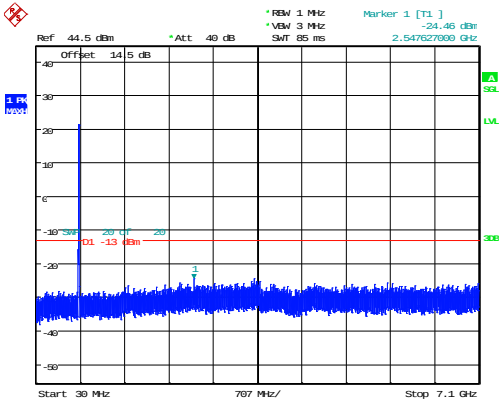
10MHz_Middle_QPSK_50@0 -24.46dBm
