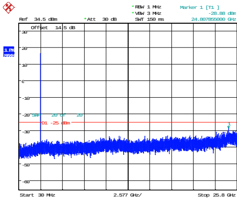
20MHz_Low_QPSK_1@0 -28.88dBm
