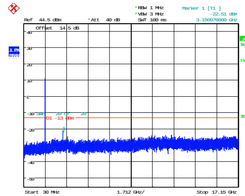
10MHz_Low_QPSK_50@0 -22.51dBm
