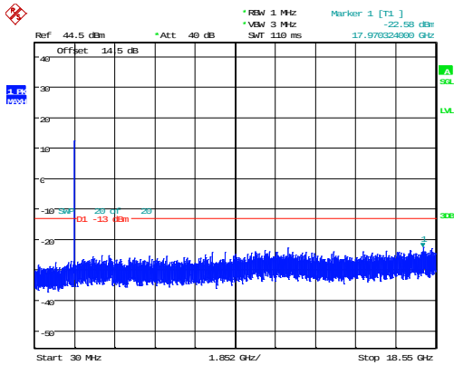
10MHz_Low_QPSK_50@0 -22.58dBm
