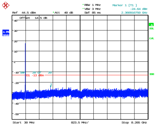
5MHz_Low_QPSK_25@0 -24.64dBm
