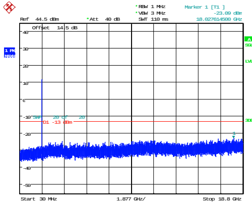
20MHz_Middle_QPSK_100@0 -23.09dBm
