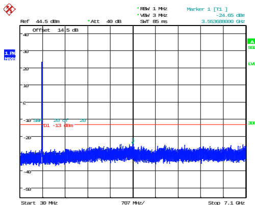
5MHz_Middle_QPSK_25@0 -24.65dBm
