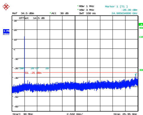
10MHz_Middle_QPSK_50@0 -28.39dBm
