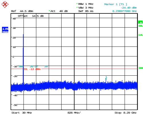
10MHz_Low_QPSK_1@0 -24.49dBm
