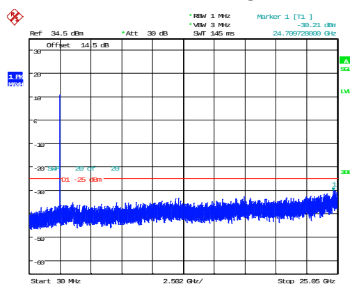
10MHz_Low_QPSK_50@0 -30.21dBm
