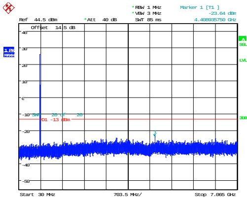
5MHz_Low_QPSK_1@0 -23.64dBm
