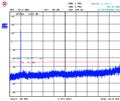
20MHz_Low_QPSK_100@0 -30.18dBm
