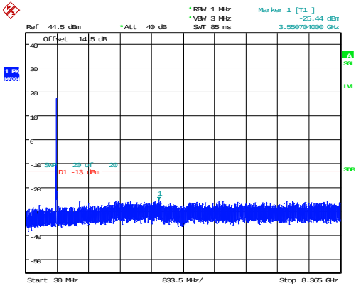
10MHz_Middle_QPSK_50@0 -25.44dBm
