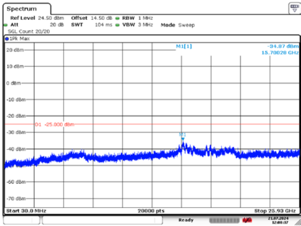
10MHz_Middle_QPSK_50@0 -34.87dBm
