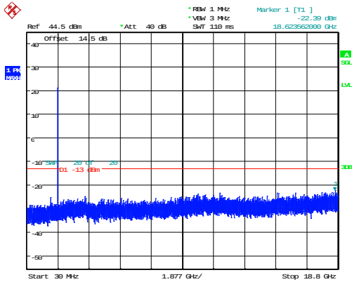
10MHz_Middle_QPSK_1@0 -22.39dBm
