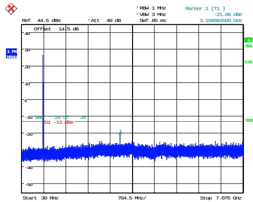
5MHz_Middle_QPSK_1@0 -21.86dBm
