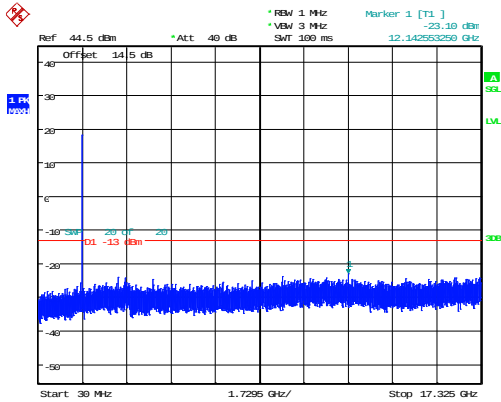
20MHz_Middle_QPSK_1@0 -23.10dBm
