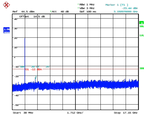
10MHz_Low_QPSK_1@0 -23.44dBm
