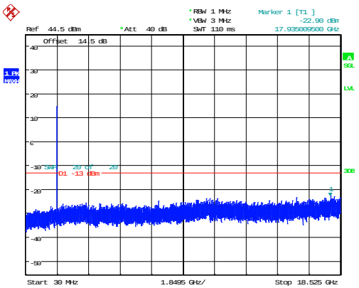
5MHz_Low_QPSK_25@0 -22.90dBm
