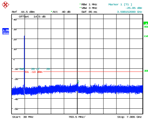
5MHz_Low_QPSK_25@0 -25.05dBm
