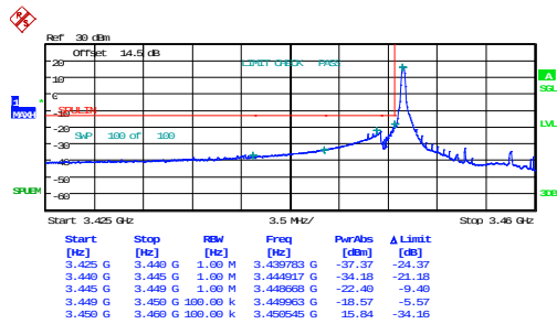
1_10MHz_Low_QPSK_1@0
