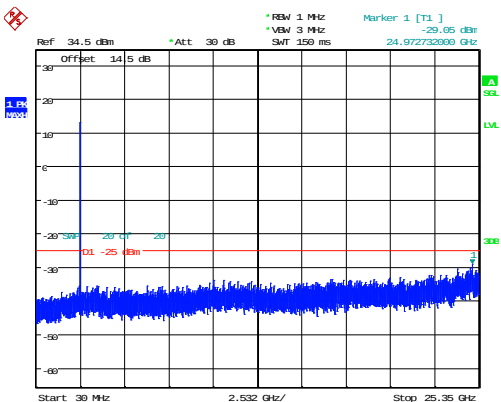
5MHz_Middle_QPSK_25@0 -29.05dBm
