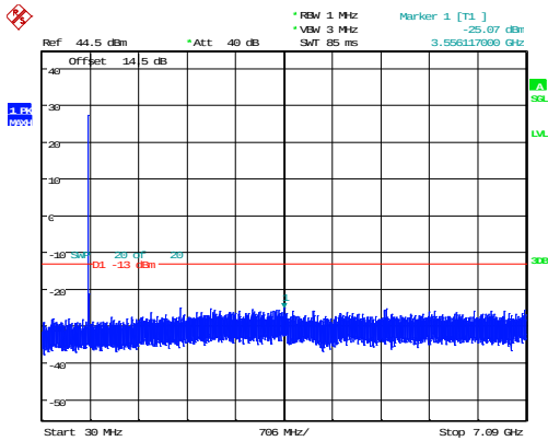
10MHz_Low_QPSK_1@0 -25.07dBm
