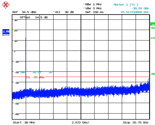
10MHz_Low_QPSK_50@0 -30.29dBm
