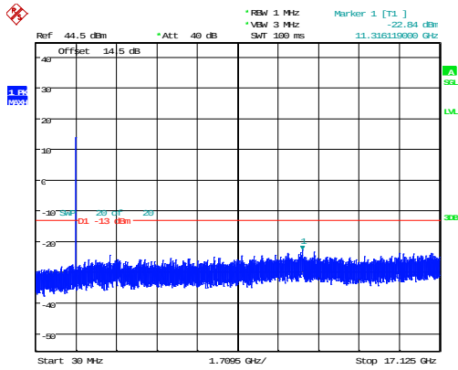
5MHz_Low_QPSK_25@0 -22.84dBm
