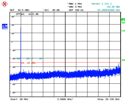
5MHz_Low_QPSK_25@0 -29.30dBm
