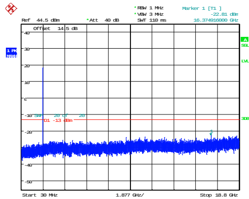
5MHz_Middle_QPSK_1@0 -22.81dBm
