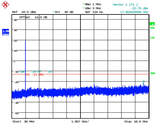
20MHz_Low_QPSK_1@0 -22.75dBm
