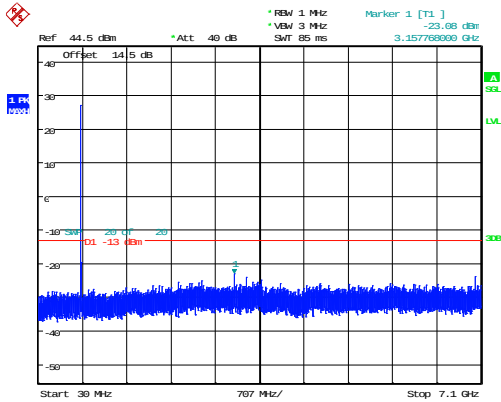
10MHz_Middle_QPSK_1@0 -23.08dBm
