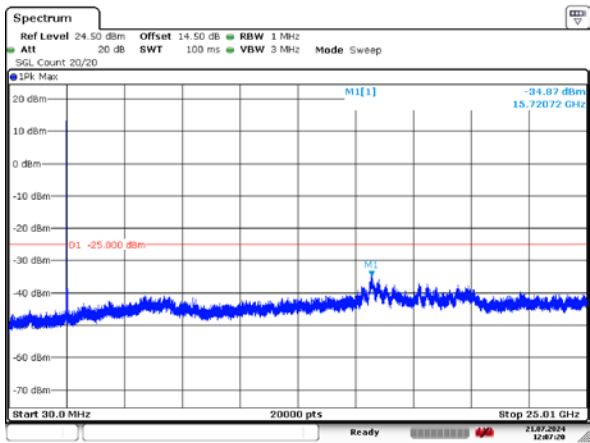
10MHz_Low_QPSK_50@0 -34.87dBm
