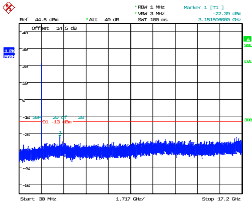
20MHz_Low_QPSK_1@0 -22.39dBm
