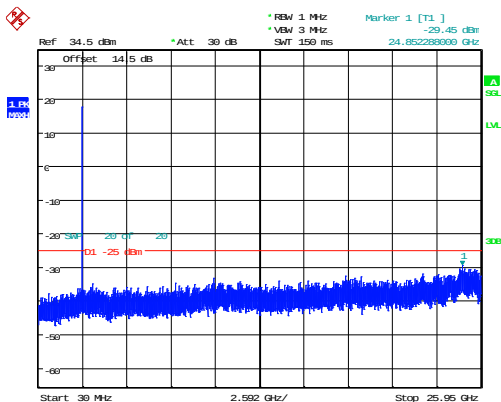
5MHz_Middle_QPSK_1@0 -29.45dBm
