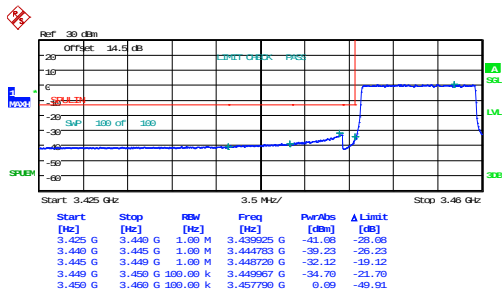
1_10MHz_Low_QPSK_50@0
