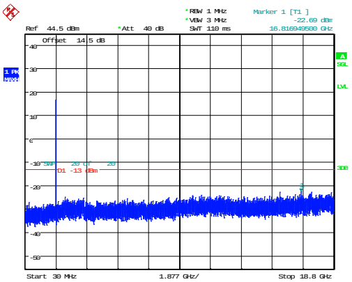
5MHz_Middle_QPSK_25@0 -22.69dBm
