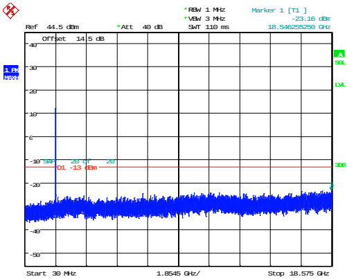
15MHz_Low_QPSK_75@0 -23.16dBm
