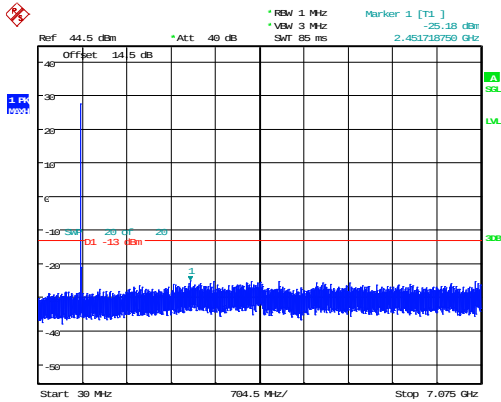
10MHz_Middle_QPSK_1@0 -25.18dBm
