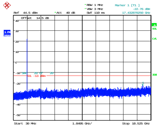
5MHz_Low_QPSK_1@0 -22.76dBm
