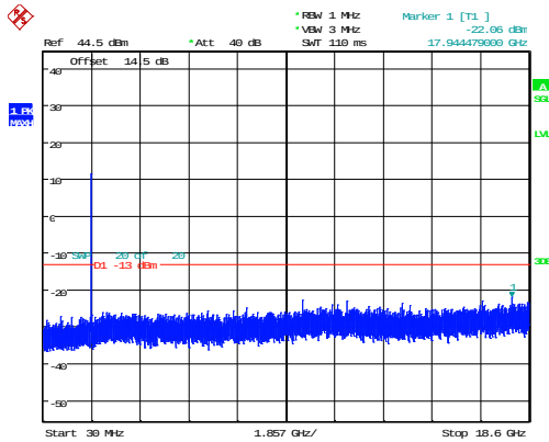
20MHz_Low_QPSK_100@0 -22.06dBm
