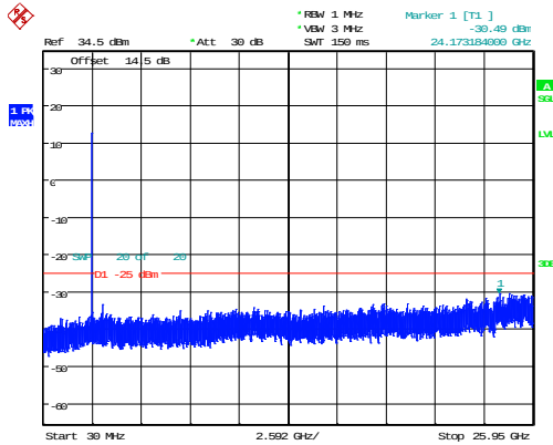
10MHz_Middle_QPSK_50@0 -30.49dBm
