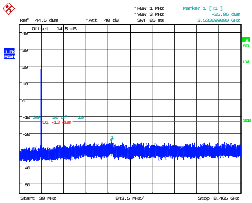
5MHz_High_QPSK_25@0 -25.06dBm
