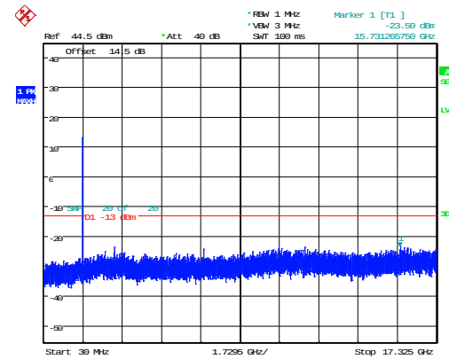
10MHz_Middle_QPSK_50@0 -23.50dBm
