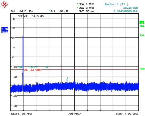
10MHz_Low_QPSK_50@0 -25.16dBm
