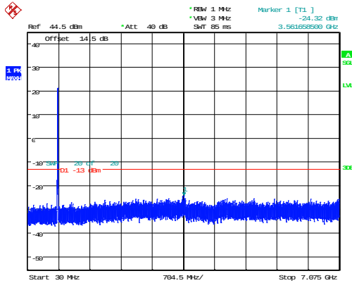
10MHz_Middle_QPSK_50@0 -24.32dBm
