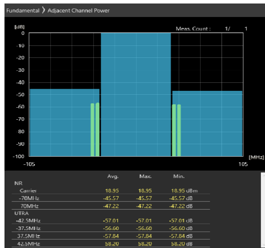
70MHz_30kHz_3665MHz-OFDM QPSK_RB90@45 -45.57,-47.22dB
