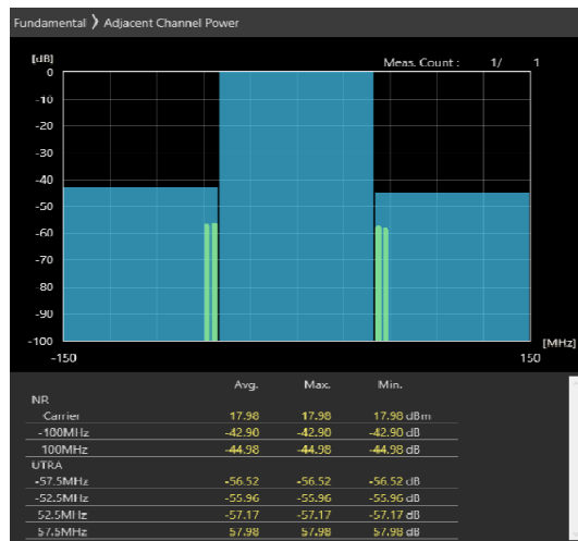
100MHz_30kHz_3650MHz-OFDM QPSK_RB270@0 -42.9,-44.98dB
