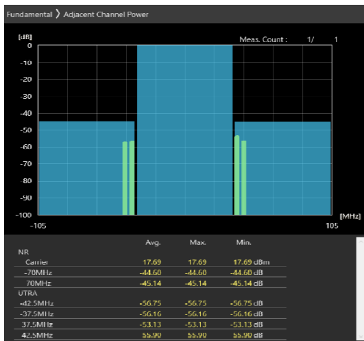
70MHz_30kHz_3665MHz-OFDM QPSK_RB1@188 -44.6,-45.14dB
