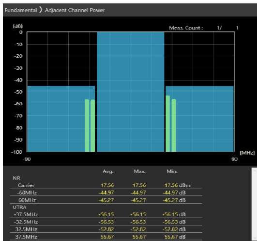
60MHz_30kHz_3670MHz-OFDM QPSK_RB1@161 -44.97,-45.27dB
