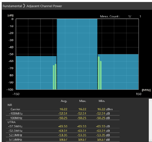
100MHz_30kHz_3650MHz-OFDM QPSK_RB1@272 -52.51,-50.25dB
