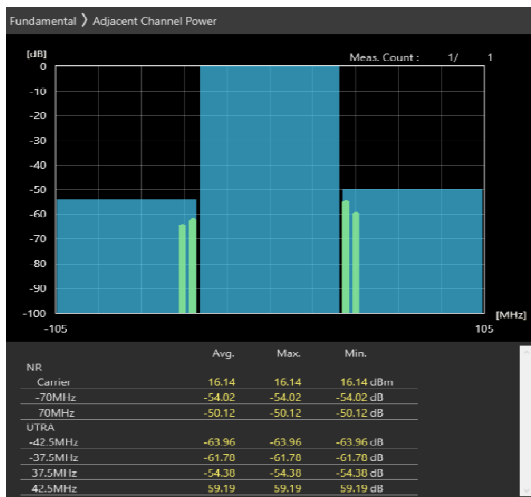
70MHz_30kHz_3665MHz-OFDM QPSK_RB1@188 -54.02,-50.12dB
