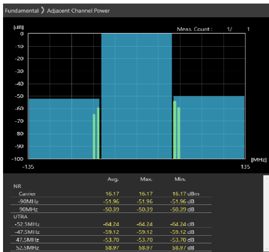
90MHz_30kHz_3655MHz-OFDM QPSK_RB1@244 -51.96,-50.39dB
