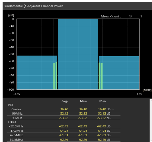
90MHz_30kHz_3655MHz-OFDM QPSK_RB243@0 -52.13,-53.22dB
