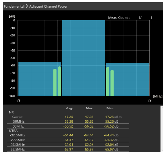
50MHz_30kHz_3675MHz-OFDM QPSK_RB64@32 -55.28,-56.52dB
