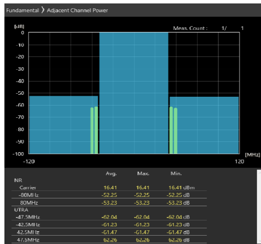
80MHz_30kHz_3660MHz-OFDM QPSK_RB216@0 -52.25,-53.23dB
