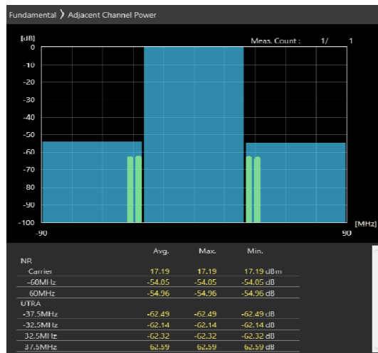
60MHz_30kHz_3670MHz-OFDM QPSK_RB81@40 -54.05,-54.96dB
