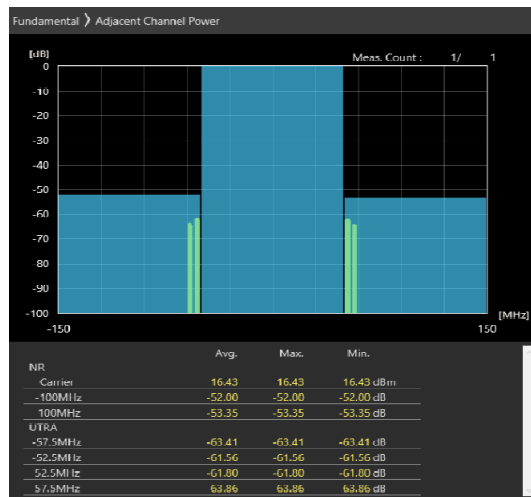
100MHz_30kHz_3650MHz-OFDM QPSK_RB270@0 -52,-53.35dB
