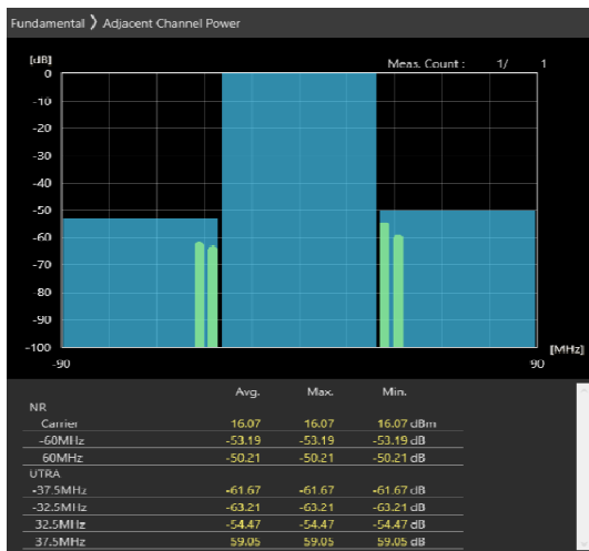
60MHz_30kHz_3670MHz-OFDM QPSK_RB1@161 -53.19,-50.21dB
