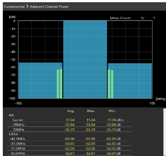
70MHz_30kHz_3665MHz-OFDM QPSK_RB90@45 -53.84,-55.19dB
