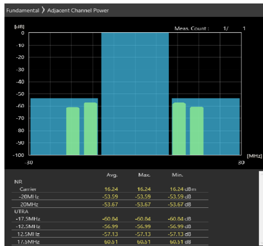
20MHz_30kHz_3690MHz-OFDM QPSK_RB50@0 -53.59,-53.67dB
