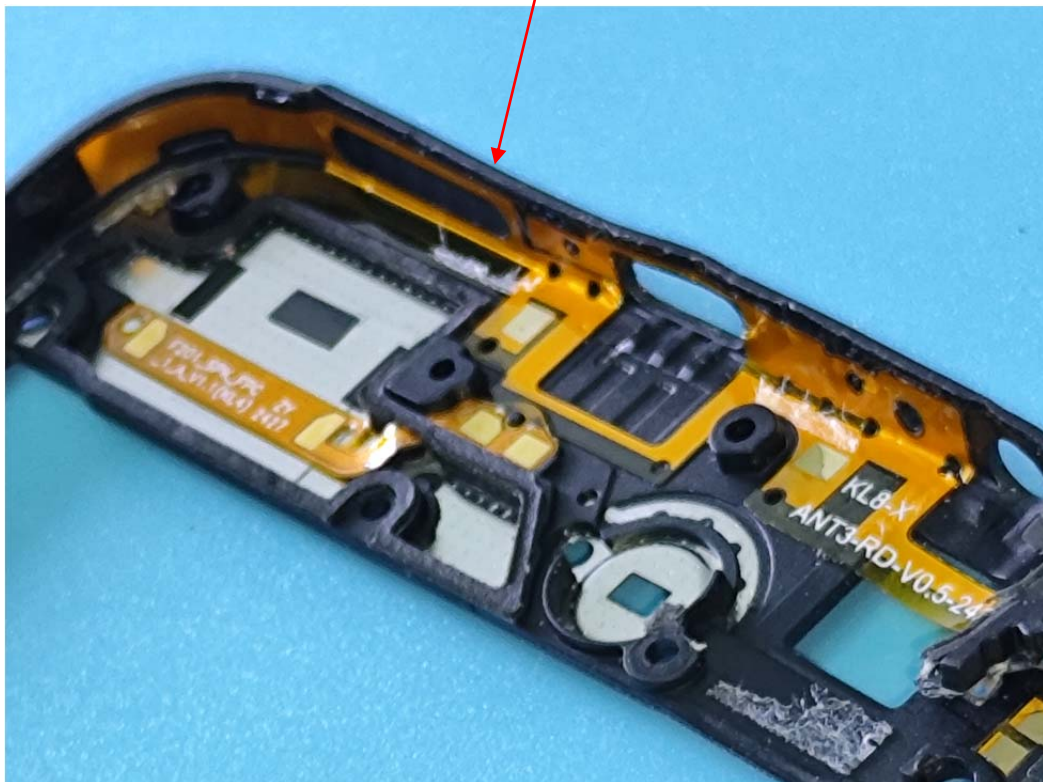
ANT3(LMHB DRX)
