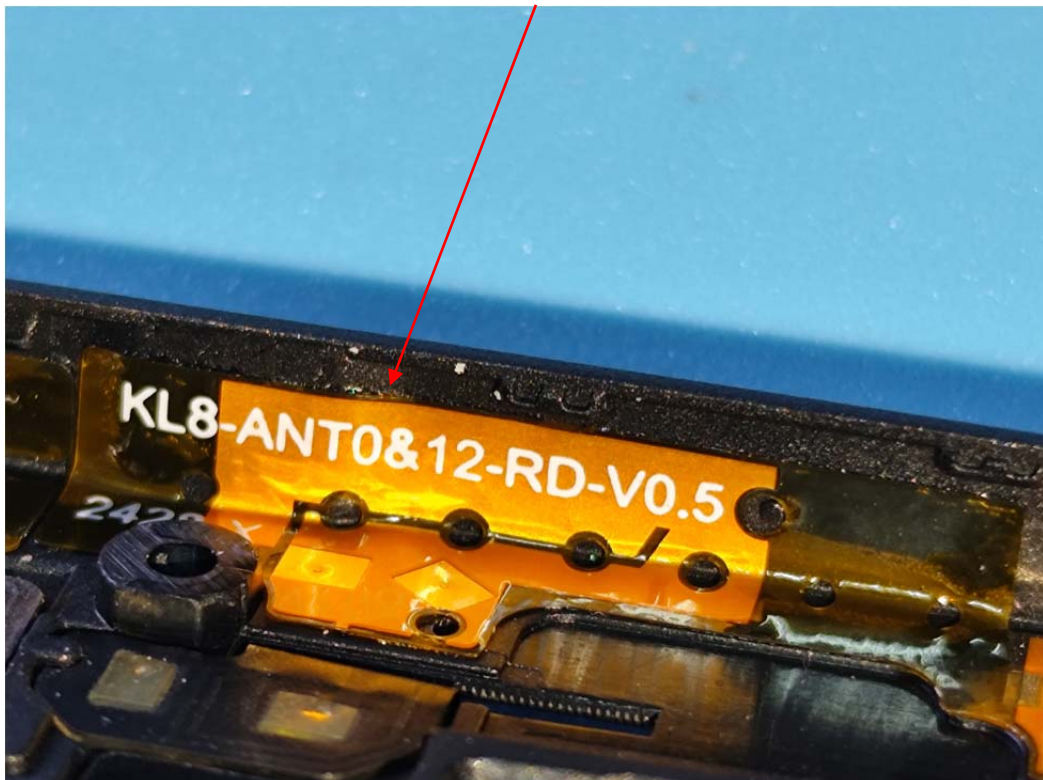
ANT12 (BT/WIFI_2.4G(chain 0)+5G)
