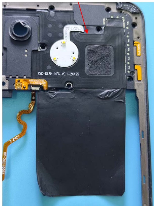
NFC Antenna
