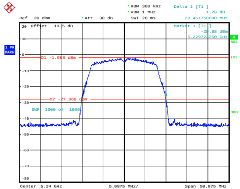
a_5240MHz 20.452MHz
