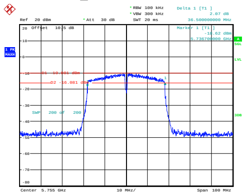
n40_5755MHz 36.500MHz
