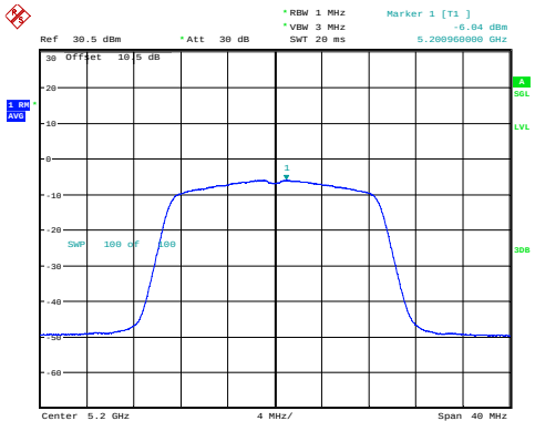
n20_5200MHz -6.04dBm/MHz
