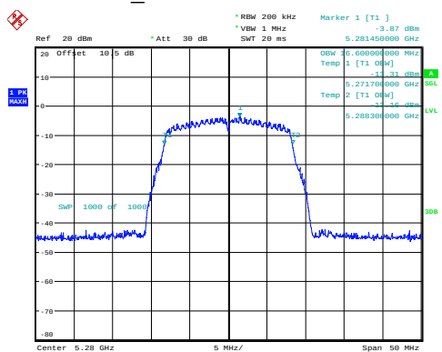
a_5280MHz 16.600MHz
