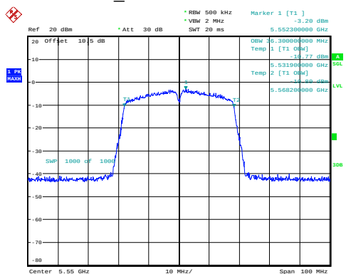
n40_5550MHz 36.300MHz
