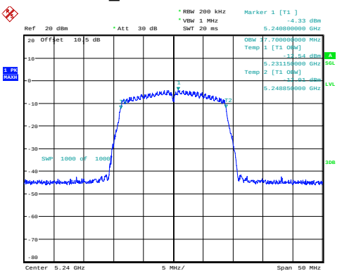
n20_5240MHz 17.700MHz
