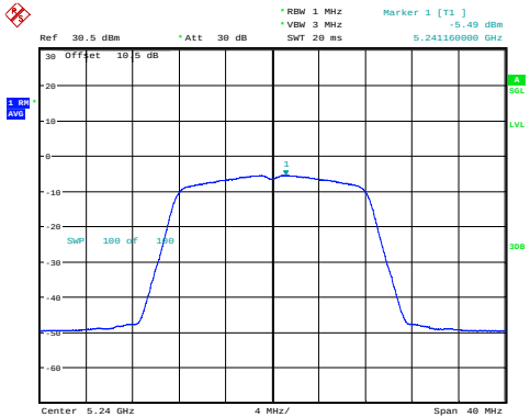
a_5240MHz -5.49dBm/MHz
