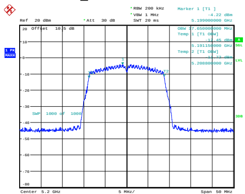
n20_5200MHz 17.650MHz
