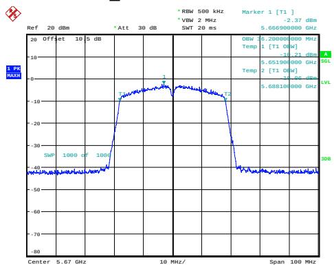
n40_5670MHz 36.200MHz
