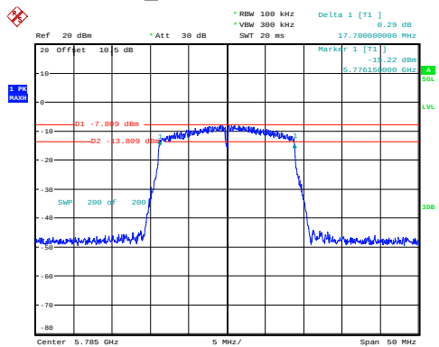
n20_5785MHz 17.700MHz
