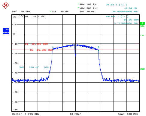
n40_5795MHz 36MHz
