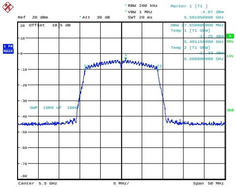
n20_5500MHz 17.650MHz
