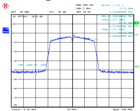
n40_5190MHz 36.200MHz
