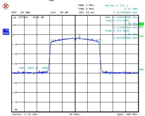
ac80_5210MHz 75.600MHz
