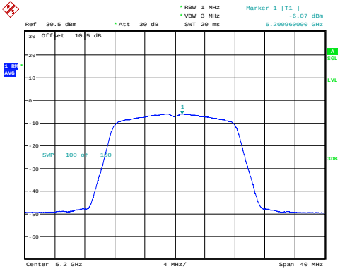
a_5200MHz -6.07dBm/MHz
