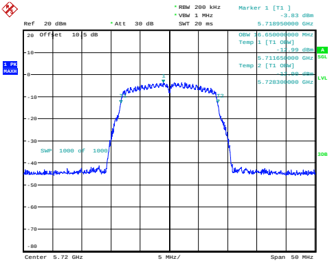
a_5720MHz 16.650MHz
