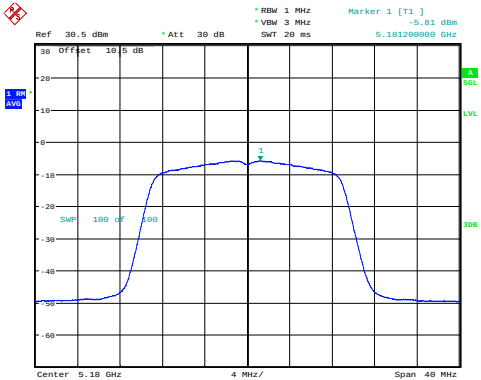
n20_5180MHz -5.81dBm/MHz
