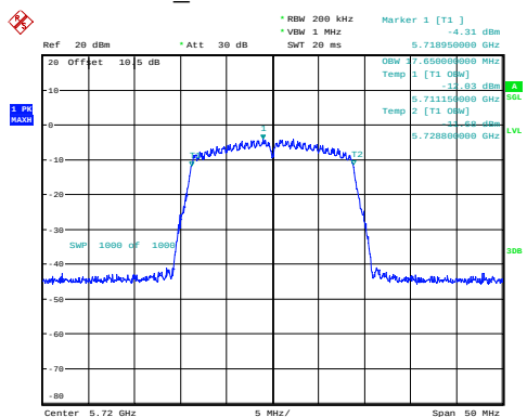
n20_5720MHz 17.650MHz
