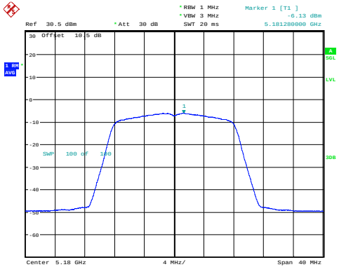
a_5180MHz -6.13dBm/MHz
