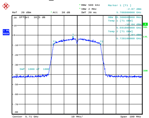
n40_5710MHz 36.300MHz
