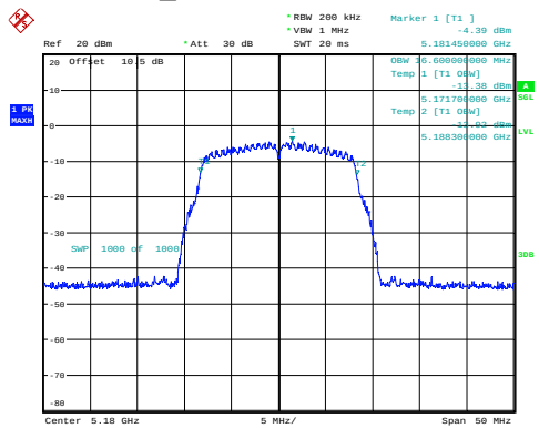
a_5180MHz 16.600MHz
