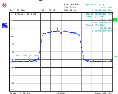
n40_5510MHz 36.400MHz
