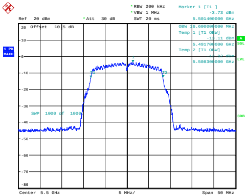
a_5500MHz 16.600MHz
