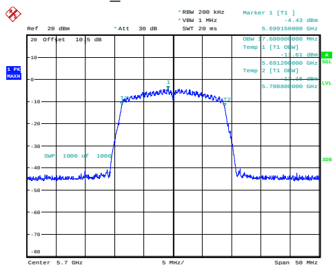
n20_5700MHz 17.600MHz
