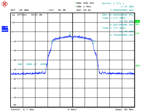
a_5700MHz 16.600MHz
