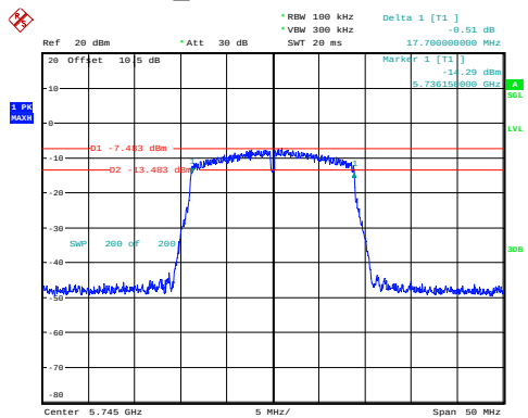
n20_5745MHz 17.700MHz
