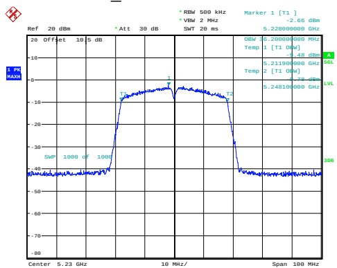
n40_5230MHz 36.200MHz
