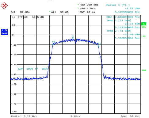
n20_5180MHz 17.650MHz
