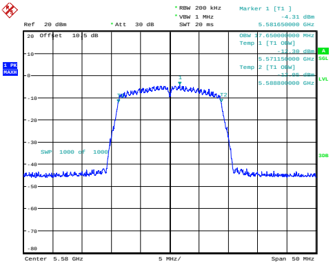
n20_5580MHz 17.650MHz
