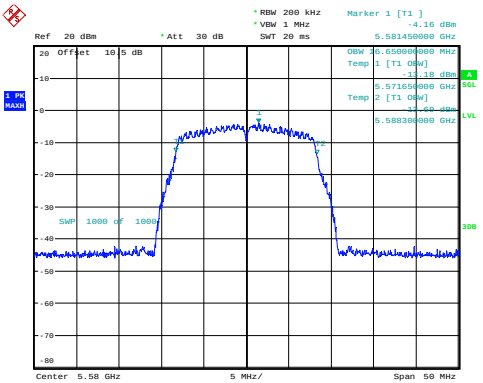
a_5580MHz 16.650MHz
