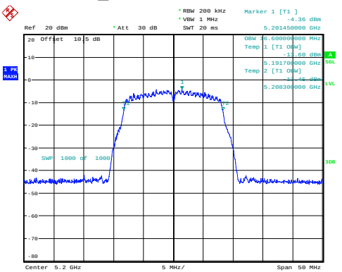
a_5200MHz 16.600MHz
