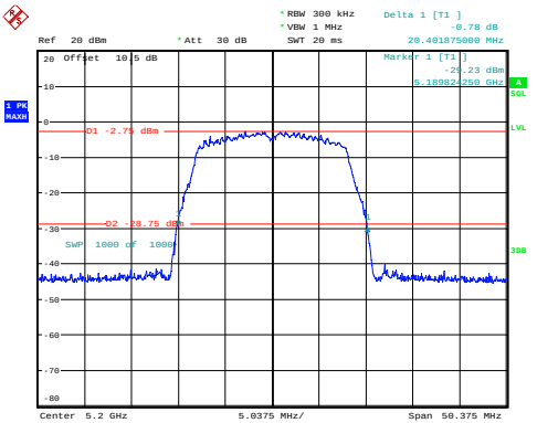
a_5200MHz 20.402MHz
