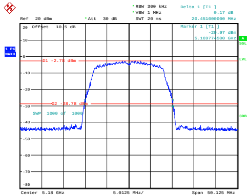
a_5180MHz 20.451MHz
