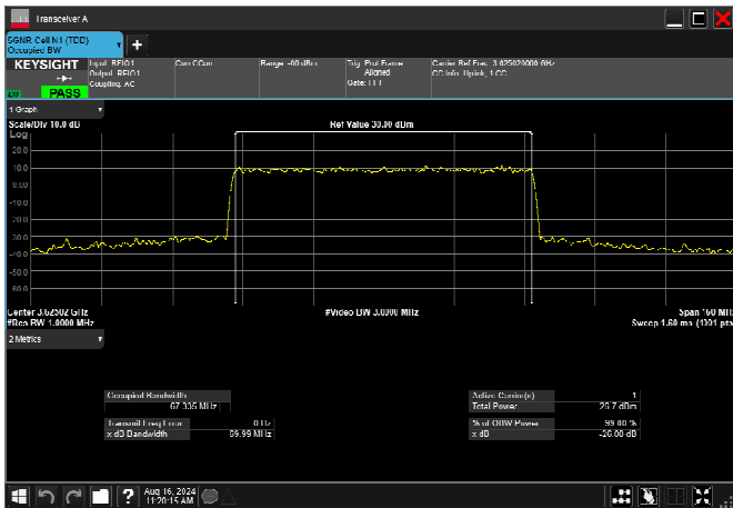
n78_2_80MHz_30kHz_3625MHz_DFT-s-OFDM QPSK_RB216@0 76.855MHz
