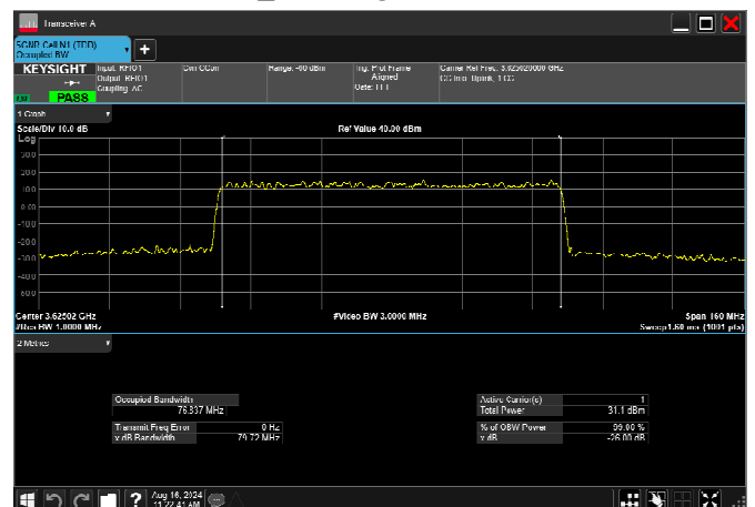
n78_2_80MHz_30kHz_3625MHz_DFT-s-OFDM 16 QAM_RB216@0 76.837MHz
