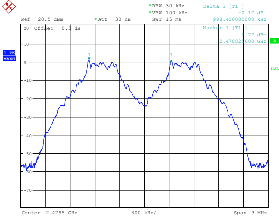
GFSK_High 0.998MHz
