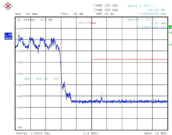
\pi/4 -DQPSK_Hopping_Upper 53.06dB
