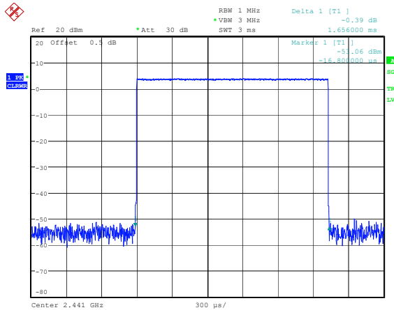
GFSK_Hopping_DH3 1.656ms
