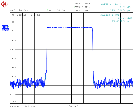
GFSK_Hopping_DH1 0.395ms
