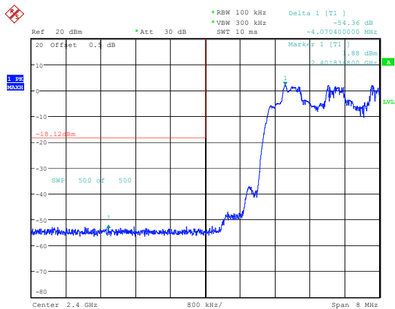
\pi/4 -DQPSK_Hopping_Lower 54.36dB
