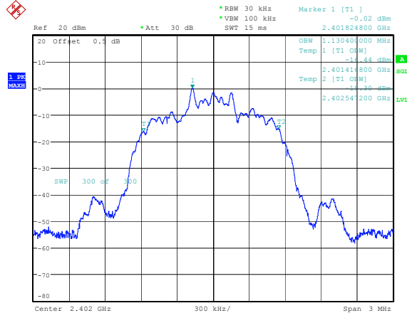
\pi/4 -DQPSK_Low 1.130MHz
