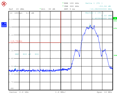
Low 53.06dB
