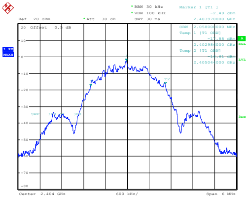
Low 2.058MHz
