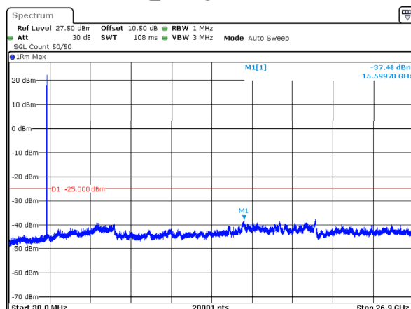
n41_15MHz_30kHz_2503.5MHz_DFT-s-OFDM QPSK_RB1@0 -37.48dBm
