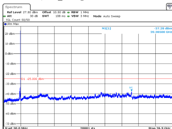
n41_90MHz_30kHz_2592.99MHz_DFT-s-OFDM QPSK_RB1@244 -37.28dBm
