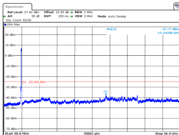
n41_100MHz_30kHz_2640MHz_DFT-s-OFDM QPSK_RB270@0 -37.77dBm
