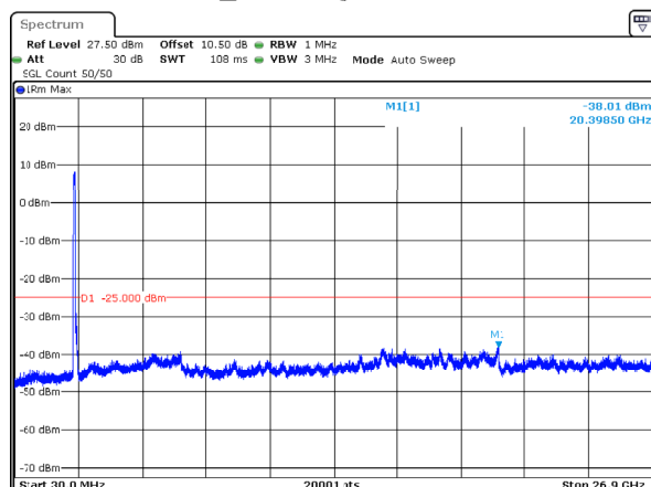
n41_90MHz_30kHz_2541MHz_DFT-s-OFDM QPSK_RB243@0 -38.01dBm
