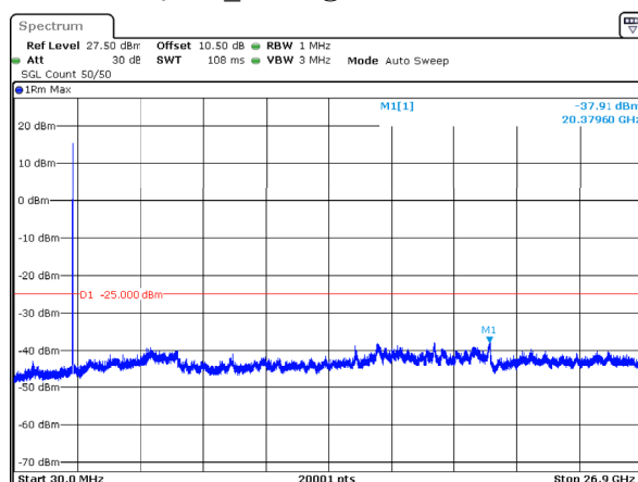
n41_15MHz_30kHz_2503.5MHz_DFT-s-OFDM QPSK_RB36@0 -37.91dBm
