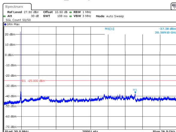
n41_90MHz_30kHz_2592.99MHz_DFT-s-OFDM QPSK_RB1@0 -37.30dBm
