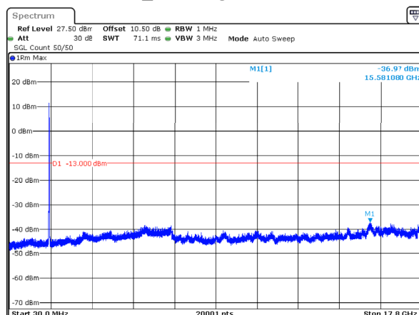
n66_20MHz_15kHz_1720MHz_DFT-s-OFDM QPSK_RB100@0 -36.97dBm
