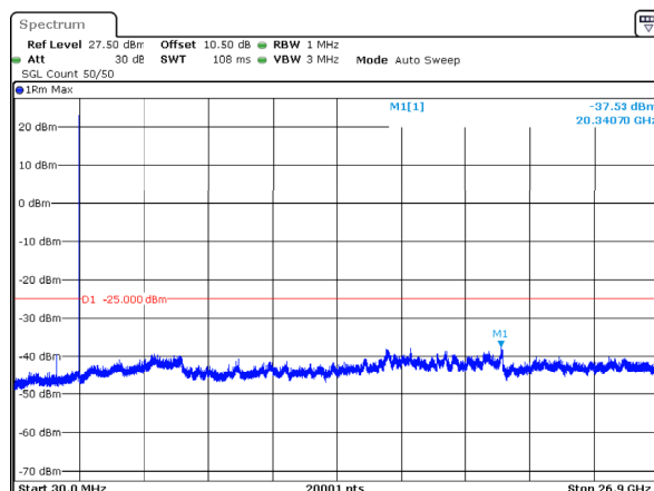
n41_10MHz_30kHz_2685MHz_DFT-s-OFDM QPSK_RB1@23 -37.53dBm
