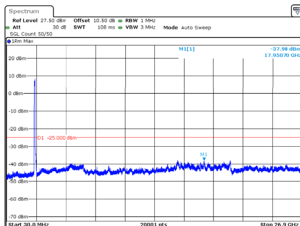
n41_100MHz_30kHz_2546.01MHz_DFT-s-OFDM QPSK_RB270@0 -37.90dBm
