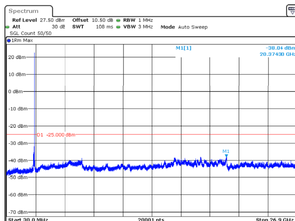
n41_90MHz_30kHz_2541MHz_DFT-s-OFDM QPSK_RB1@244 -38.04dBm
