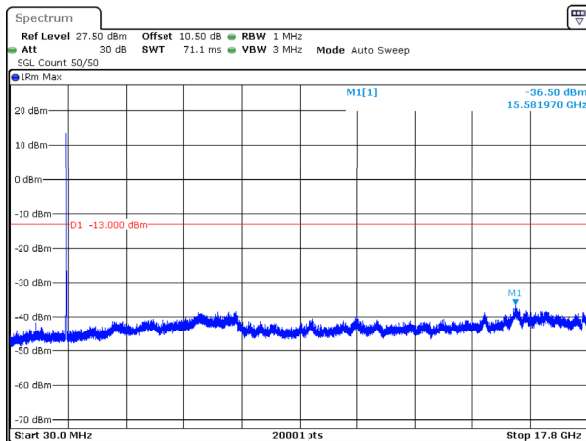
n66_10MHz_15kHz_1745MHz_DFT-s-OFDM QPSK_RB50@0 -36.50dBm
