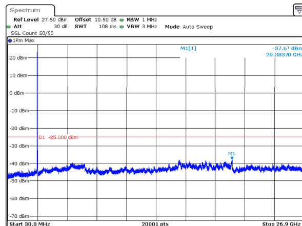
n41_30MHz_30kHz_2674.98MHz_DFT-s-OFDM QPSK_RB1@0 -37.67dBm
