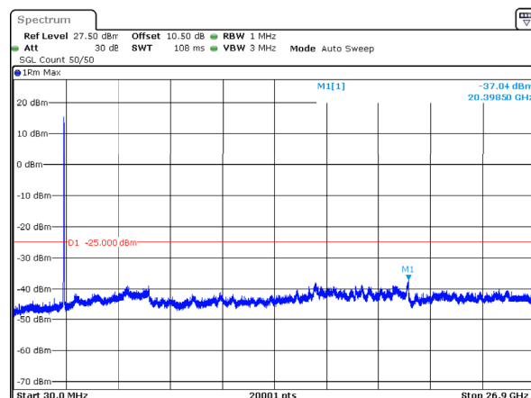
n41_20MHz_30kHz_2592.99MHz_DFT-s-OFDM QPSK_RB50@0 -37.04dBm
