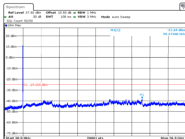
n41_30MHz_30kHz_2674.98MHz_DFT-s-OFDM QPSK_RB75@0 -37.69dBm
