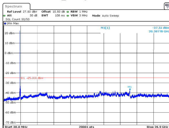
n41_100MHz_30kHz_2640MHz_DFT-s-OFDM QPSK_RB1@0 -37.55dBm
