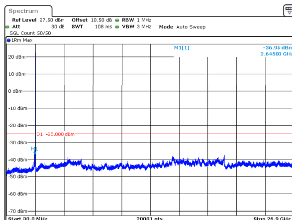
n41_90MHz_30kHz_2644.98MHz_DFT-s-OFDM QPSK_RB1@244 -36.95dBm
