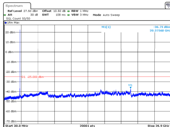
n41_20MHz_30kHz_2506.02MHz_DFT-s-OFDM QPSK_RB1@50 -36.73dBm
