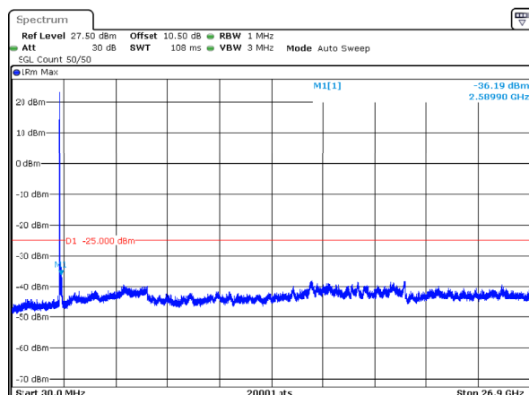
n41_90MHz_30kHz_2541MHz_DFT-s-OFDM QPSK_RB1@0 -36.19dBm
