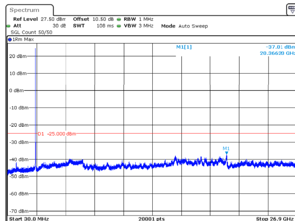
n41_50MHz_30kHz_2592.99MHz_DFT-s-OFDM QPSK_RB1@0 -37.01dBm
