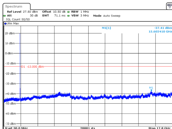
n66_20MHz_15kHz_1720MHz_DFT-s-OFDM QPSK_RB1@0 -37.41dBm
