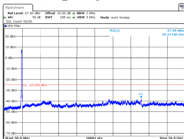
n41_90MHz_30kHz_2592.99MHz_DFT-s-OFDM QPSK_RB243@0 -37.09dBm
