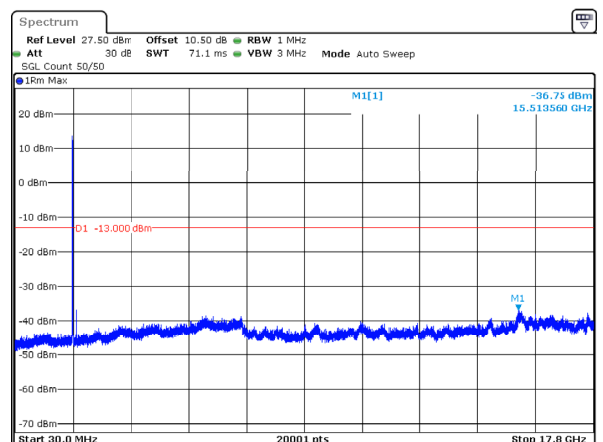
n66_10MHz_15kHz_1775MHz_DFT-s-OFDM QPSK_RB50@0 -36.75dBm
