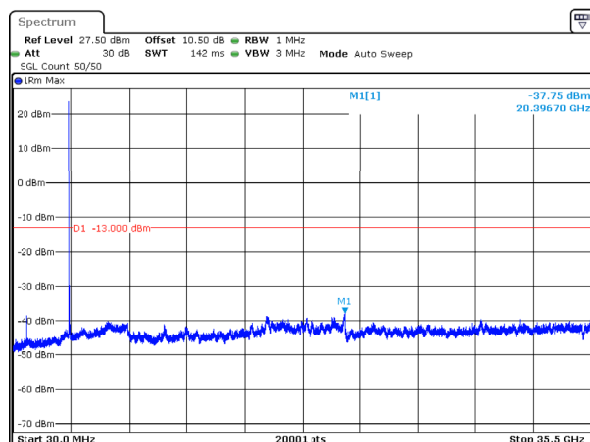
n78_1_50MHz_30kHz_3475MHz_DFT-s-OFDM QPSK_RB1@0 -37.75dBm
