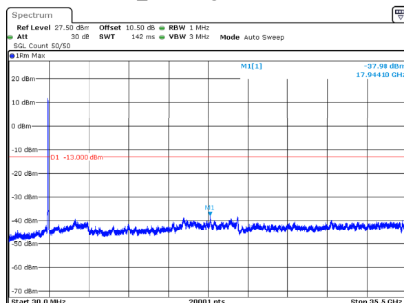
n78_1_50MHz_30kHz_3475MHz_DFT-s-OFDM QPSK_RB128@0 -37.98dBm
