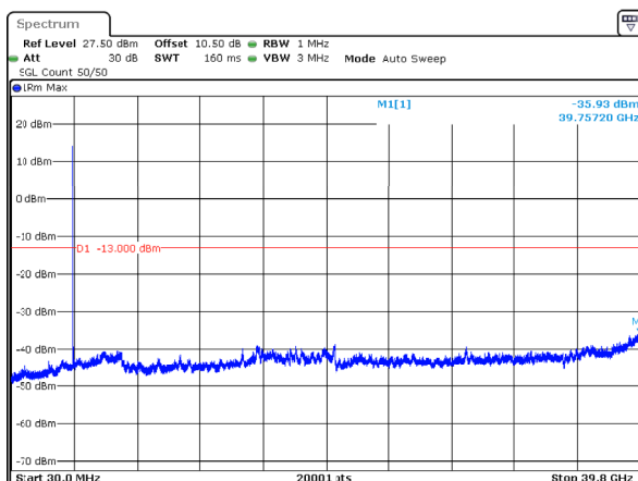
n77_3_60MHz_30kHz_3950MHz_DFT-s-OFDM QPSK_RB1@0 -35.93dBm
