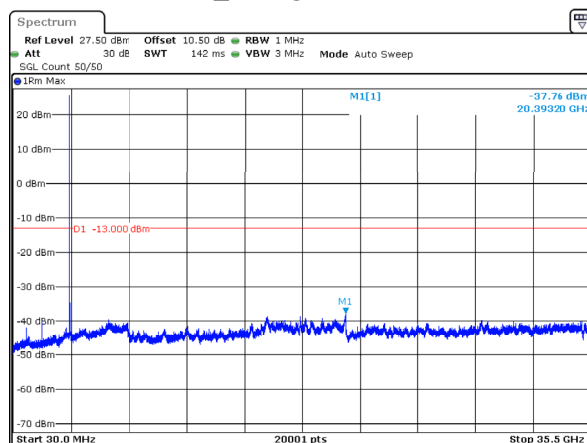
n78_1_30MHz_30kHz_3465MHz_DFT-s-OFDM QPSK_RB1@0 -37.76dBm
