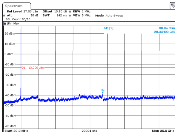
n78_1_30MHz_30kHz_3500MHz_DFT-s-OFDM QPSK_RB1@77 -38.05dBm
