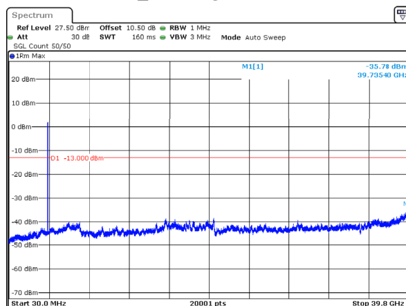
n77_3_50MHz_30kHz_3840MHz_DFT-s-OFDM QPSK_RB128@0 -35.78dBm
