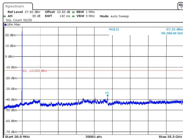
n78_1_20MHz_30kHz_3460MHz_DFT-s-OFDM QPSK_RB1@50 -37.25dBm
