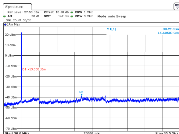
n78_1_40MHz_30kHz_3530MHz_DFT-s-OFDM QPSK_RB1@0 -38.22dBm
