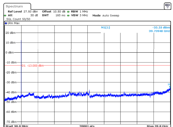
n77_3_60MHz_30kHz_3950MHz_DFT-s-OFDM QPSK_RB1@161 -35.53dBm
