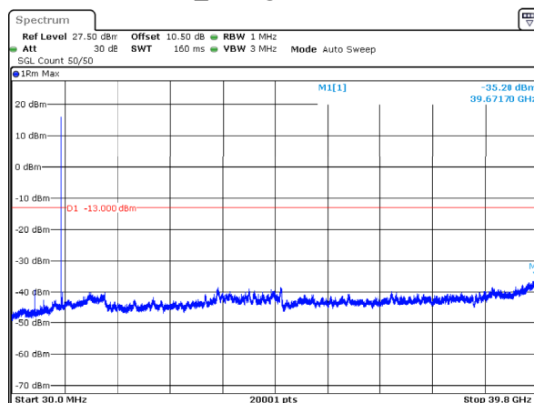
n77_3_100MHz_30kHz_3750MHz_DFT-s-OFDM QPSK_RB1@0 -35.20dBm
