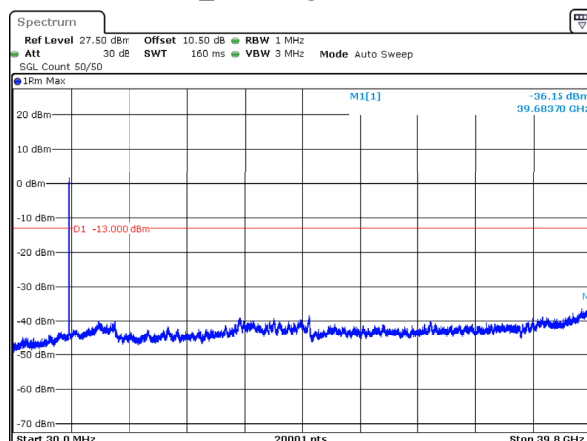
n77_3_70MHz_30kHz_3840MHz_DFT-s-OFDM QPSK_RB180@0 -36.15dBm
