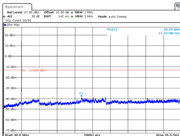
n78_1_30MHz_30kHz_3535MHz_DFT-s-OFDM QPSK_RB75@0 -38.39dBm
