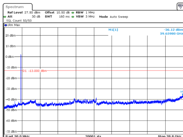
n77_3_70MHz_30kHz_3735MHz_DFT-s-OFDM QPSK_RB180@0 -36.12dBm
