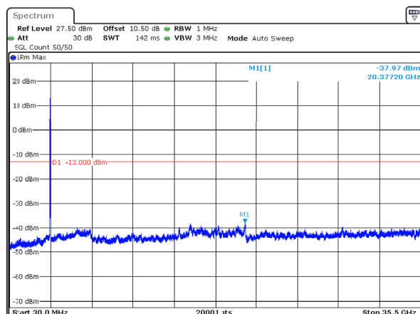
n78_1_40MHz_30kHz_3530MHz_DFT-s-OFDM QPSK_RB100@0 -37.97dBm
