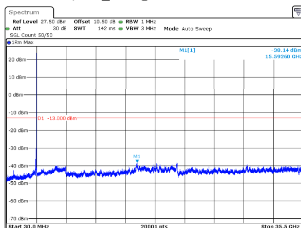
n78_1_60MHz_30kHz_3500MHz_DFT-s-OFDM QPSK_RB1@161 -38.14dBm
