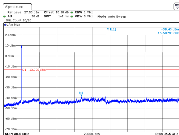
n78_1_70MHz_30kHz_3485MHz_DFT-s-OFDM QPSK_RB180@0 -38.45dBm
