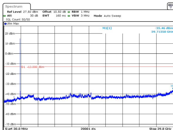
n77_3_80MHz_30kHz_3840MHz_DFT-s-OFDM QPSK_RB1@0 -35.46dBm
