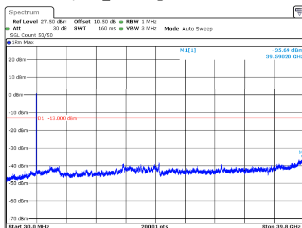
n77_3_80MHz_30kHz_3940MHz_DFT-s-OFDM QPSK_RB216@0 -35.69dBm
