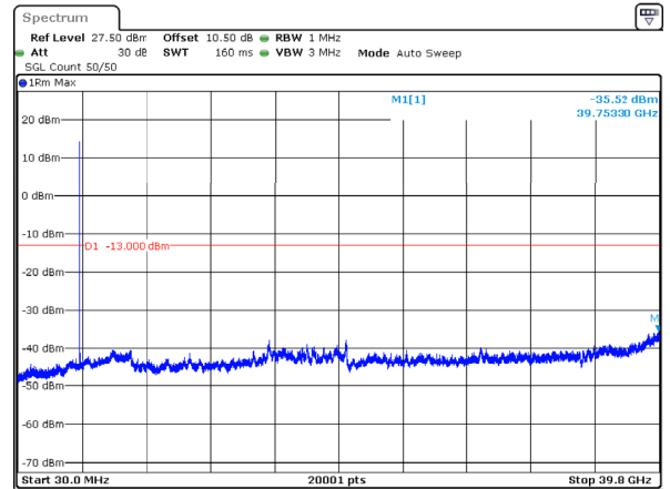
n77_3_60MHz_30kHz_3840MHz_DFT-s-OFDM QPSK_RB1@0 -35.52dBm
