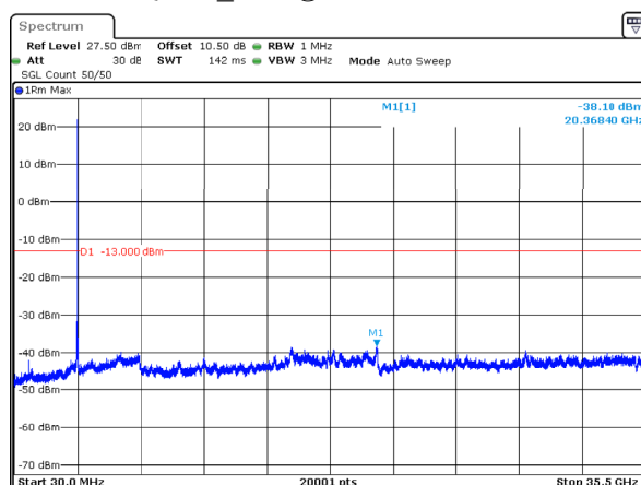
n78_1_70MHz_30kHz_3515MHz_DFT-s-OFDM QPSK_RB1@188 -38.10dBm
