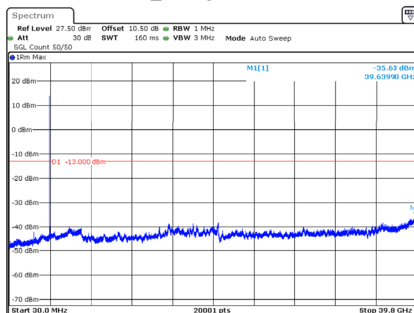
n77_3_80MHz_30kHz_3940MHz_DFT-s-OFDM QPSK_RB1@0 -35.63dBm
