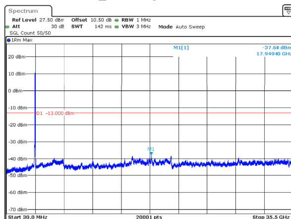
n78_1_70MHz_30kHz_3515MHz_DFT-s-OFDM QPSK_RB180@0 -37.60dBm
