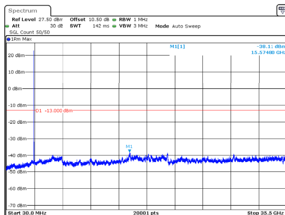
n78_1_40MHz_30kHz_3470MHz_DFT-s-OFDM QPSK_RB1@0 -38.11dBm
