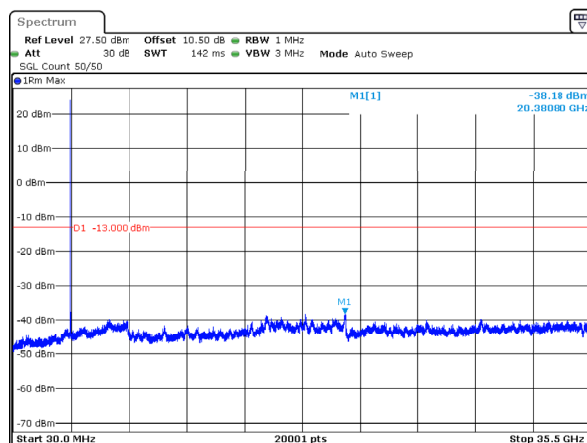
n78_1_15MHz_30kHz_3500MHz_DFT-s-OFDM QPSK_RB1@37 -38.18dBm
