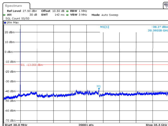
n78_1_20MHz_30kHz_3500MHz_DFT-s-OFDM QPSK_RB1@0 -38.27dBm
