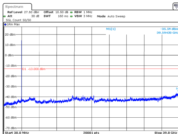
n77_3_90MHz_30kHz_3935MHz_DFT-s-OFDM QPSK_RB1@244 -35.59dBm
