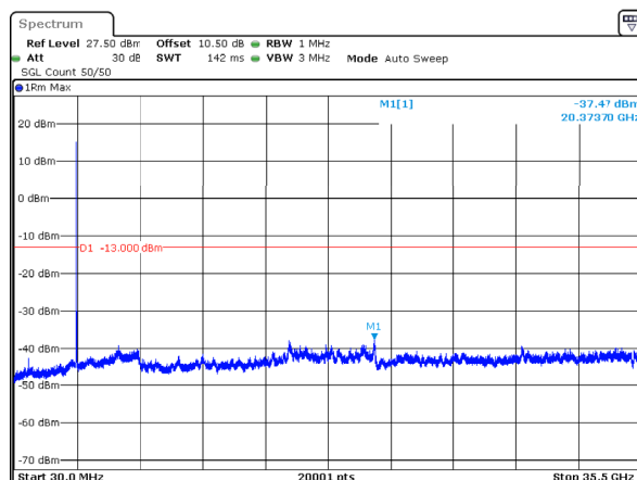
n78_1_20MHz_30kHz_3500MHz_DFT-s-OFDM QPSK_RB50@0 -37.47dBm
