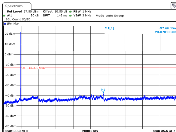
n78_1_15MHz_30kHz_3457.5MHz_DFT-s-OFDM QPSK_RB1@0 -37.60dBm
