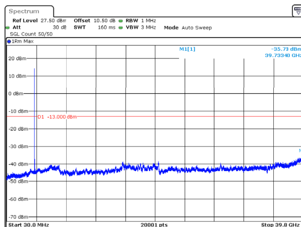
n77_3_50MHz_30kHz_3725MHz_DFT-s-OFDM QPSK_RB1@0 -35.73dBm
