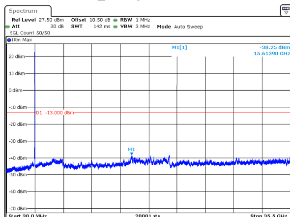
n78_1_40MHz_30kHz_3530MHz_DFT-s-OFDM QPSK_RB1@105 -38.25dBm
