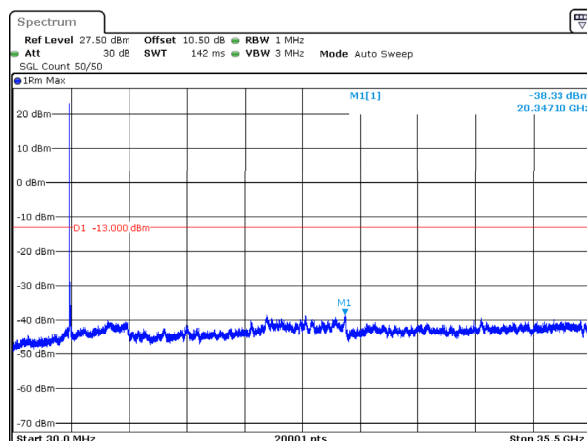
n78_1_60MHz_30kHz_3480MHz_DFT-s-OFDM QPSK_RB1@0 -38.33dBm
