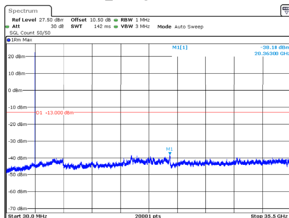
n78_1_15MHz_30kHz_3542.5MHz_DFT-s-OFDM QPSK_RB1@0 -38.18dBm
