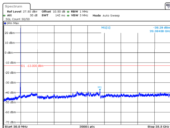
n78_1_70MHz_30kHz_3485MHz_DFT-s-OFDM QPSK_RB1@188 -38.20dBm
