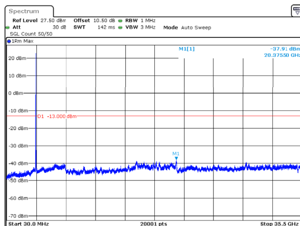
n78_1_70MHz_30kHz_3500MHz_DFT-s-OFDM QPSK_RB1@0 -37.91dBm
