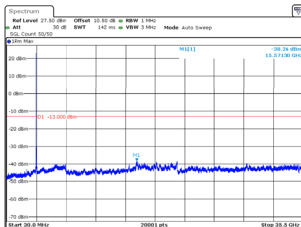
n78_1_60MHz_30kHz_3520MHz_DFT-s-OFDM QPSK_RB1@0 -38.26dBm
