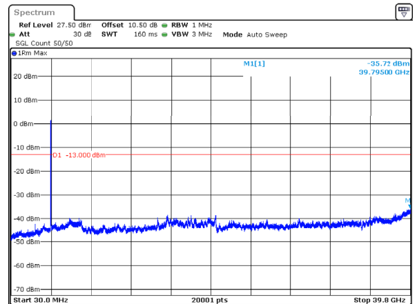
n77_3_60MHz_30kHz_3950MHz_DFT-s-OFDM QPSK_RB162@0 -35.72dBm
