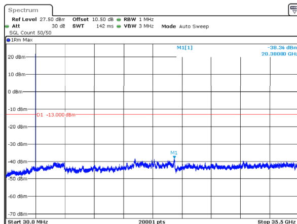
n78_1_10MHz_30kHz_3545MHz_DFT-s-OFDM QPSK_RB1@23 -38.36dBm
