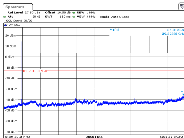
n77_3_80MHz_30kHz_3840MHz_DFT-s-OFDM QPSK_RB1@216 -36.01dBm
