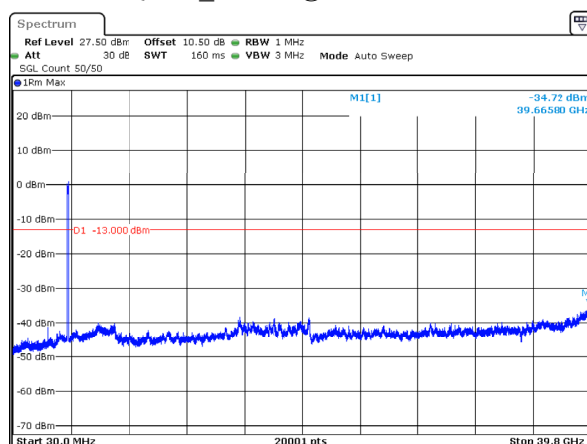
n77_3_100MHz_30kHz_3750MHz_DFT-s-OFDM QPSK_RB270@0 -34.72dBm
