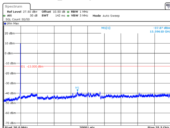
n78_1_60MHz_30kHz_3500MHz_DFT-s-OFDM QPSK_RB162@0 -37.87dBm
