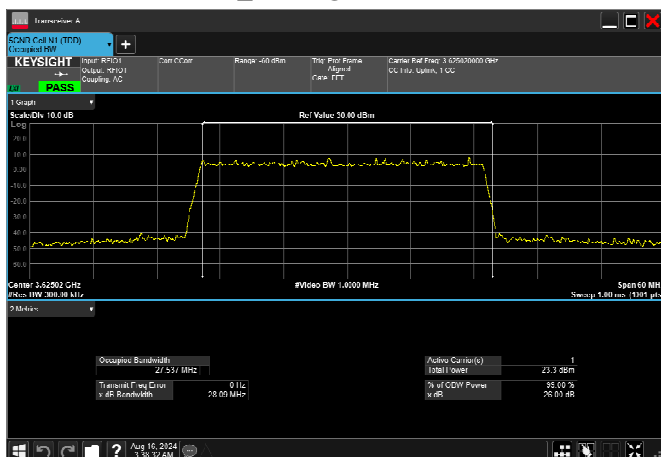
n77_2_30MHz_30kHz_3625MHz_DFT-s-OFDM QPSK_RB75@0 27.537MHz
