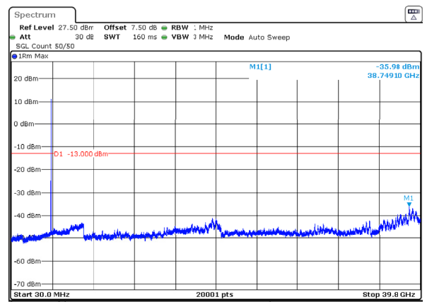
n77_3_15MHz_30kHz_3840MHz_DFT-s-OFDM QPSK_RB1@0 -35.98dBm
