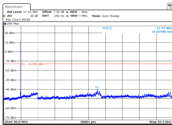
n77_1_90MHz_30kHz_3495MHz_DFT-s-OFDM QPSK_RB1@0 -41.25dBm
