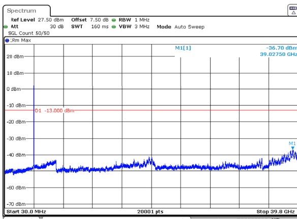
n77_3_30MHz_30kHz_3965MHz_DFT-s-OFDM QPSK_RB75@0 -36.70dBm
