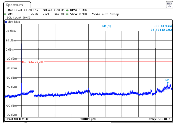
n77_3_10MHz_30kHz_3975MHz_DFT-s-OFDM QPSK_RB24@0 -36.48dBm
