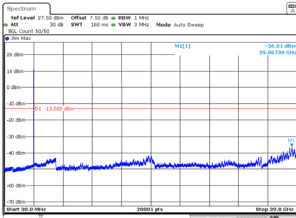
n77_3_30MHz_30kHz_3965MHz_DFT-s-OFDM QPSK_RB1@0 -36.01dBm
