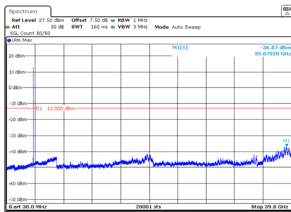
n77_3_50MHz_30kHz_3725MHz_DFT-s-OFDM QPSK_RB1@132 -36.87dBm
