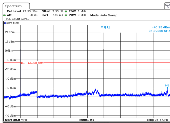
n77_1_80MHz_30kHz_3510MHz_DFT-s-OFDM QPSK_RB1@0 -40.93dBm
