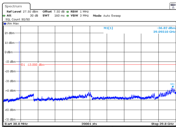
n77_3_40MHz_30kHz_3720MHz_DFT-s-OFDM QPSK_RB1@0 -36.82dBm
