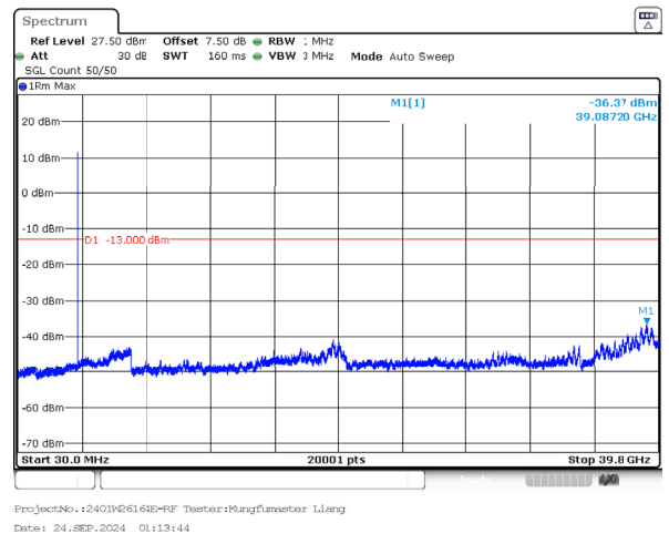
n77_3_10MHz_30kHz_3705MHz_DFT-s-OFDM QPSK_RB1@0 -36.37dBm
