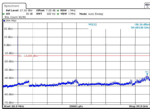
n77_3_10MHz_30kHz_3975MHz_DFT-s-OFDM QPSK_RB1@0 -36.16dBm
