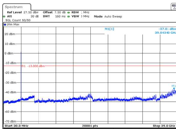
n77_3_40MHz_30kHz_3960MHz_DFT-s-OFDM QPSK_RB100@0 -37.01dBm
