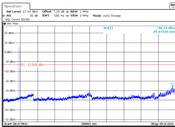
n77_3_15MHz_30kHz_3707.5MHz_DFT-s-OFDM QPSK_RB36@0 -36.25dBm
