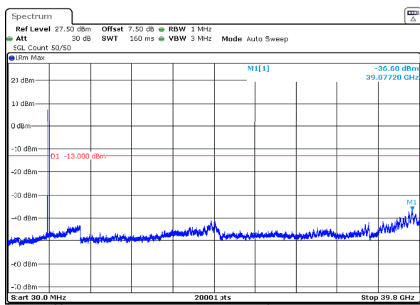
n77_3_10MHz_30kHz_3840MHz_DFT-s-OFDM QPSK_RB24@0 -36.60dBm
