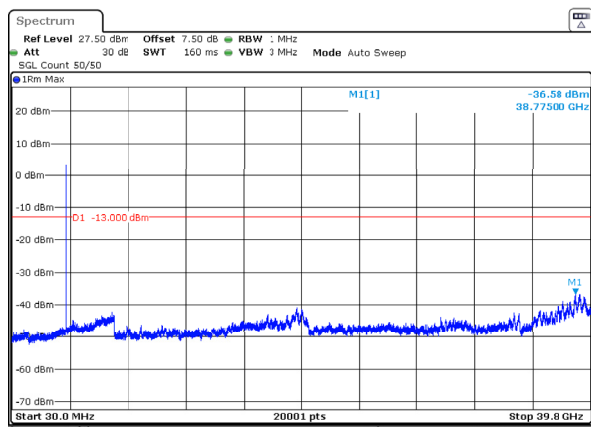
n77_3_20MHz_30kHz_3710MHz_DFT-s-OFDM QPSK_RB50@0 -36.58dBm
