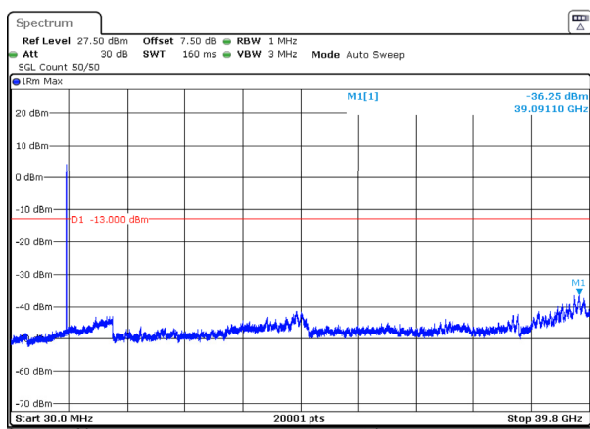
n77_3_20MHz_30kHz_3840MHz_DFT-s-OFDM QPSK_RB50@0 -36.25dBm
