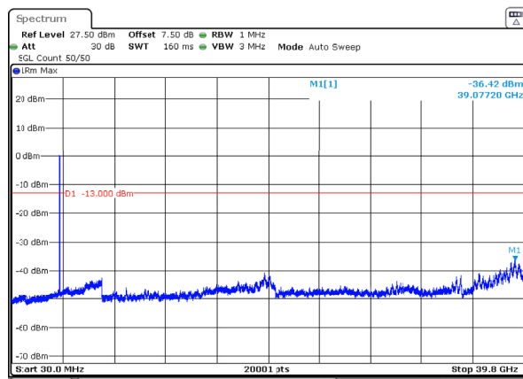
n77_3_50MHz_30kHz_3725MHz_DFT-s-OFDM QPSK_RB128@0 -36.42dBm
