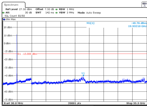
n77_1_90MHz_30kHz_3500MHz_DFT-s-OFDM QPSK_RB1@0 -40.76dBm
