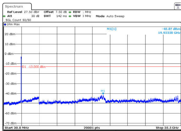
n77_1_90MHz_30kHz_3495MHz_DFT-s-OFDM QPSK_RB243@0 -40.82dBm
