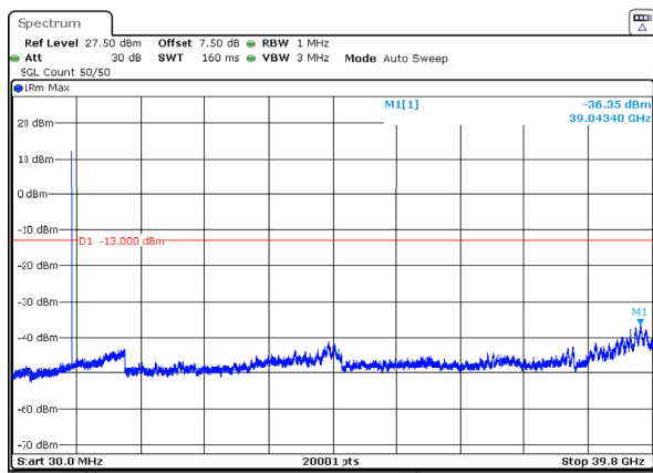
n77_3_20MHz_30kHz_3710MHz_DFT-s-OFDM QPSK_RB1@50 -36.35dBm
