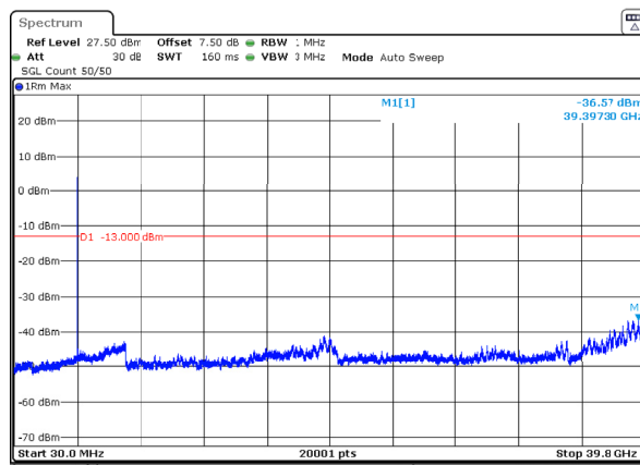
n77_3_20MHz_30kHz_3970MHz_DFT-s-OFDM QPSK_RB50@0 -36.57dBm
