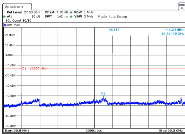
n77_1_80MHz_30kHz_3490MHz_DFT-s-OFDM QPSK_RB1@0 -41.24dBm
