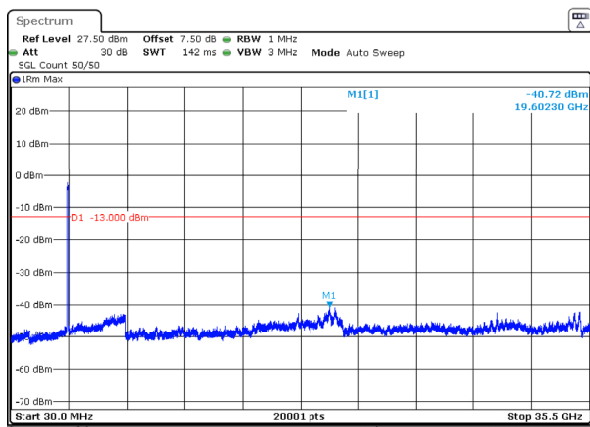
n77_1_90MHz_30kHz_3500MHz_DFT-s-OFDM QPSK_RB243@0 -40.72dBm
