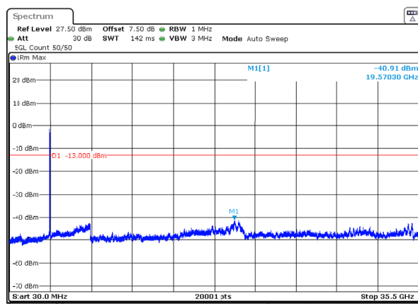
n77_1_80MHz_30kHz_3510MHz_DFT-s-OFDM QPSK_RB216@0 -40.91dBm
