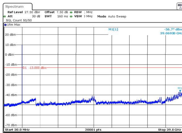
n77_3_40MHz_30kHz_3960MHz_DFT-s-OFDM QPSK_RB1@105 -36.77dBm
