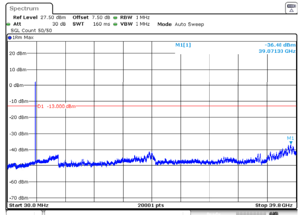
n77_3_30MHz_30kHz_3840MHz_DFT-s-OFDM QPSK_RB75@0 -36.48dBm
