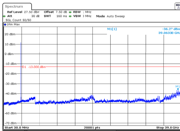
n77_3_40MHz_30kHz_3840MHz_DFT-s-OFDM QPSK_RB1@0 -36.27dBm
