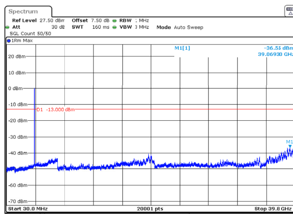
n77_3_50MHz_30kHz_3840MHz_DFT-s-OFDM QPSK_RB128@0 -36.55dBm
