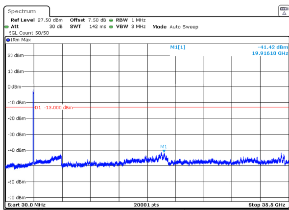
n77_1_80MHz_30kHz_3490MHz_DFT-s-OFDM QPSK_RB216@0 -41.42dBm
