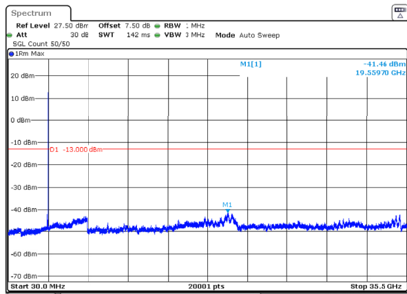
n77_1_90MHz_30kHz_3500MHz_DFT-s-OFDM QPSK_RB1@244 -41.46dBm
