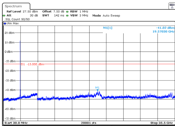
n77_1_70MHz_30kHz_3515MHz_DFT-s-OFDM QPSK_RB1@0 -41.02dBm
