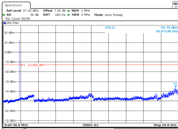
n77_3_15MHz_30kHz_3707.5MHz_DFT-s-OFDM QPSK_RB1@0 -35.70dBm
