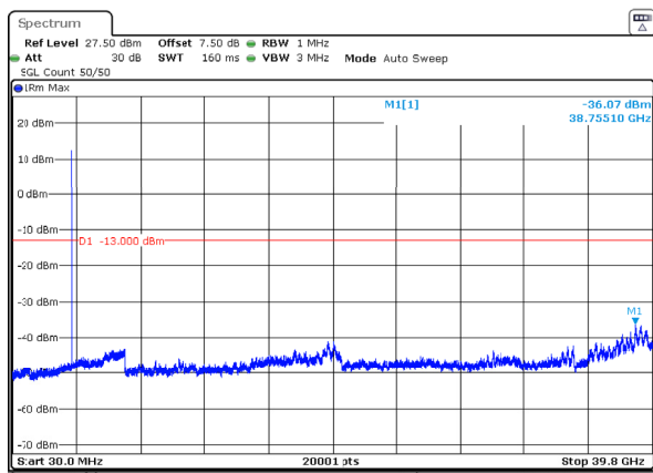
n77_3_10MHz_30kHz_3705MHz_DFT-s-OFDM QPSK_RB1@23 -36.07dBm
