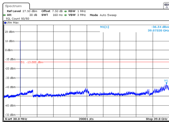
n77_3_40MHz_30kHz_3960MHz_DFT-s-OFDM QPSK_RB1@0 -36.54dBm
