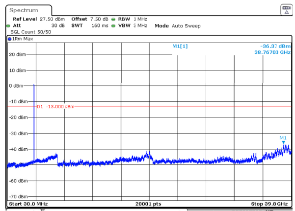
n77_3_40MHz_30kHz_3720MHz_DFT-s-OFDM QPSK_RB100@0 -36.37dBm
