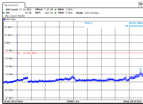
n77_3_20MHz_30kHz_3970MHz_DFT-s-OFDM QPSK_RB1@50 -36.81dBm
