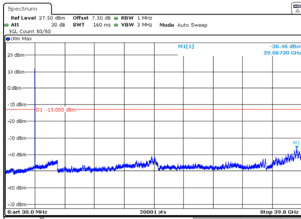
n77_3_10MHz_30kHz_3975MHz_DFT-s-OFDM QPSK_RB1@23 -36.46dBm
