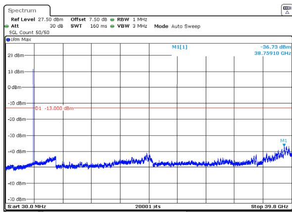
n77_3_10MHz_30kHz_3840MHz_DFT-s-OFDM QPSK_RB1@0 -36.73dBm
