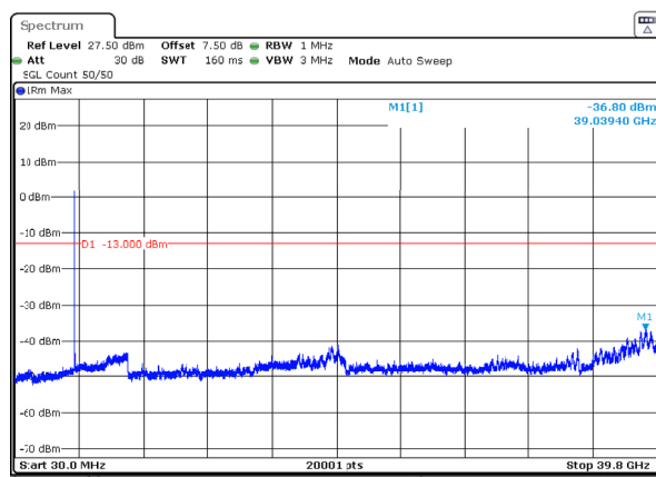
n77_3_30MHz_30kHz_3715MHz_DFT-s-OFDM QPSK_RB75@0 -36.80dBm
