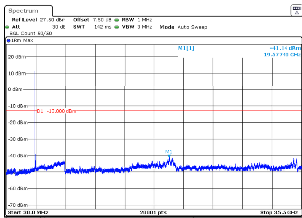
n77_1_90MHz_30kHz_3505MHz_DFT-s-OFDM QPSK_RB1@0 -41.14dBm
