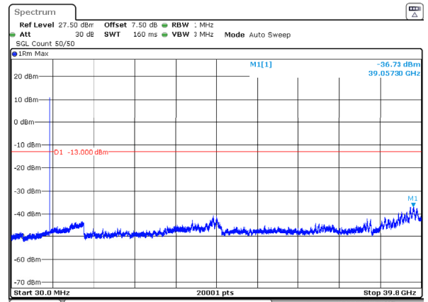
n77_3_15MHz_30kHz_3707.5MHz_DFT-s-OFDM QPSK_RB1@37 -36.73dBm
