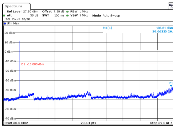
n77_3_40MHz_30kHz_3720MHz_DFT-s-OFDM QPSK_RB1@105 -36.64dBm
