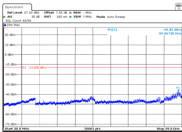
n77_3_20MHz_30kHz_3970MHz_DFT-s-OFDM QPSK_RB1@0 -36.85dBm
