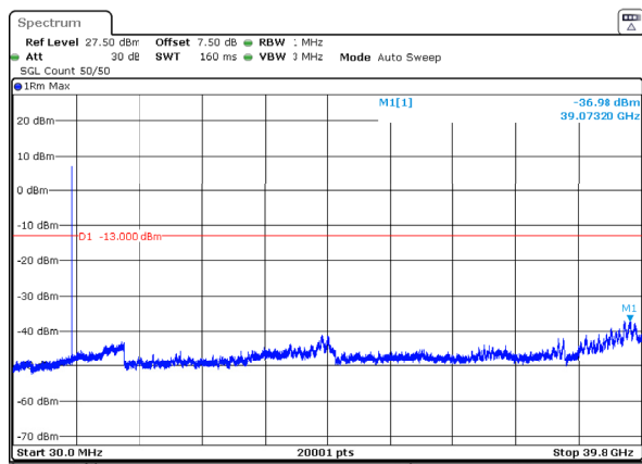
n77_3_10MHz_30kHz_3705MHz_DFT-s-OFDM QPSK_RB24@0 -36.98dBm
