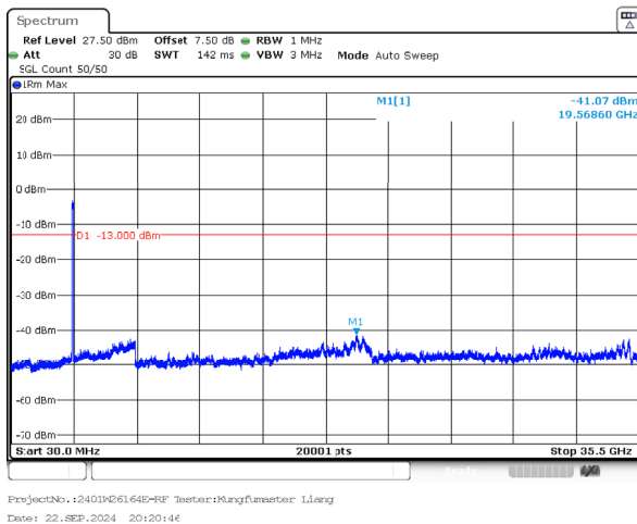
n77_1_100MHz_30kHz_3500MHz_DFT-s-OFDM QPSK_RB270@0 -41.07dBm
