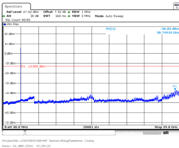
n77_3_15MHz_30kHz_3972.5MHz_DFT-s-OFDM QPSK_RB36@0 -36.85dBm
