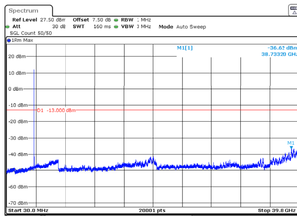
n77_3_50MHz_30kHz_3725MHz_DFT-s-OFDM QPSK_RB1@0 -36.62dBm
