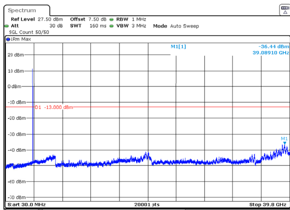
n77_3_20MHz_30kHz_3840MHz_DFT-s-OFDM QPSK_RB1@0 -36.44dBm
