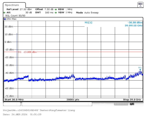
n77_3_20MHz_30kHz_3710MHz_DFT-s-OFDM QPSK_RB1@0 -36.88dBm
