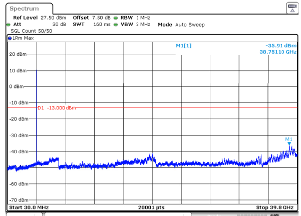
n77_3_30MHz_30kHz_3965MHz_DFT-s-OFDM QPSK_RB1@77 -35.91dBm
