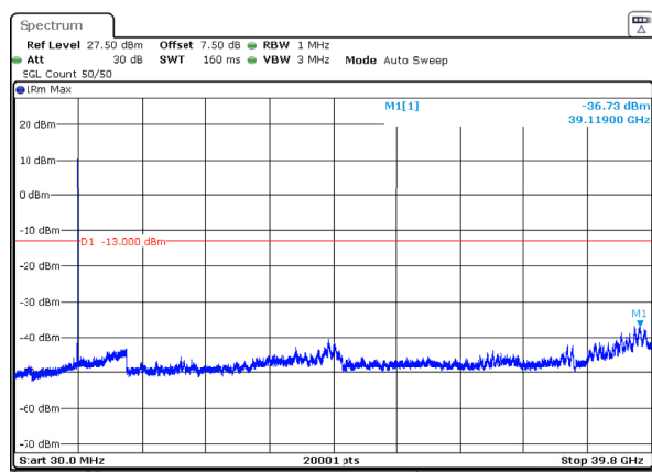
n77_3_50MHz_30kHz_3955MHz_DFT-s-OFDM QPSK_RB1@132 -36.73dBm
