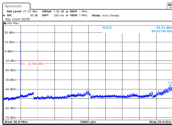
n77_3_60MHz_30kHz_3950MHz_DFT-s-OFDM QPSK_RB1@161 -36.54dBm
