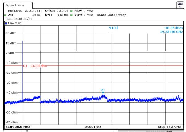
n78_1_20MHz_30kHz_3460MHz_DFT-s-OFDM QPSK_RB1@50 -40.92dBm
