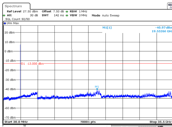
n78_1_10MHz_30kHz_3500MHz_DFT-s-OFDM QPSK_RB24@0 -40.97dBm
