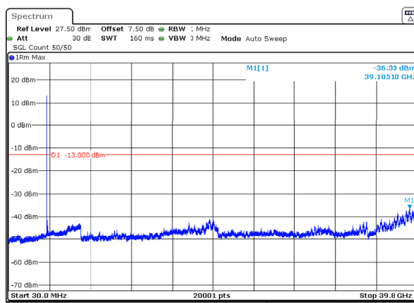
n77_3_80MHz_30kHz_3740MHz_DFT-s-OFDM QPSK_RB1@0 -36.33dBm
