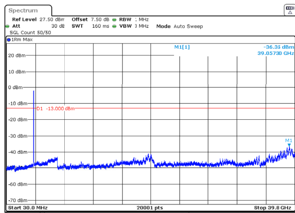
n77_3_80MHz_30kHz_3740MHz_DFT-s-OFDM QPSK_RB216@0 -36.35dBm
