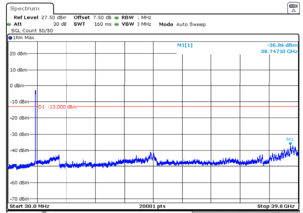
n77_3_100MHz_30kHz_3750MHz_DFT-s-OFDM QPSK_RB270@0 -36.86dBm
