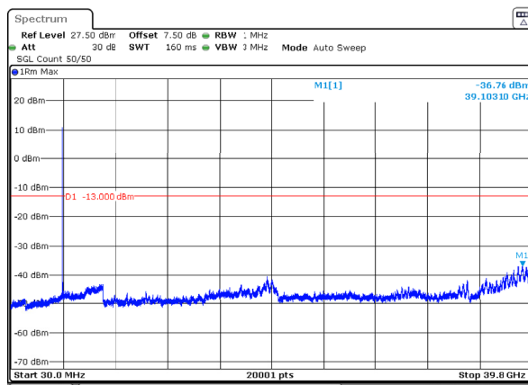
n77_3_70MHz_30kHz_3945MHz_DFT-s-OFDM QPSK_RB1@0 -36.76dBm
