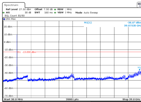
n77_3_50MHz_30kHz_3955MHz_DFT-s-OFDM QPSK_RB1@0 -36.67dBm
