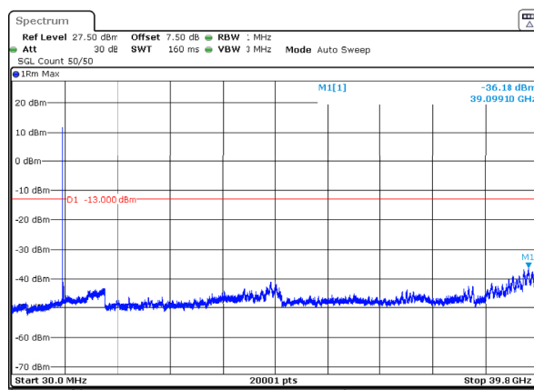
n77_3_90MHz_30kHz_3840MHz_DFT-s-OFDM QPSK_RB1@0 -36.18dBm
