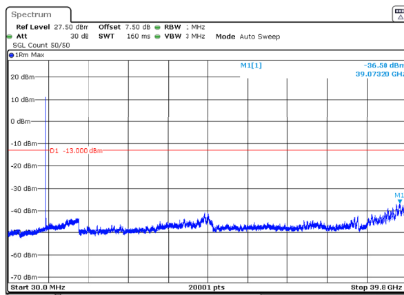
n77_3_70MHz_30kHz_3735MHz_DFT-s-OFDM QPSK_RB1@0 -36.50dBm
