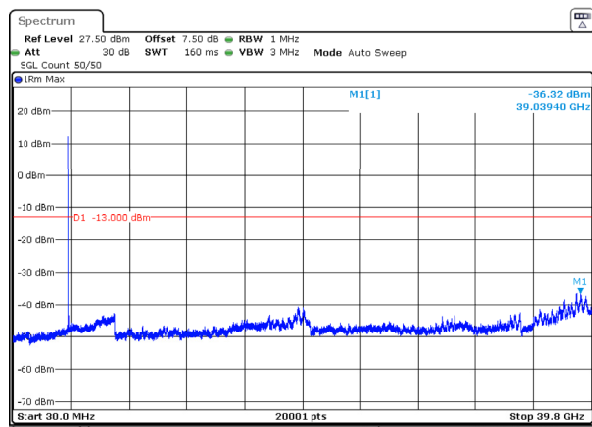
n77_3_50MHz_30kHz_3840MHz_DFT-s-OFDM QPSK_RB1@0 -36.32dBm
