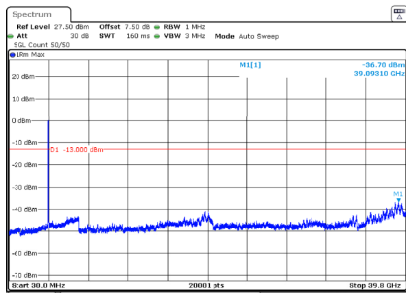
n77_3_50MHz_30kHz_3955MHz_DFT-s-OFDM QPSK_RB128@0 -36.70dBm
