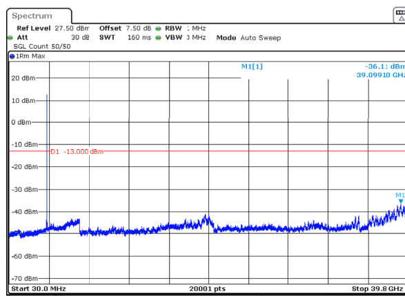
n77_3_60MHz_30kHz_3730MHz_DFT-s-OFDM QPSK_RB1@161 -36.11dBm
