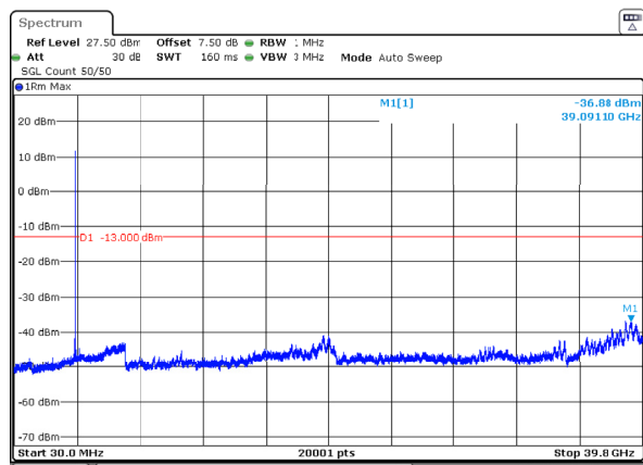
n77_3_80MHz_30kHz_3840MHz_DFT-s-OFDM QPSK_RB1@216 -36.88dBm
