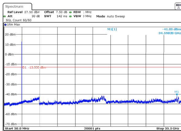
n78_1_15MHz_30kHz_3500MHz_DFT-s-OFDM QPSK_RB1@37 -41.03dBm
