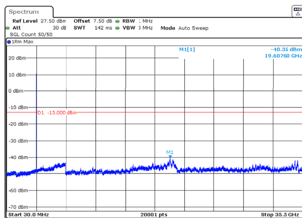
n78_1_15MHz_30kHz_3542.5MHz_DFT-s-OFDM QPSK_RB1@0 -40.35dBm
