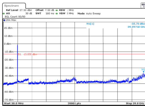
n77_3_60MHz_30kHz_3950MHz_DFT-s-OFDM QPSK_RB162@0 -35.73dBm
