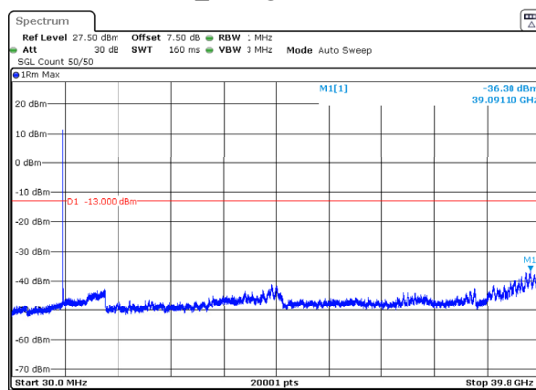
n77_3_60MHz_30kHz_3840MHz_DFT-s-OFDM QPSK_RB1@0 -36.30dBm
