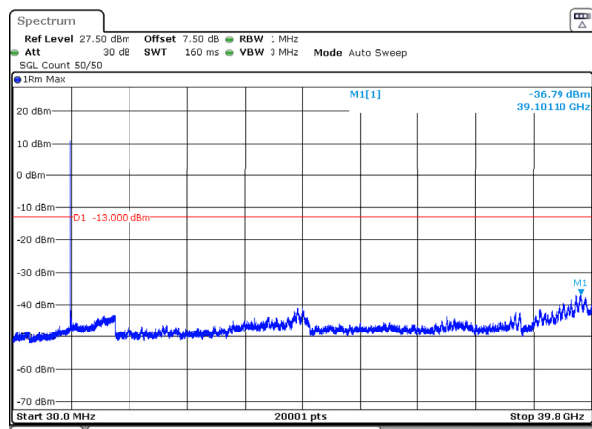
n77_3_80MHz_30kHz_3940MHz_DFT-s-OFDM QPSK_RB1@0 -36.79dBm
