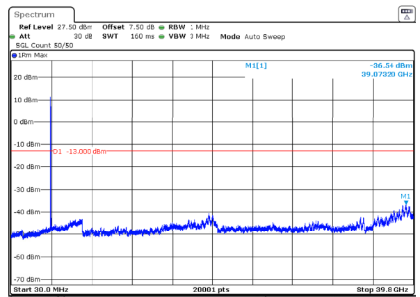
n77_3_100MHz_30kHz_3930MHz_DFT-s-OFDM QPSK_RB1@0 -36.54dBm
