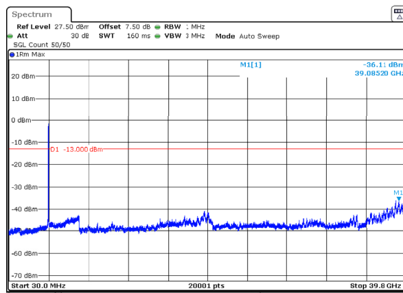
n77_3_80MHz_30kHz_3940MHz_DFT-s-OFDM QPSK_RB216@0 -36.11dBm
