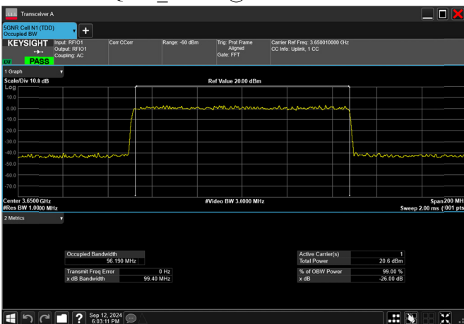
n77_2_100MHz_30kHz_3650MHz_DFT-s-OFDM 256 QAM_RB270@0 96.190MHz
