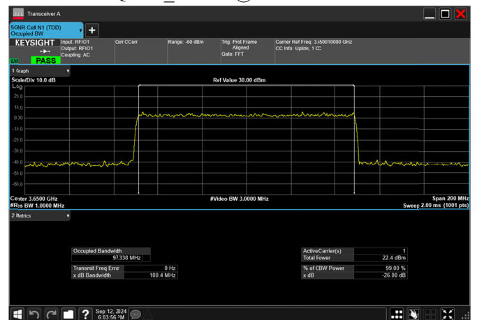
n77_2_100MHz_30kHz_3650MHz_CP-OFDM QPSK_RB273@0 97.338MHz
