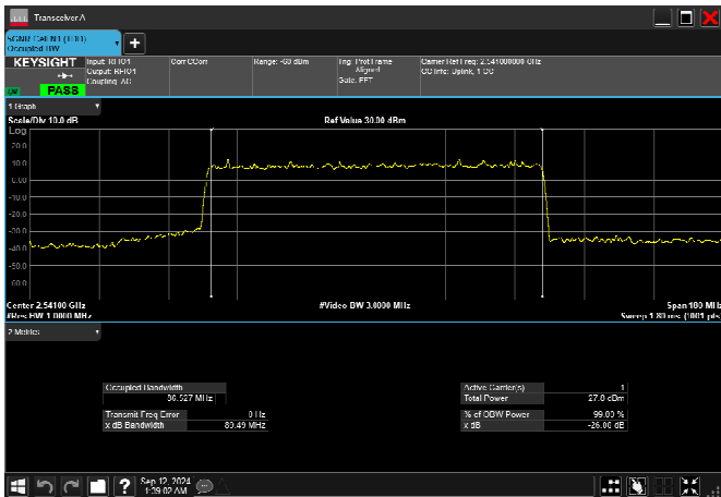
n41_90MHz_30kHz_2541MHz_DFT-s-OFDM 16 QAM_RB243@0 86.520MHz
