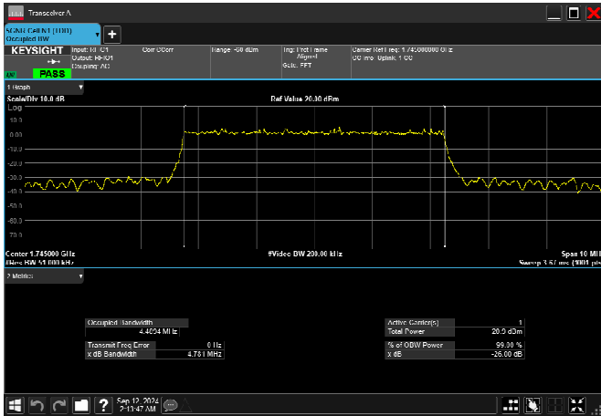
n66_5MHz_15kHz_1745MHz_CP-OFDM QPSK_RB25@0 4.468MHz
