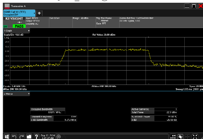
n77_1_10MHz_30kHz_3455MHz_DFT-s-OFDM 16 QAM RB24@0 8.602MHz
