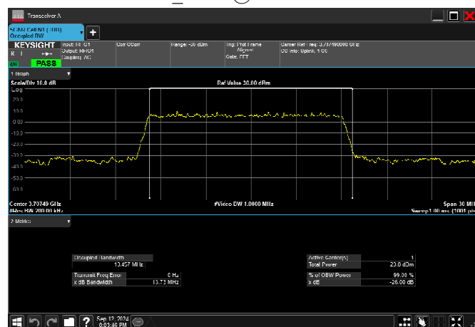
n77_3_15MHz_30kHz_3707.5MHz_DFT-s-OFDM 16 QAM RB36@0 13.500MHz
