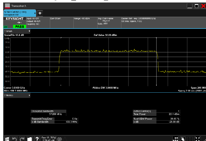
n77_3_100MHz_30kHz_3930MHz_CP-OFDM 64 QAM_RB273@0 97.288MHz
