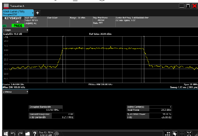
n78_1_10MHz_30kHz_3455MHz_DFT-s-OFDM QPSK_RB24@0 8.575MHz
