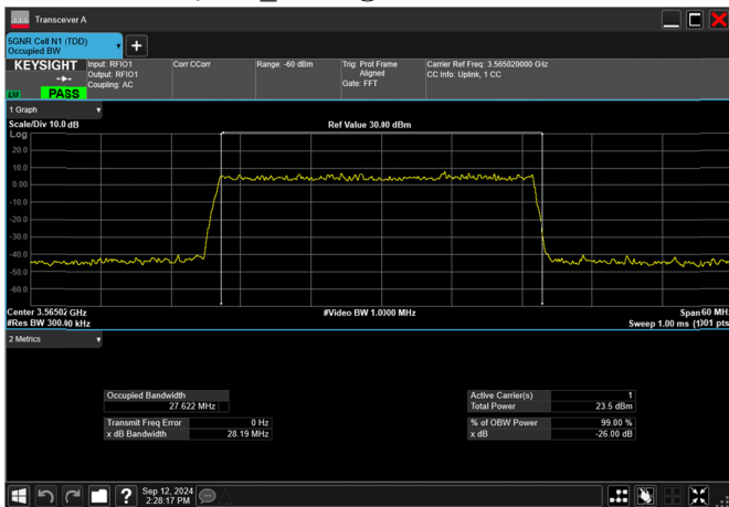
n77_2_30MHz_30kHz_3565MHz_DFT-s-OFDM QPSK_RB75@0 27.622MHz
