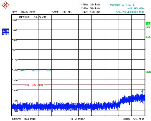
5MHz_Low_QPSK_25@0(763MHz~775MHz)
