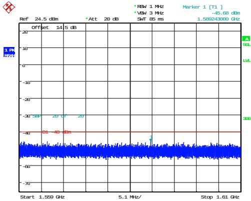
5MHz_Low_QPSK_1@0(1559MHz~1610MHz)
