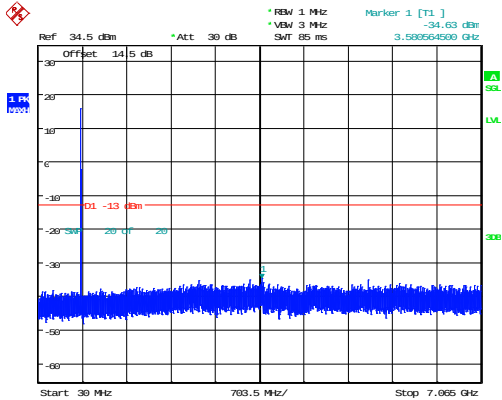
5MHz_Low_QPSK_1@0
