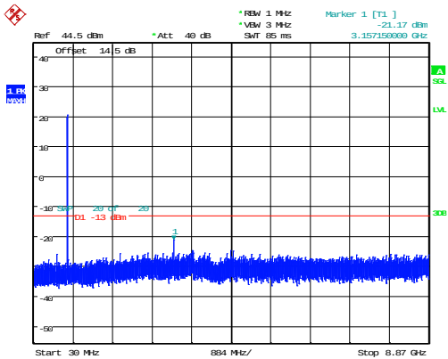
5MHz_Low_QPSK_25@0(30MHz~8.87GHz)
