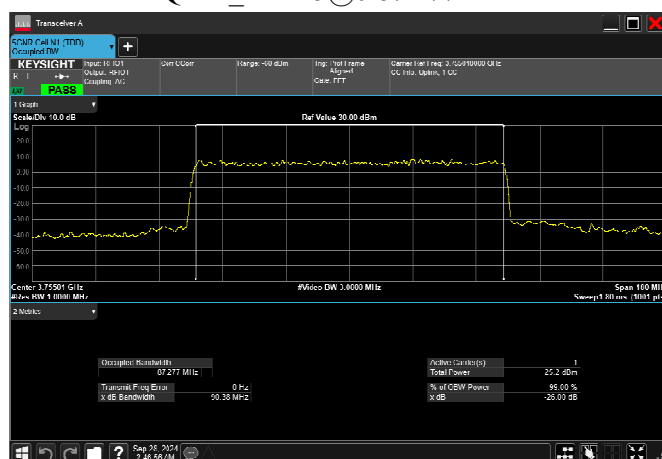
n78_3_90MHz_30kHz_3755MHz_CP-OFDM 256 OAM RB245@0 87.277MHz
