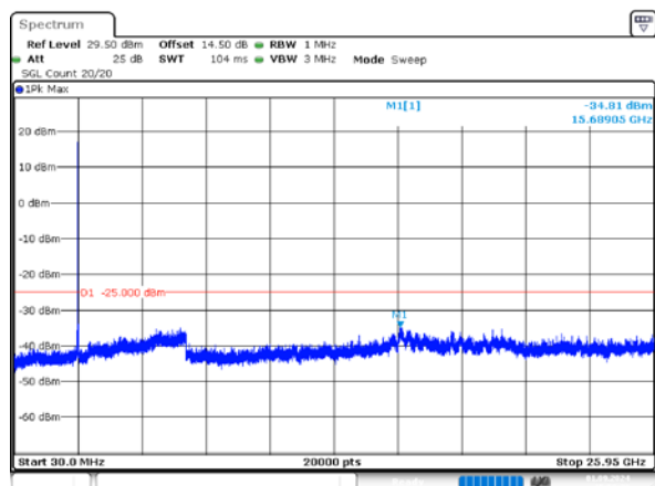
20MHz_Middle_QPSK_1@0
