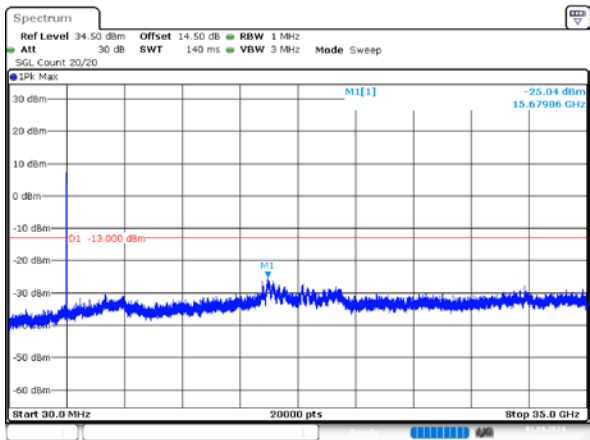
1_15MHz_Middle_QPSK_75@0
