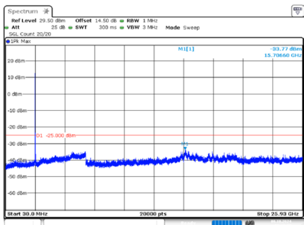
10MHz_Middle_QPSK_50@0
