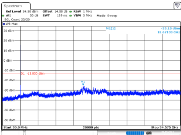
1_15MHz_Low_QPSK_1@0
