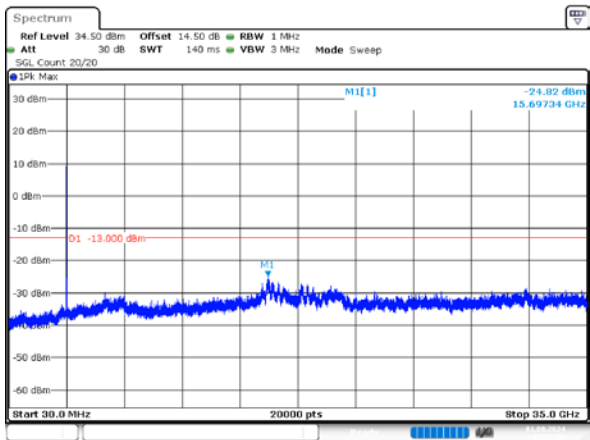
1_10MHz_Middle_QPSK_50@0
