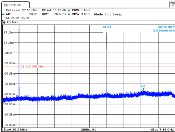
n12_15MHz_15kHz_706.5MHz_DFT-s-OFDM QPSK_RB1@0 -36.06dBm
