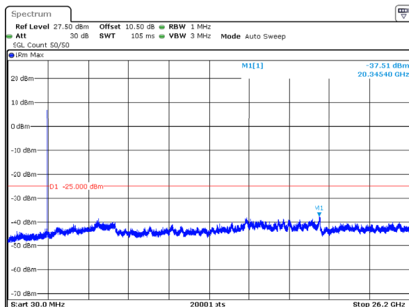
n38_10MHz_30kHz_2575MHz_DFT-s-OFDM QPSK_RB24@0 -37.51dBm
