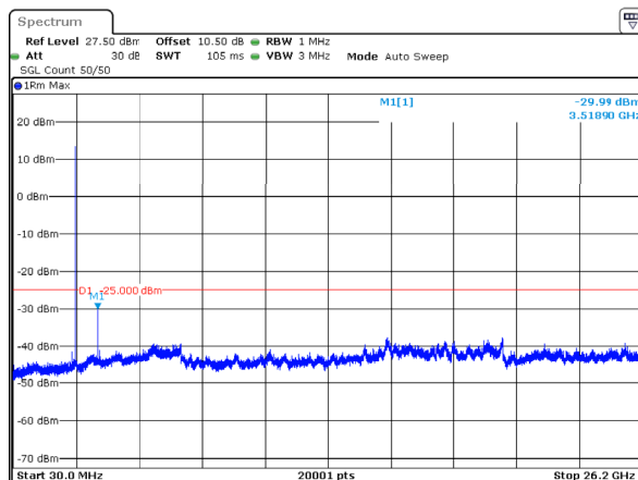
n38_10MHz_30kHz_2575MHz_DFT-s-OFDM QPSK_RB1@23 -29.99dBm
