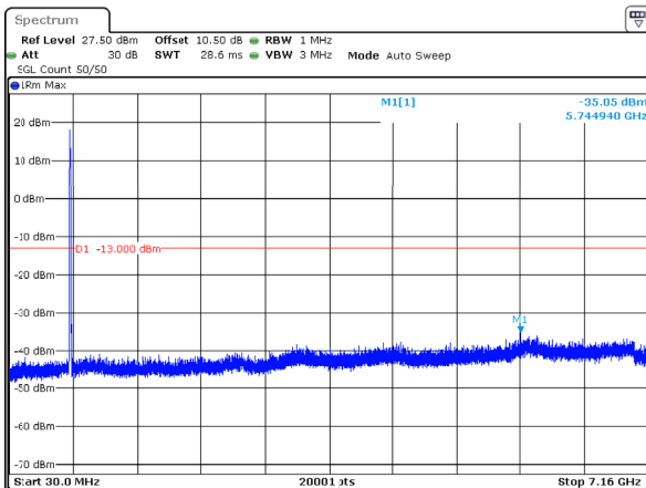
n12_10MHz_15kHz_707.5MHz_DFT-s-OFDM QPSK_RB50@0 -35.05dBm
