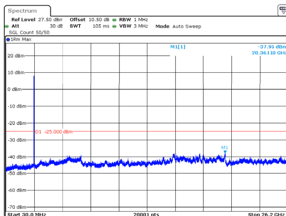
n38_10MHz_30kHz_2595MHz_DFT-s-OFDM QPSK_RB24@0 -37.95dBm
