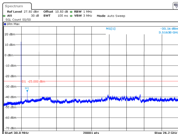
n38_10MHz_30kHz_2595MHz_DFT-s-OFDM QPSK_RB1@0 -35.16dBm
