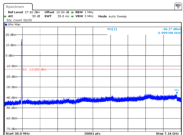
n12_15MHz_15kHz_707.5MHz_DFT-s-OFDM QPSK_RB75@0 -36.27dBm
