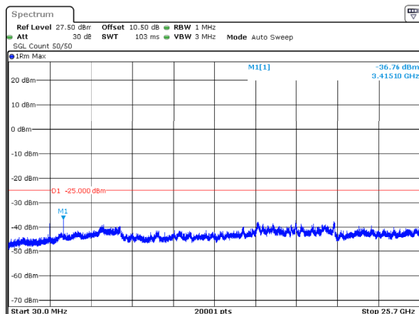
n7_10MHz_15kHz_2565MHz_DFT-s-OFDM QPSK_RB1@0 -36.76dBm
