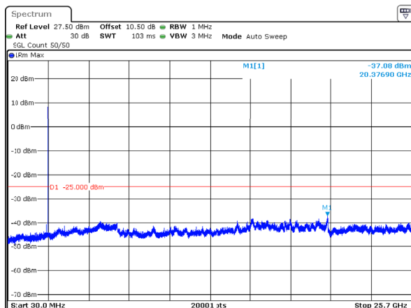
n7_5MHz_15kHz_2567.5MHz_DFT-s-OFDM QPSK_RB25@0 -37.08dBm
