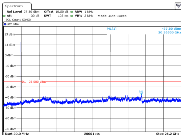
n38_10MHz_30kHz_2575MHz_DFT-s-OFDM QPSK_RB1@0 -37.80dBm
