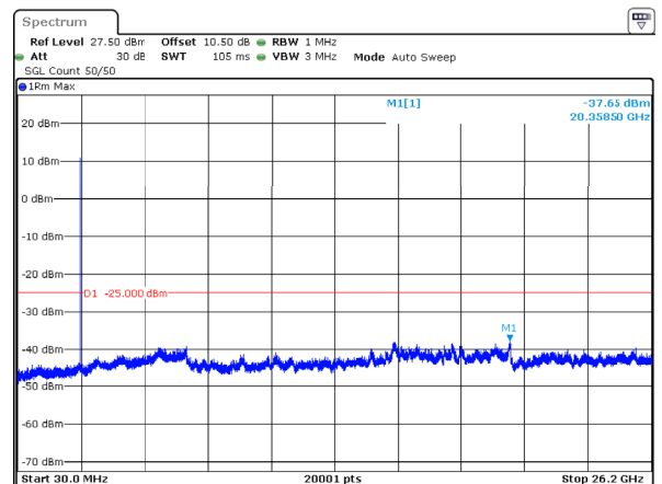
n38_5MHz_15kHz_2572.5MHz_DFT-s-OFDM QPSK_RB25@0 -37.65dBm
