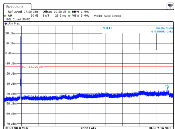
n12_10MHz_15kHz_711MHz_DFT-s-OFDM QPSK_RB50@0 -35.35dBm
