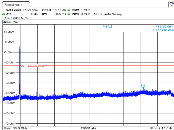
n12_15MHz_15kHz_708.5MHz_DFT-s-OFDM QPSK_RB1@0 -35.96dBm
