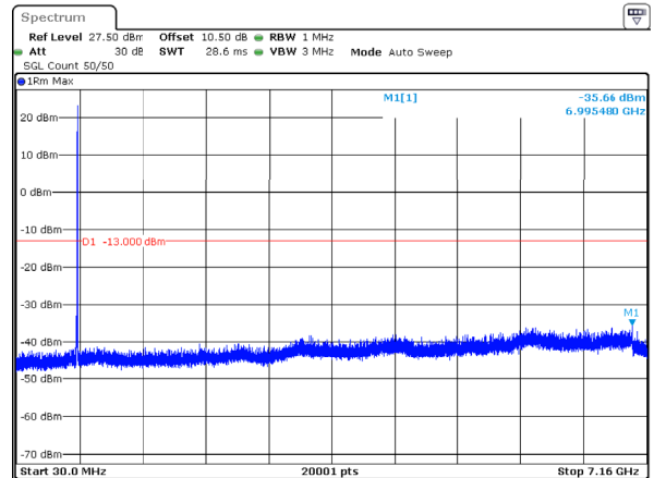
n12_10MHz_15kHz_707.5MHz_DFT-s-OFDM QPSK_RB1@51 -35.66dBm
