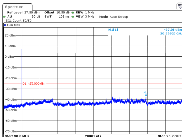
n7_10MHz_15kHz_2505MHz_DFT-s-OFDM QPSK_RB50@0 -37.08dBm
