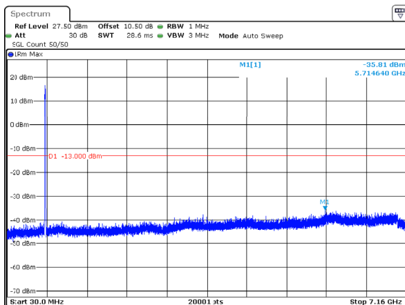
n12_15MHz_15kHz_708.5MHz_DFT-s-OFDM QPSK_RB75@0 -35.81dBm
