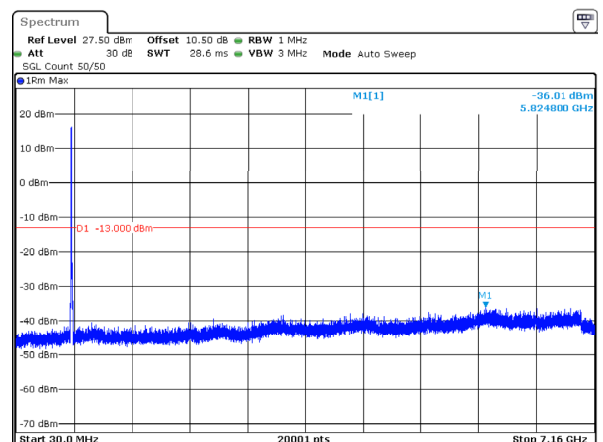
n12_10MHz_15kHz_704MHz_DFT-s-OFDM QPSK_RB50@0 -36.01dBm
