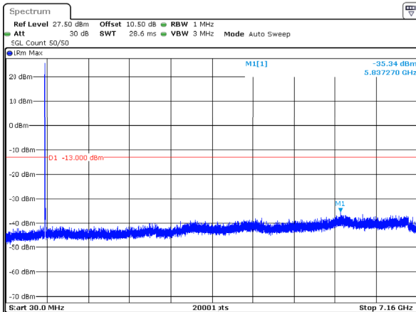
n12_10MHz_15kHz_707.5MHz_DFT-s-OFDM QPSK_RB1@0 -35.34dBm
