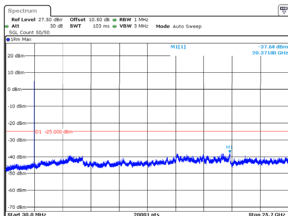
n7_10MHz_15kHz_2565MHz_DFT-s-OFDM QPSK_RB50@0 -37.60dBm
