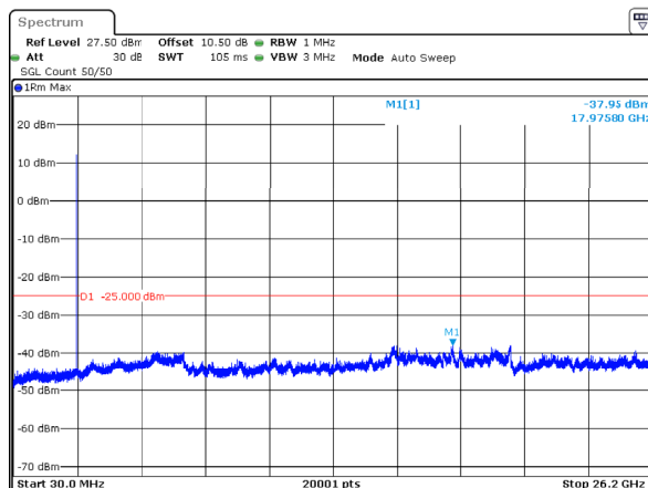
n38_15MHz_30kHz_2577.5MHz_DFT-s-OFDM QPSK_RB1@0 -37.95dBm
