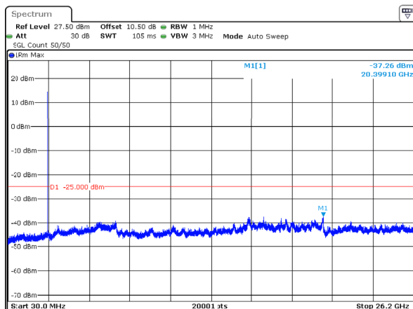
n38_15MHz_30kHz_2595MHz_DFT-s-OFDM QPSK_RB1@0 -37.26dBm
