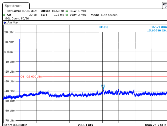
n7_10MHz_15kHz_2505MHz_DFT-s-OFDM QPSK_RB1@0 -37.78dBm
