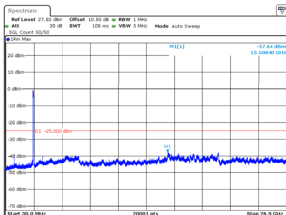
n41_100MHz_30kHz_2640MHz_DFT-s-OFDM QPSK_RB270@0 -37.64dBm
