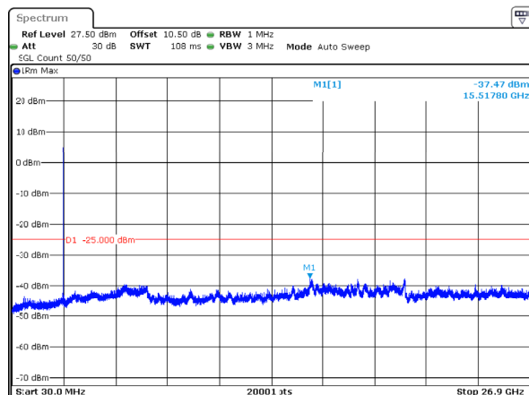
n41_20MHz_30kHz_2679.99MHz_DFT-s-OFDM QPSK_RB50@0 -37.47dBm
