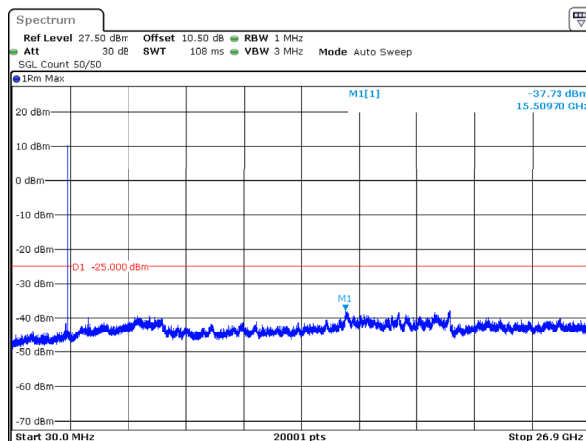
n41_90MHz_30kHz_2541MHz_DFT-s-OFDM QPSK_RB1@244 -37.73dBm
