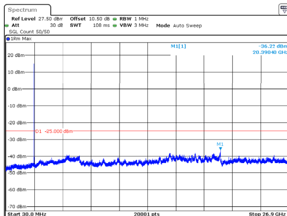
n41_30MHz_30kHz_2674.98MHz_DFT-s-OFDM QPSK_RB1@0 -36.22dBm
