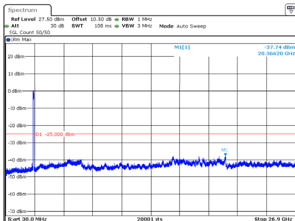
n41_100MHz_30kHz_2592.99MHz_DFT-s-OFDM QPSK_RB270@0 -37.74dBm
