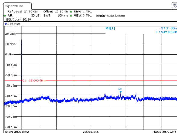
n41_20MHz_30kHz_2679.99MHz_DFT-s-OFDM QPSK_RB1@50 -37.11dBm
