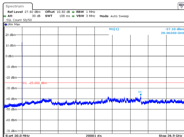
n41_20MHz_30kHz_2679.99MHz_DFT-s-OFDM QPSK_RB1@0 -37.10dBm
