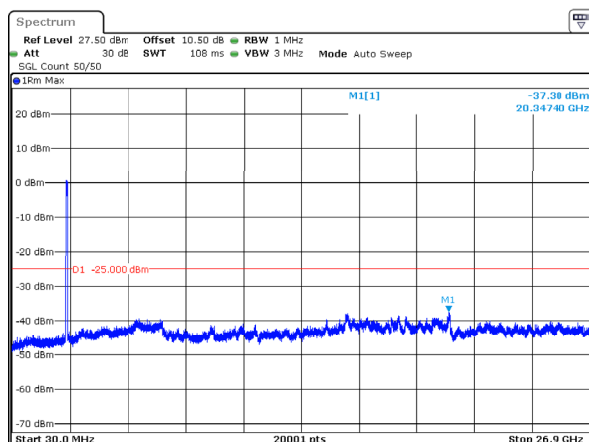
n41_80MHz_30kHz_2536.02MHz_DFT-s-OFDM QPSK_RB216@0 -37.30dBm
