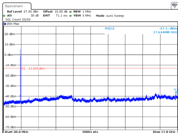
n66_20MHz_15kHz_1720MHz_DFT-s-OFDM QPSK_RB100@0 -37.11dBm
