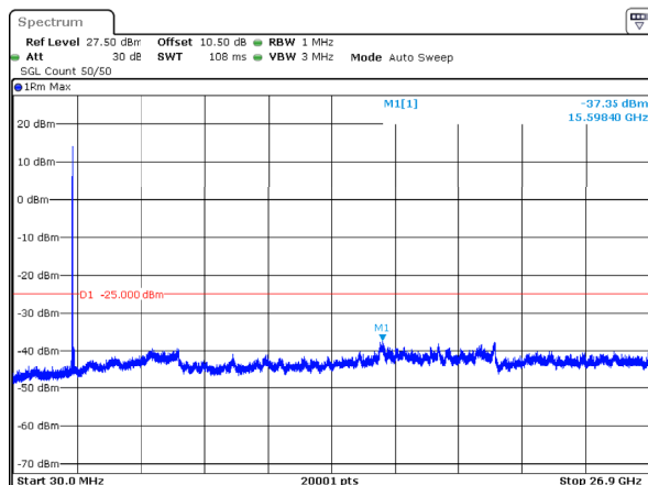
n41_80MHz_30kHz_2536.02MHz_DFT-s-OFDM QPSK_RB1@0 -37.35dBm
