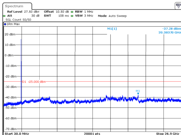
n41_60MHz_30kHz_2659.98MHz_DFT-s-OFDM QPSK_RB1@0 -37.28dBm
