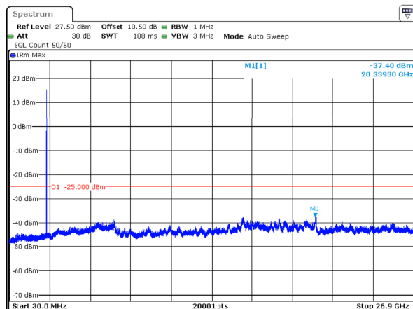
n41_20MHz_30kHz_2506.02MHz_DFT-s-OFDM QPSK_RB1@0 -37.40dBm
