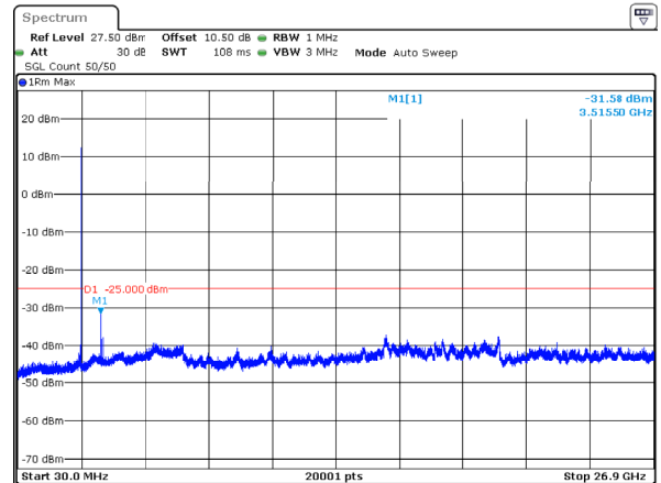
n41_90MHz_30kHz_2644.98MHz_DFT-s-OFDM QPSK_RB1@244 -31.58dBm
