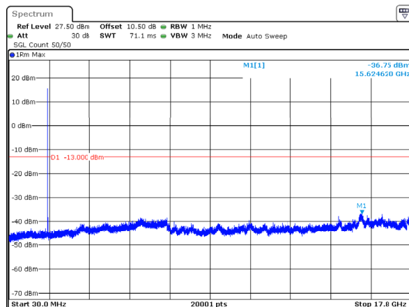
n66_25MHz_15kHz_1722.5MHz_DFT-s-OFDM QPSK_RB1@0 -36.75dBm
