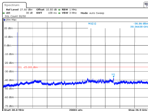
n41_50MHz_30kHz_2592.99MHz_DFT-s-OFDM QPSK_RB1@0 -36.86dBm
