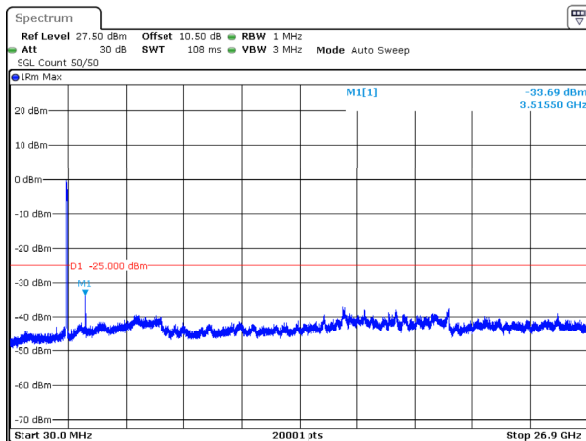
n41_90MHz_30kHz_2644.98MHz_DFT-s-OFDM QPSK_RB243@0 -33.69dBm
