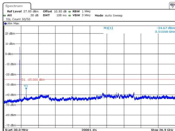
n41_20MHz_30kHz_2506.02MHz_DFT-s-OFDM QPSK_RB50@0 -34.67dBm
