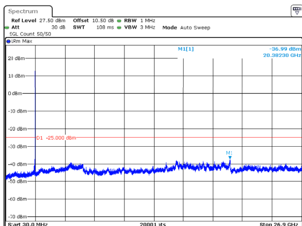
n41_80MHz_30kHz_2649.99MHz_DFT-s-OFDM QPSK_RB1@216 -36.99dBm
