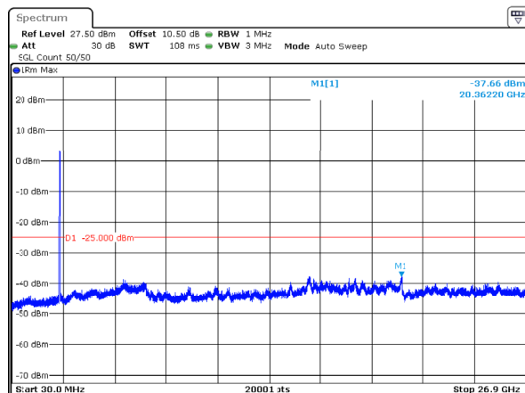
n41_40MHz_30kHz_2516.01MHz_DFT-s-OFDM QPSK_RB100@0 -37.66dBm
