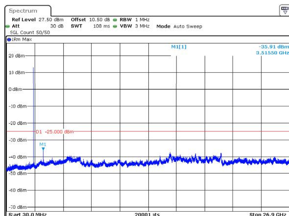
n41_40MHz_30kHz_2592.99MHz_DFT-s-OFDM QPSK_RB1@0 -35.91dBm
