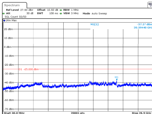
n41_80MHz_30kHz_2649.99MHz_DFT-s-OFDM QPSK_RB1@0 -37.57dBm
