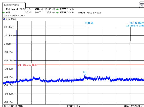
n41_40MHz_30kHz_2516.01MHz_DFT-s-OFDM QPSK_RB1@0 -37.42dBm
