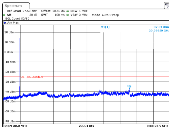
n41_30MHz_30kHz_2592.99MHz_DFT-s-OFDM QPSK_RB1@77 -37.39dBm
