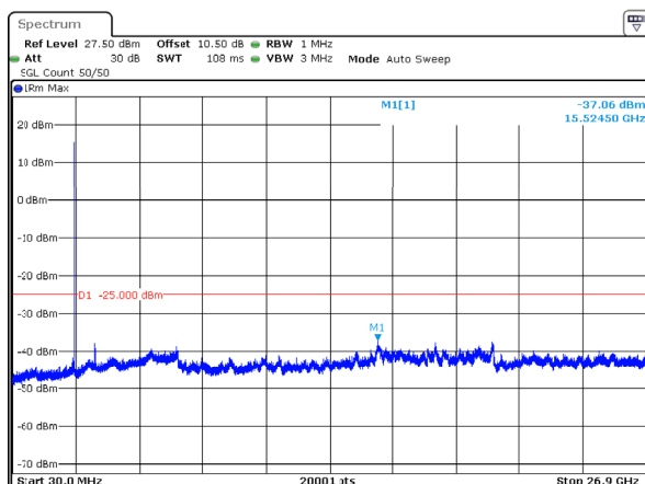
n41_90MHz_30kHz_2592.99MHz_DFT-s-OFDM QPSK_RB1@244 -37.06dBm
