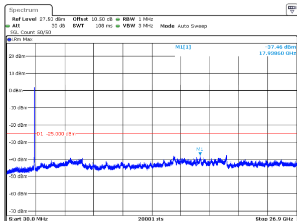
n41_50MHz_30kHz_2592.99MHz_DFT-s-OFDM QPSK_RB128@0 -37.46dBm
