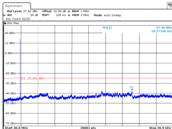
n41_20MHz_30kHz_2592.99MHz_DFT-s-OFDM QPSK_RB1@0 -37.06dBm
