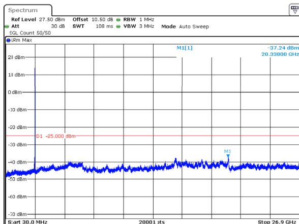
n41_60MHz_30kHz_2659.98MHz_DFT-s-OFDM QPSK_RB1@161 -37.24dBm
