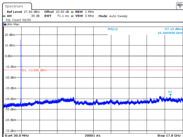
n66_20MHz_15kHz_1720MHz_DFT-s-OFDM QPSK_RB1@0 -37.15dBm
