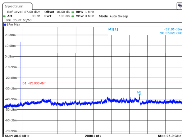
n41_90MHz_30kHz_2592.99MHz_DFT-s-OFDM QPSK_RB1@0 -37.05dBm
