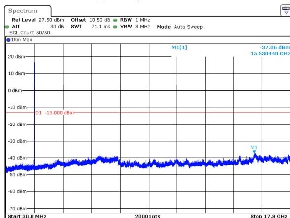
n66_25MHz_15kHz_1767.5MHz_DFT-s-OFDM QPSK_RB1@132 -37.06dBm
