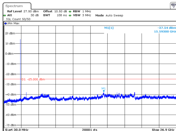
n41_15MHz_30kHz_2592.99MHz_DFT-s-OFDM QPSK_RB1@0 -37.54dBm
