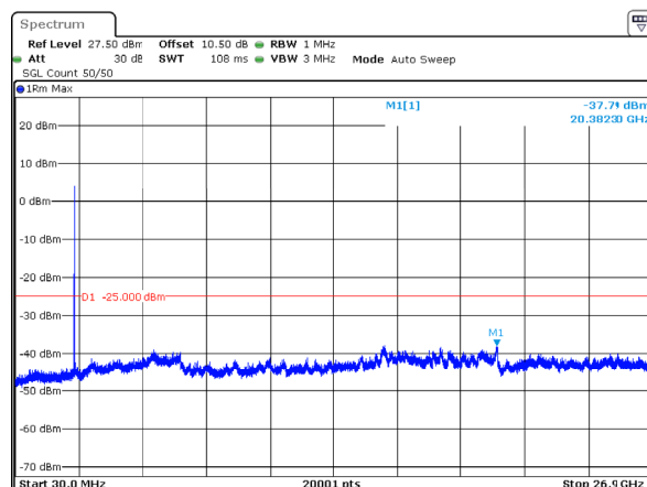
n41_30MHz_30kHz_2511MHz_DFT-s-OFDM QPSK_RB75@0 -37.79dBm
