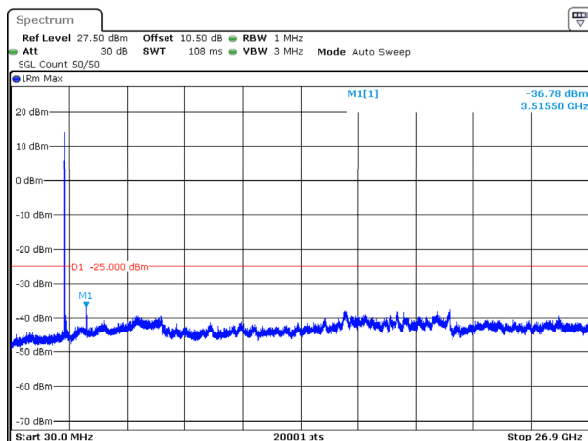
n41_90MHz_30kHz_2541MHz_DFT-s-OFDM QPSK_RB1@0 -36.78dBm
