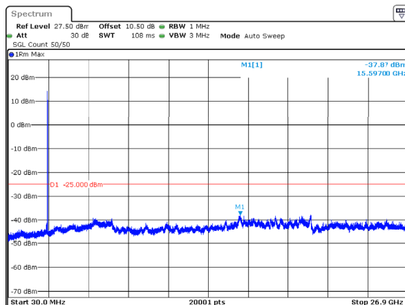
n41_80MHz_30kHz_2592.99MHz_DFT-s-OFDM QPSK_RB1@216 -37.87dBm
