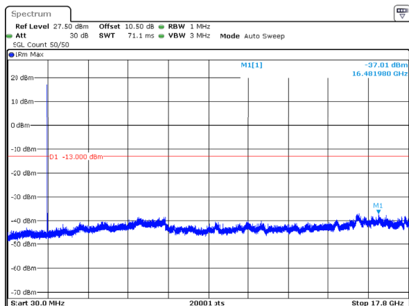
n66_15MHz_15kHz_1772.5MHz_DFT-s-OFDM QPSK_RB1@0 -37.01dBm
