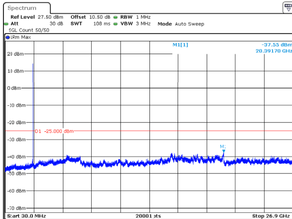
n41_90MHz_30kHz_2644.98MHz_DFT-s-OFDM QPSK_RB1@0 -37.55dBm
