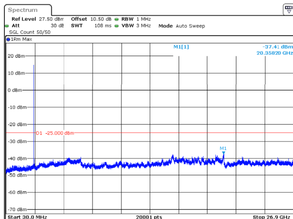
n41_100MHz_30kHz_2640MHz_DFT-s-OFDM QPSK_RB1@0 -37.41dBm
