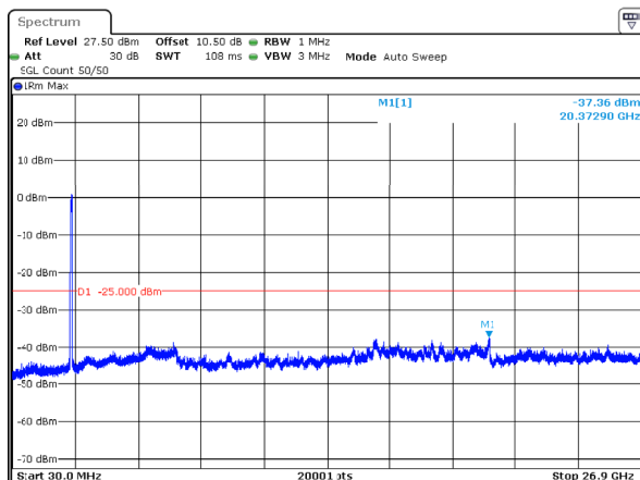
n41_90MHz_30kHz_2541MHz_DFT-s-OFDM QPSK_RB243@0 -37.36dBm
