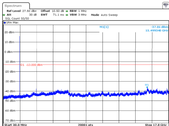
n66_15MHz_15kHz_1745MHz_DFT-s-OFDM QPSK_RB1@0 -37.05dBm
