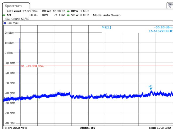
n66_15MHz_15kHz_1717.5MHz_DFT-s-OFDM QPSK_RB1@0 -36.85dBm
