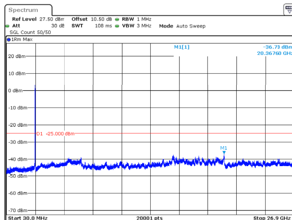
n41_50MHz_30kHz_2664.99MHz_DFT-s-OFDM QPSK_RB128@0 -36.73dBm
