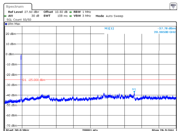
n41_100MHz_30kHz_2546.01MHz_DFT-s-OFDM QPSK_RB270@0 -37.70dBm
