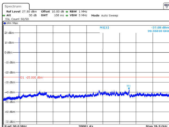
n41_80MHz_30kHz_2536.02MHz_DFT-s-OFDM QPSK_RB1@216 -37.08dBm
