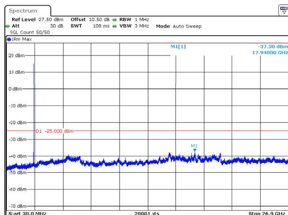
n41_20MHz_30kHz_2592.99MHz_DFT-s-OFDM QPSK_RB1@50 -37.30dBm
