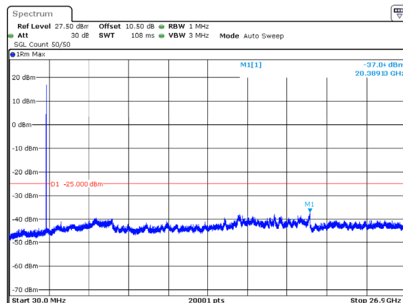
n41_30MHz_30kHz_2511MHz_DFT-s-OFDM QPSK_RB1@0 -37.04dBm
