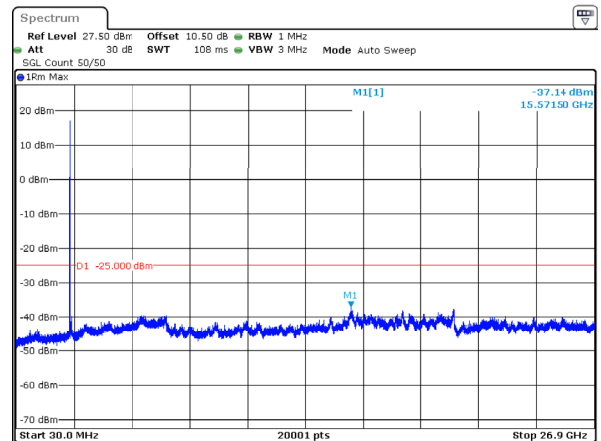
n41_100MHz_30kHz_2546.01MHz_DFT-s-OFDM QPSK_RB1@0 -37.14dBm
