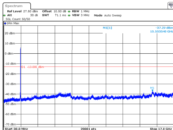
n66_25MHz_15kHz_1745MHz_DFT-s-OFDM QPSK_RB128@0 -37.29dBm
