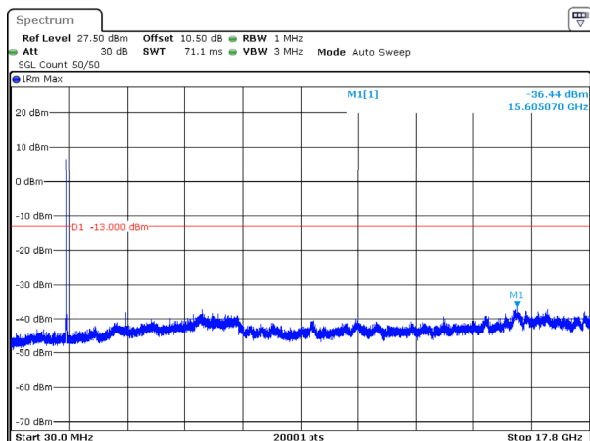
n66_15MHz_15kHz_1717.5MHz_DFT-s-OFDM QPSK_RB75@0 -36.44dBm
