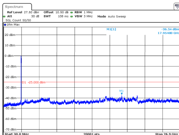
n41_80MHz_30kHz_2649.99MHz_DFT-s-OFDM QPSK_RB216@0 -36.54dBm
