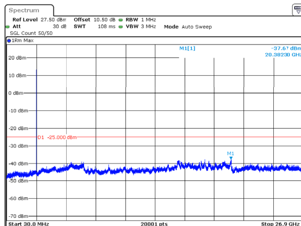
n41_15MHz_30kHz_2682.48MHz_DFT-s-OFDM QPSK_RB1@0 -37.67dBm
