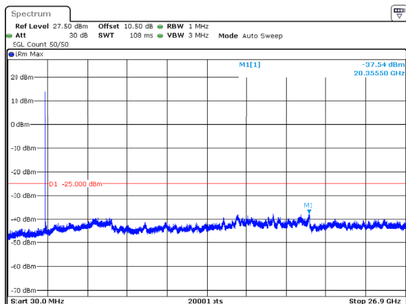
n41_80MHz_30kHz_2592.99MHz_DFT-s-OFDM QPSK_RB1@0 -37.54dBm
