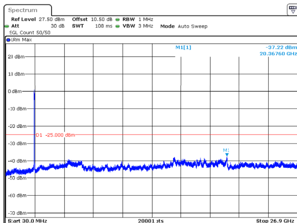
n41_60MHz_30kHz_2659.98MHz_DFT-s-OFDM QPSK_RB162@0 -37.22dBm
