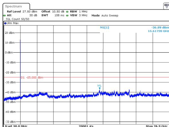
n41_15MHz_30kHz_2682.48MHz_DFT-s-OFDM QPSK_RB1@37 -36.89dBm
