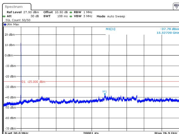
n41_30MHz_30kHz_2674.98MHz_DFT-s-OFDM QPSK_RB1@77 -37.79dBm
