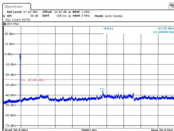
n41_90MHz_30kHz_2592.99MHz_DFT-s-OFDM QPSK_RB243@0 -37.53dBm
