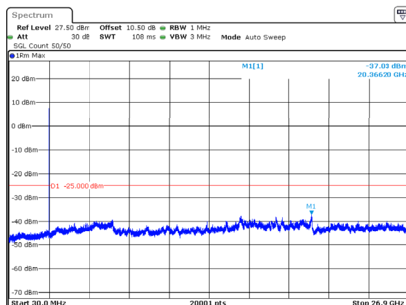
n41_15MHz_30kHz_2682.48MHz_DFT-s-OFDM QPSK_RB36@0 -37.03dBm
