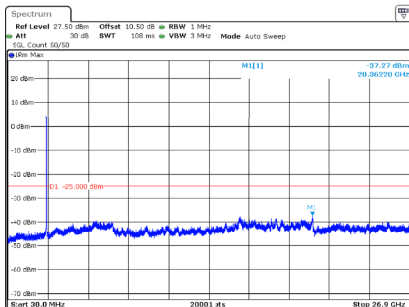
n41_30MHz_30kHz_2592.99MHz_DFT-s-OFDM QPSK_RB75@0 -37.27dBm
