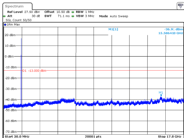
n66_20MHz_15kHz_1720MHz_DFT-s-OFDM QPSK_RB1@105 -36.91dBm
