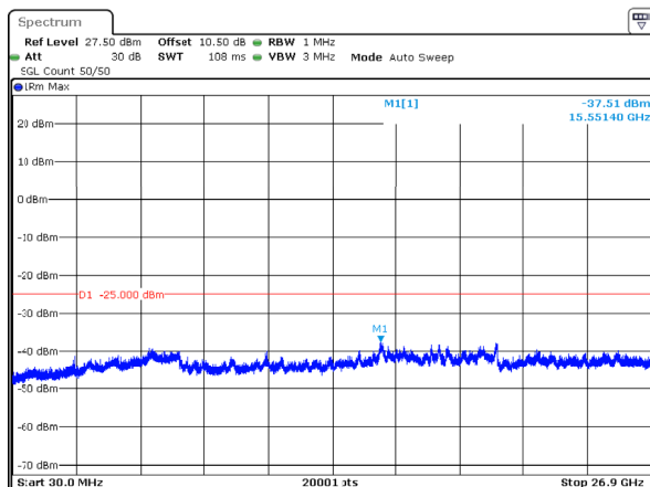
n41_100MHz_30kHz_2592.99MHz_DFT-s-OFDM QPSK_RB1@0 -37.51dBm
