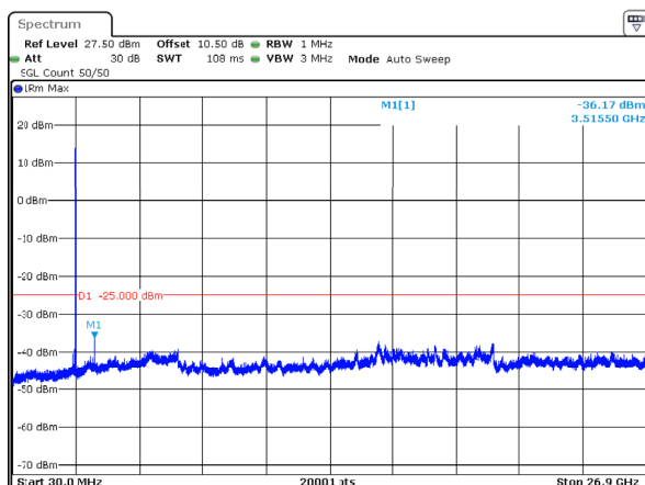
n41_100MHz_30kHz_2640MHz_DFT-s-OFDM QPSK_RB1@272 -36.17dBm
