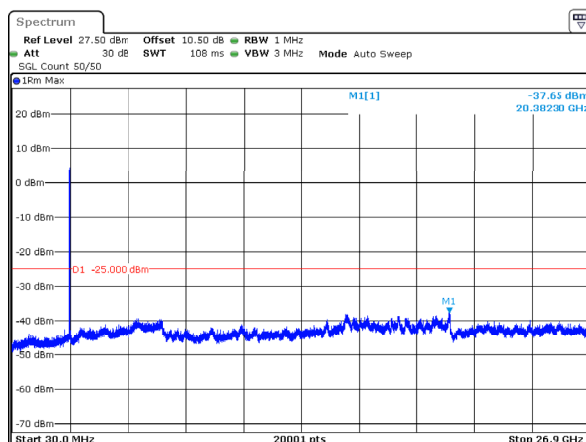
n41_30MHz_30kHz_2674.98MHz_DFT-s-OFDM QPSK_RB75@0 -37.65dBm
