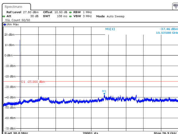
n41_100MHz_30kHz_2546.01MHz_DFT-s-OFDM QPSK_RB1@272 -37.46dBm
