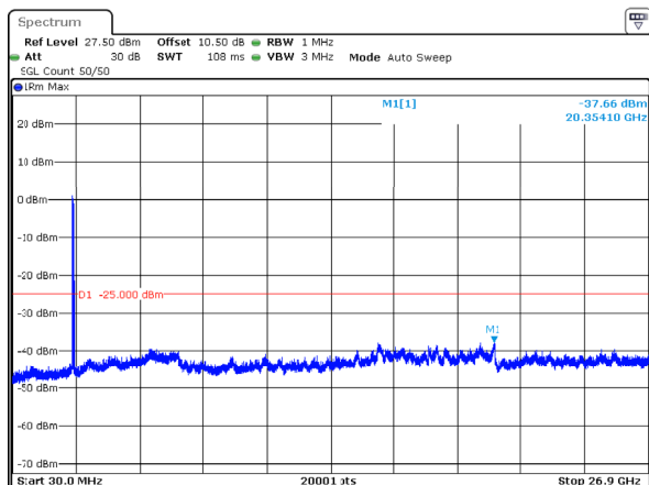
n41_80MHz_30kHz_2592.99MHz_DFT-s-OFDM QPSK_RB216@0 -37.66dBm
