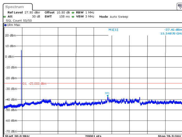
n41_20MHz_30kHz_2592.99MHz_DFT-s-OFDM QPSK_RB50@0 -37.45dBm
