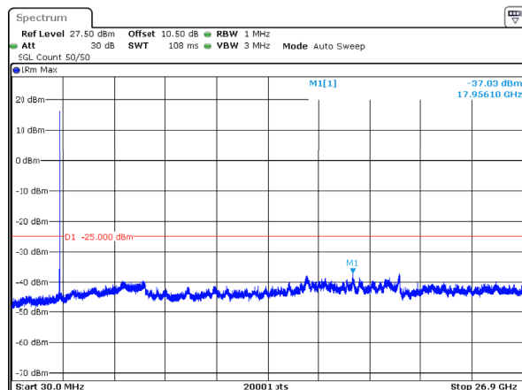
n41_40MHz_30kHz_2516.01MHz_DFT-s-OFDM QPSK_RB1@105 -37.03dBm
