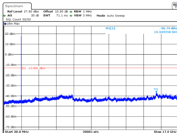
n66_25MHz_15kHz_1767.5MHz_DFT-s-OFDM QPSK_RB1@0 -36.74dBm
