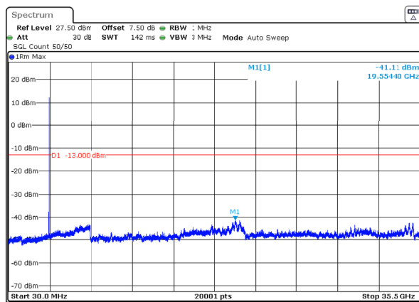
n77_1_20MHz_30kHz_3460MHz_DFT-s-OFDM QPSK_RB1@50 -41.11dBm
