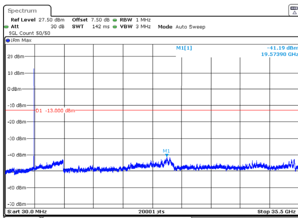
n77_1_40MHz_30kHz_3470MHz_DFT-s-OFDM QPSK_RB1@105 -41.19dBm
