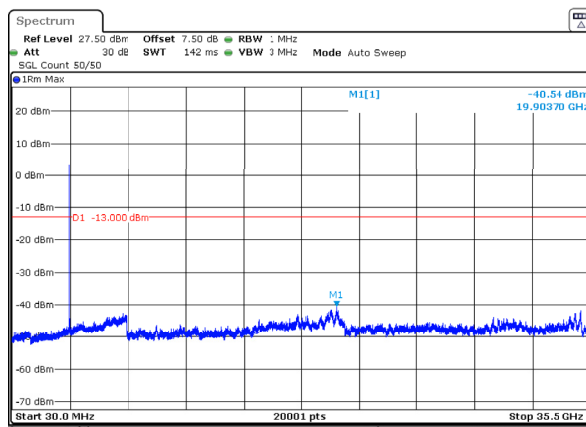
n77_1_20MHz_30kHz_3500MHz_DFT-s-OFDM QPSK_RB50@0 -40.54dBm
