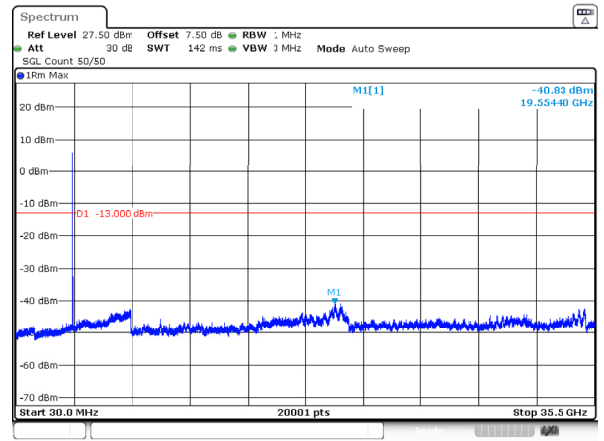
n77_1_10MHz_30kHz_3455MHz_DFT-s-OFDM QPSK_RB24@0 -40.83dBm
