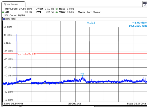
n77_1_30MHz_30kHz_3465MHz_DFT-s-OFDM QPSK_RB1@77 -41.03dBm
