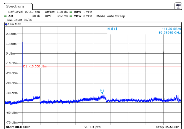
n77_1_30MHz_30kHz_3535MHz_DFT-s-OFDM QPSK_RB1@0 -41.03dBm
