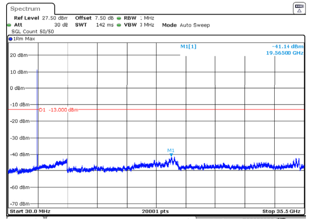
n77_1_40MHz_30kHz_3470MHz_DFT-s-OFDM QPSK_RB1@0 -41.14dBm
