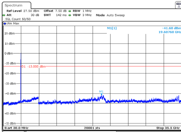
n77_1_40MHz_30kHz_3530MHz_DFT-s-OFDM QPSK_RB100@0 -41.60dBm
