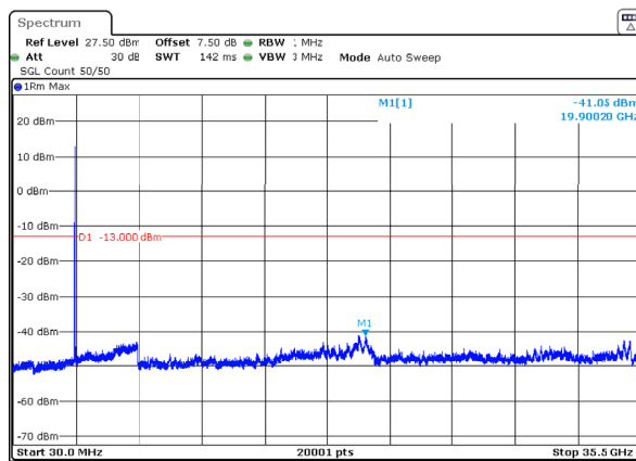
n77_1_70MHz_30kHz_3500MHz_DFT-s-OFDM QPSK_RB1@0 -41.05dBm
