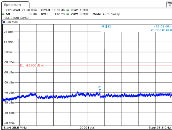
n77_1_10MHz_30kHz_3455MHz_DFT-s-OFDM QPSK_RB1@23 -38.01dBm
