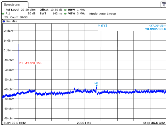
n77_1_10MHz_30kHz_3455MHz_DFT-s-OFDM QPSK_RB24@0 -37.35dBm
