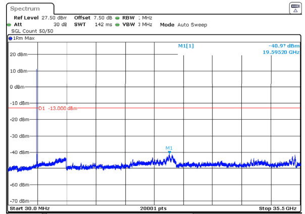
n77_1_60MHz_30kHz_3480MHz_DFT-s-OFDM QPSK_RB1@0 -40.97dBm
