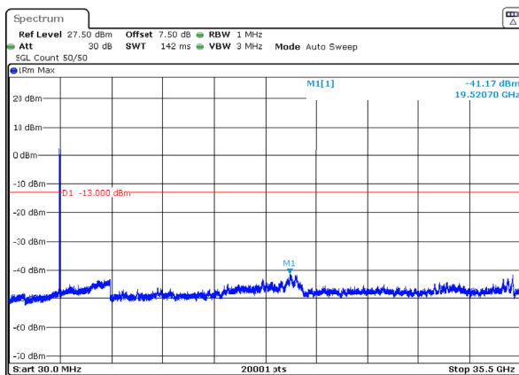
n77_1_30MHz_30kHz_3500MHz_DFT-s-OFDM QPSK_RB75@0 -41.17dBm
