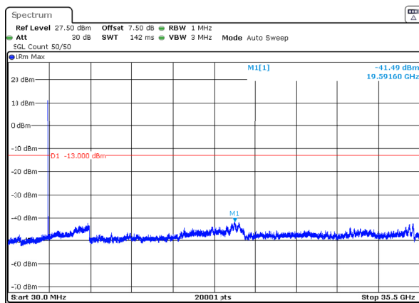
n77_1_20MHz_30kHz_3460MHz_DFT-s-OFDM QPSK_RB1@0 -41.49dBm
