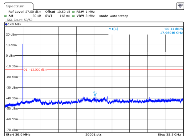
n77_1_10MHz_30kHz_3500MHz_DFT-s-OFDM QPSK_RB1@23 -38.10dBm
