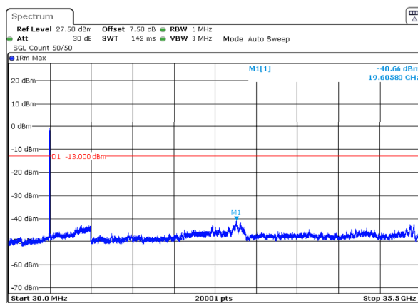
n77_1_70MHz_30kHz_3515MHz_DFT-s-OFDM QPSK_RB180@0 -40.66dBm
