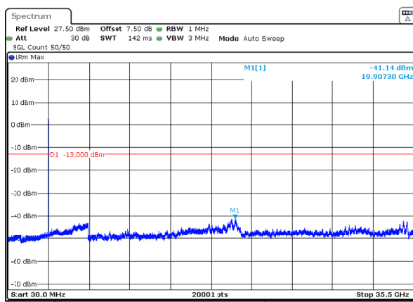
n77_1_20MHz_30kHz_3540MHz_DFT-s-OFDM QPSK_RB50@0 -41.14dBm
