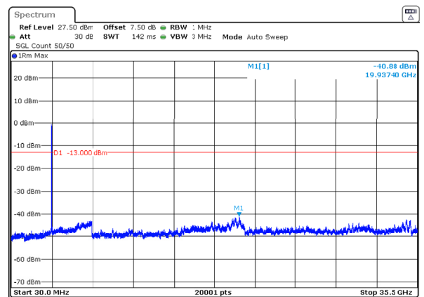
n77_1_60MHz_30kHz_3500MHz_DFT-s-OFDM QPSK_RB162@0 -40.88dBm
