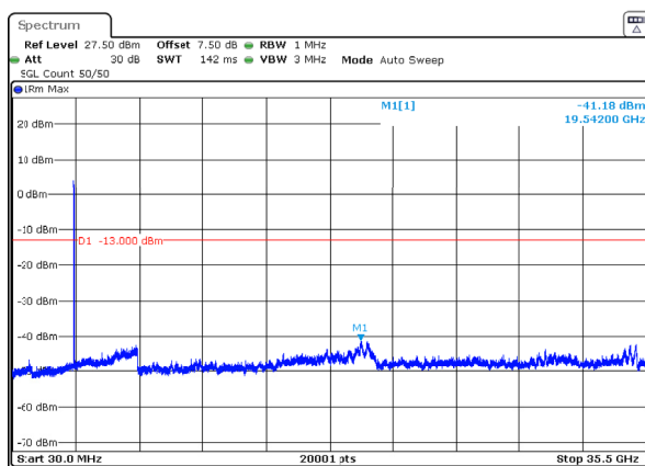
n77_1_20MHz_30kHz_3460MHz_DFT-s-OFDM QPSK_RB50@0 -41.18dBm
