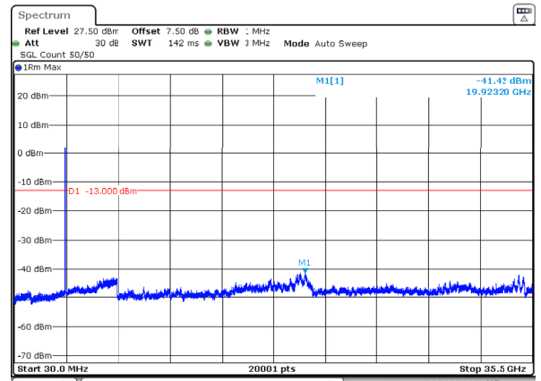
n77_1_30MHz_30kHz_3465MHz_DFT-s-OFDM QPSK_RB75@0 -41.42dBm
