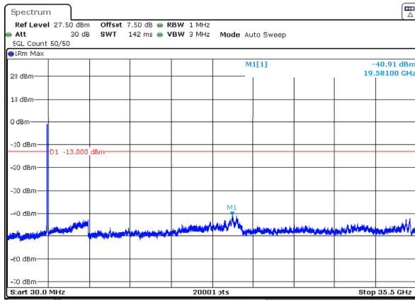
n77_1_60MHz_30kHz_3480MHz_DFT-s-OFDM QPSK_RB162@0 -40.91dBm
