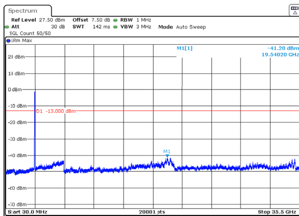
n77_1_70MHz_30kHz_3500MHz_DFT-s-OFDM QPSK_RB180@0 -41.20dBm
