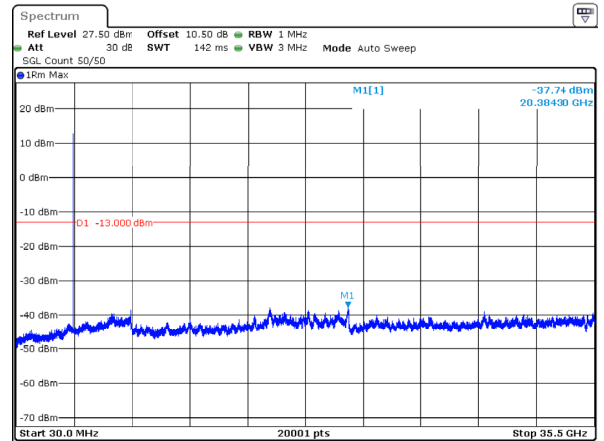
n77_1_10MHz_30kHz_3500MHz_DFT-s-OFDM QPSK_RB1@0 -37.74dBm
