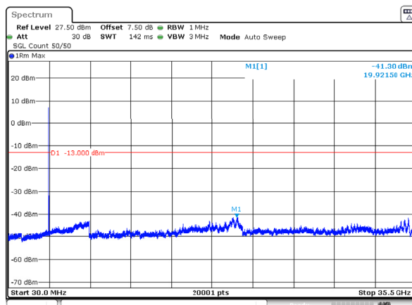
n77_1_10MHz_30kHz_3500MHz_DFT-s-OFDM QPSK_RB24@0 -41.30dBm
