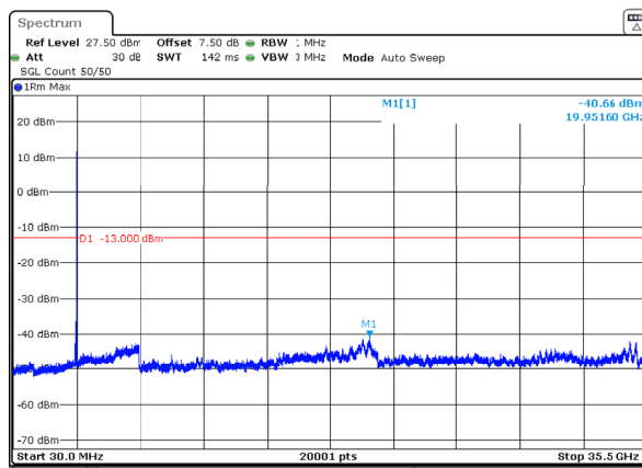
n77_1_70MHz_30kHz_3485MHz_DFT-s-OFDM QPSK_RB1@188 -40.66dBm
