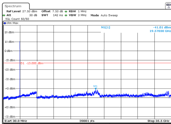
n77_1_20MHz_30kHz_3500MHz_DFT-s-OFDM QPSK_RB1@50 -41.01dBm
