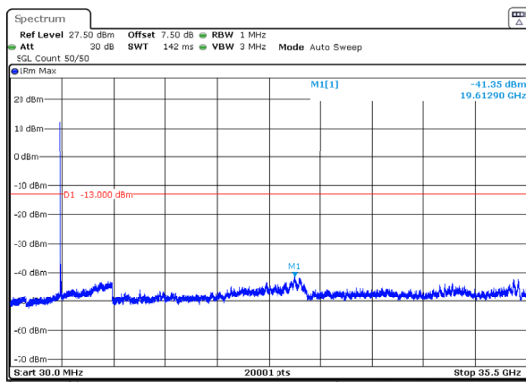
n77_1_70MHz_30kHz_3485MHz_DFT-s-OFDM QPSK_RB1@0 -41.35dBm
