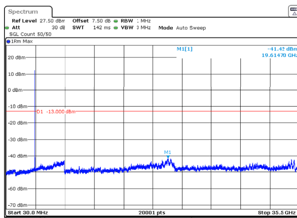
n77_1_30MHz_30kHz_3465MHz_DFT-s-OFDM QPSK_RB1@0 -41.42dBm
