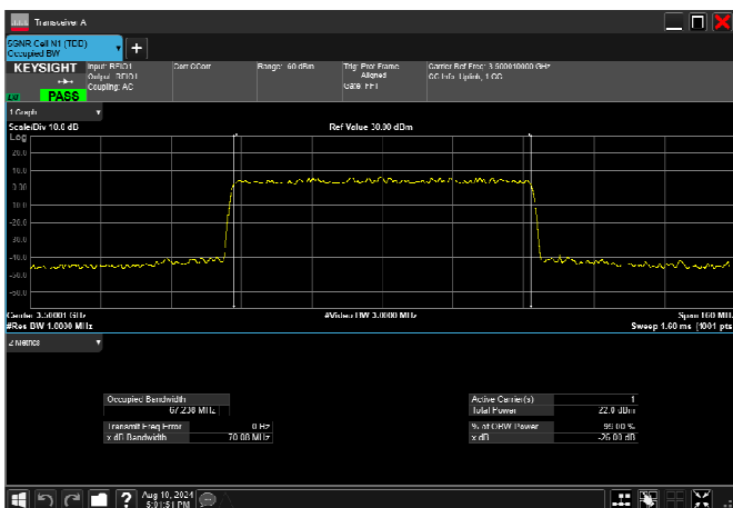
n77_1_70MHz_30kHz_3500MHz_CP-OFDM 64 QAM_RB189@0 67.238MHz
