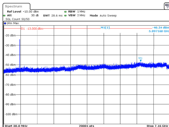
n12_10MHz_15kHz_704MHz_DFT-s-OFDM QPSK_RB50@0 -46.54dBm
