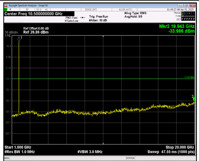
Band4-20MHz-QPSK-20050-1RB#0-Range2:1000~20000MHz
