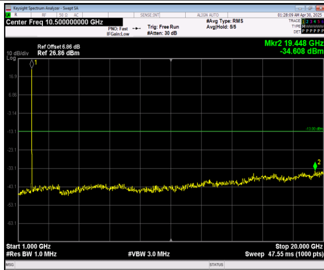
Band2-20MHz-64QAM-18900-1RB#0-Range2:1000~20000MHz
