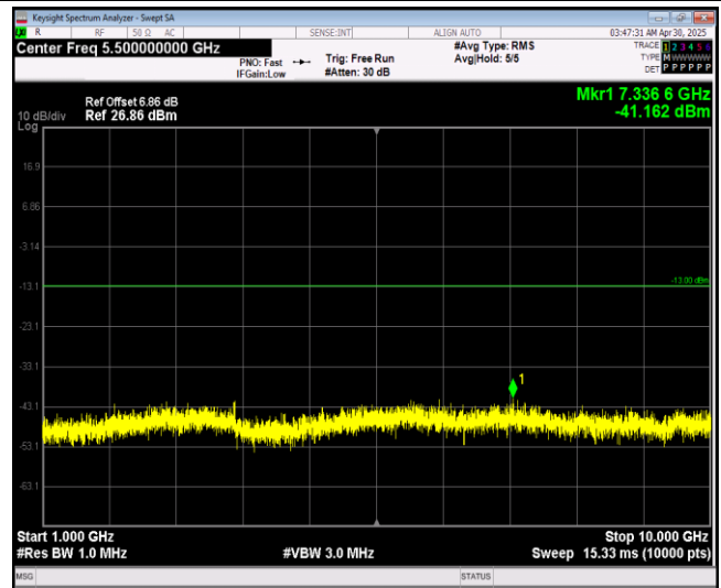
Band5-10MHz-QPSK-20525-1RB#0-Range2:1000~1 0000MHz
