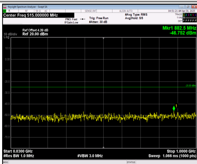
Band12-1.4MHz-QPSK-23017-1RB#0-Range1:30~1000MHz
