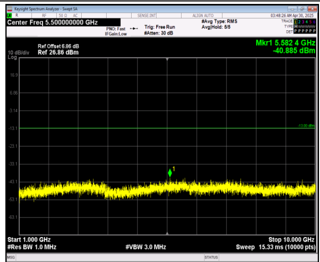
Band5-10MHz-QPSK-20600-1RB#0-Range2:1000~1 0000MHz
