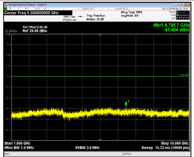
Band12-10MHz-QPSK-23060-1RB#0-Range2:1000~ 10000MHz
