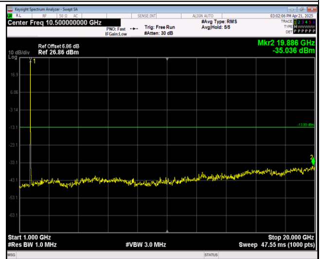
Band4-20MHz-QPSK-20300-1RB#0-Range2:1000~2 0000MHz
