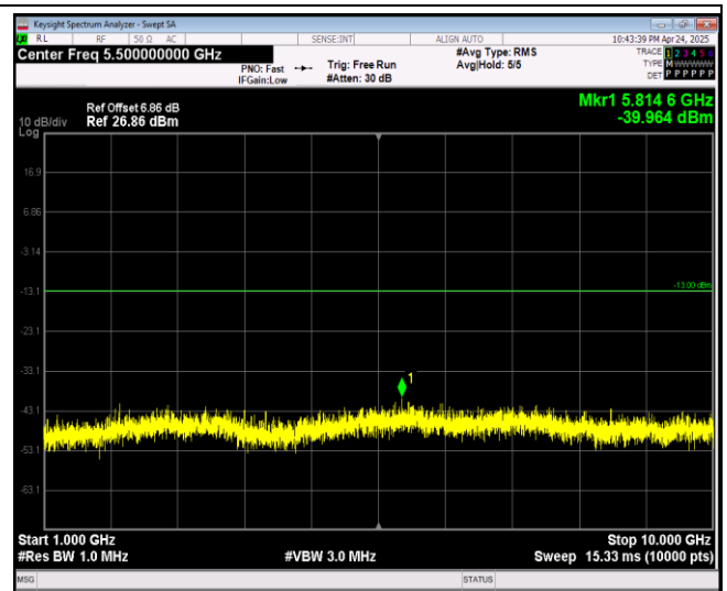
Band26-1.4MHz-QPSK-26797-1RB#0-Range2:1000~10000MHz
