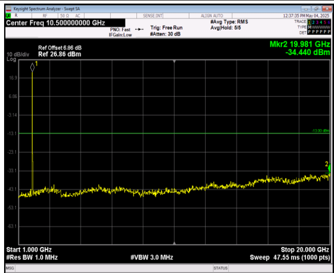
Band2-20MHz-64QAM-18900-1RB#0-Range2:1000~20000MHz
