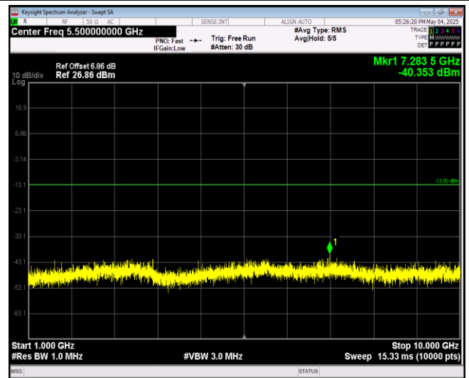
Band13-5MHz-QPSK-23230-1RB#0-Range2:1000~1 0000MHz
