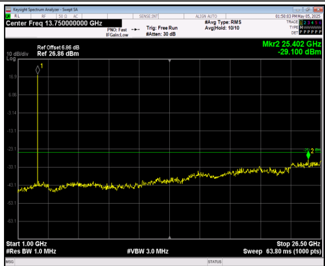
Band41-20MHz-QPSK-40140-1RB#0-Range2:1000~26500MHz
