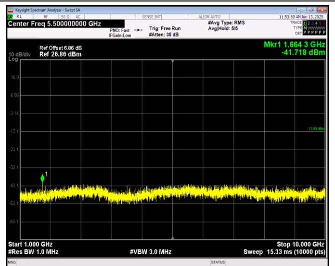
Band5-10MHz-QPSK-20600-1RB#0-Range2:1000~10 000MHz
