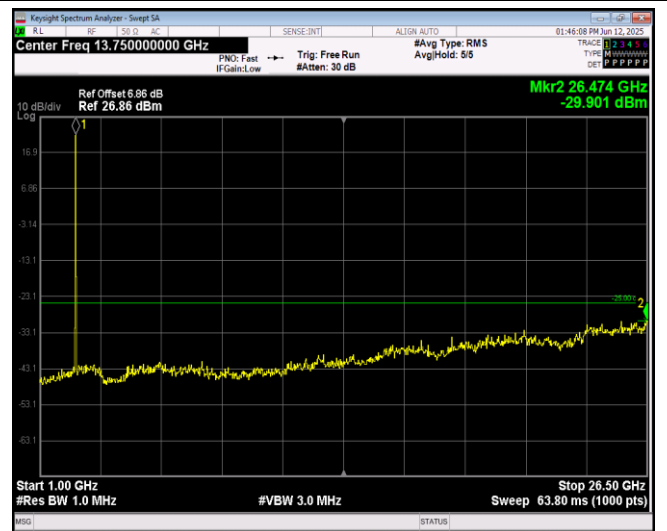
Band7-20MHz-16QAM-21100-1RB#0-Range2:1000~2 6500MHz
