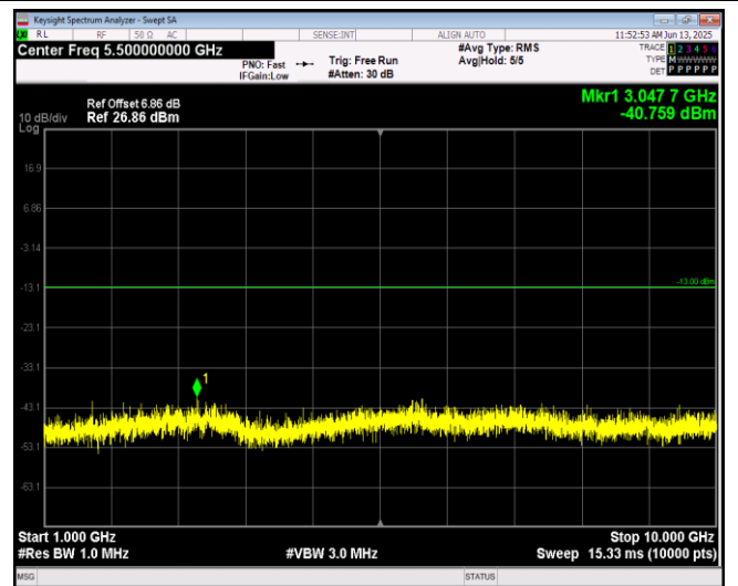
Band5-10MHz-QPSK-20525-1RB#0-Range2:1000~10 000MHz
