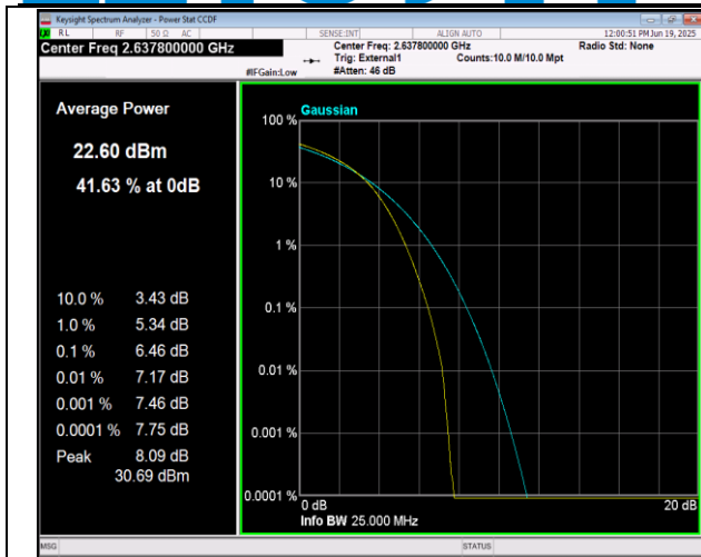
41(2555-2655)-41(2555-2655)-15MHz-10MHz-QPSK-QPS K-40315-40435-75RB#0-50RB#0-PASS
