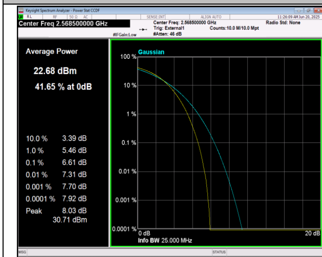
41(2555-2655)-41(2555-2655)-15MHz-10MHz-QPSK-QPS K-40691-40811-75RB#0-50RB#0-PASS
