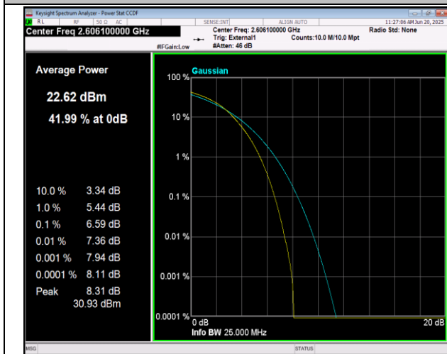
41(2555-2655)-41(2555-2655)-15MHz-10MHz-QPSK-QPS K-41067-41187-75RB#0-50RB#0-PASS
