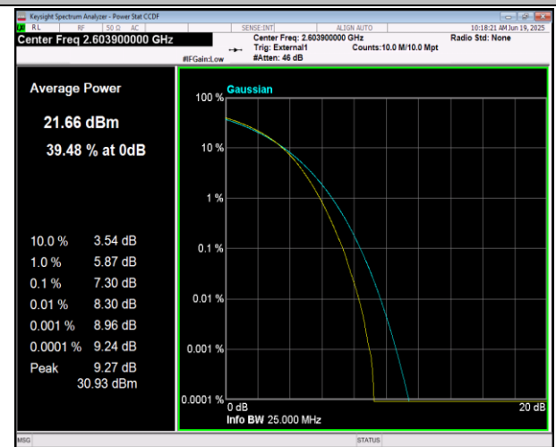
41(2555-2655)-41(2555-2655)-10MHz-15MHz-16QAM-16 QAM-41045-41165-50RB#0-75RB#0-PASS
