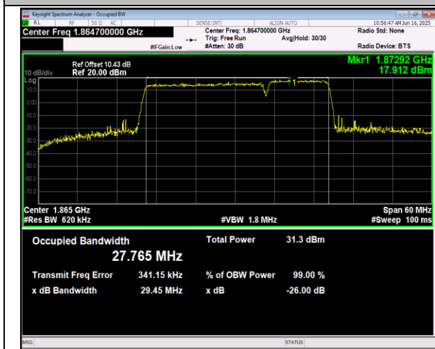
2-2-20MHz-10MHz-QPSK-QPSK-18851-18995-100RB#0-50RB#0-PASS
