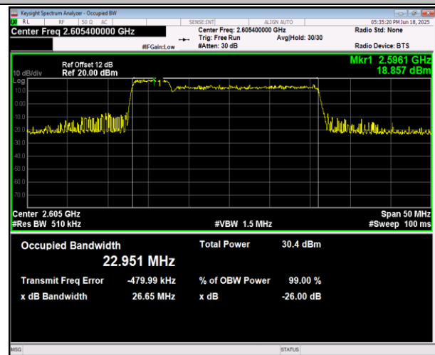
41(2555-2655)-41(2555-2655)-5MHz-20MHz-16QAM-16QA M-41023-41140-25RB#0-100RB#0-PASS
