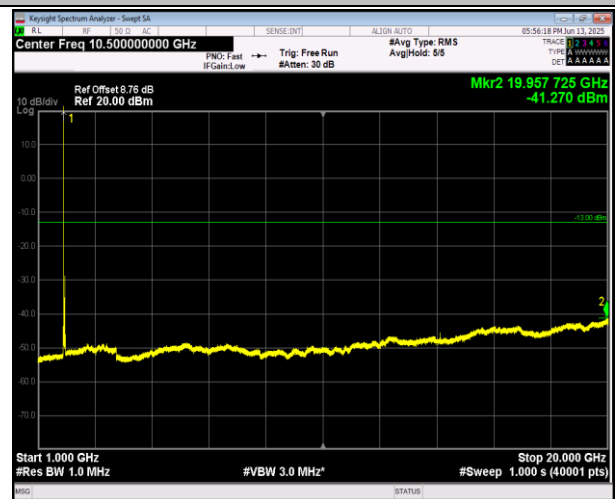
2-2-5MHz-20MHz-16QAM-16QAM-18633-18750-1RB#0-1R B#99-1000~20000MHz-PASS
