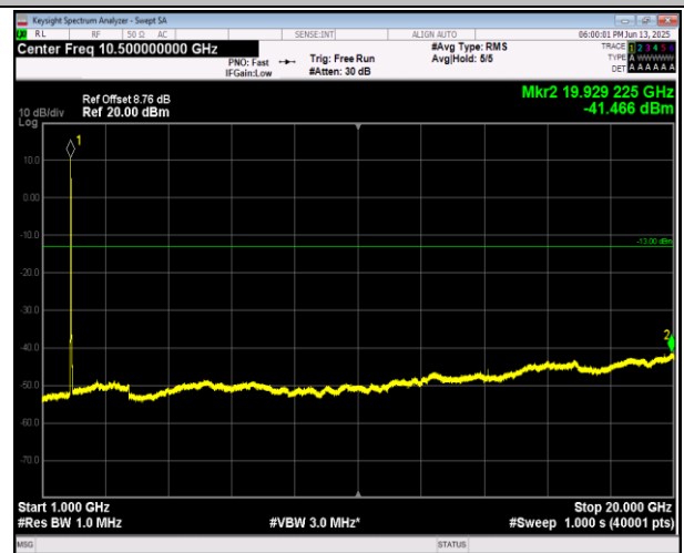
2-2-5MHz-20MHz-QPSK-QPSK-18808-18925-1RB#0-0RB# 0-1000~20000MHz-PASS
