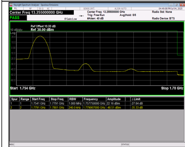
66-66-20MHz-5MHz-QPSK@QPSK-QPSK@QPSK-1320
