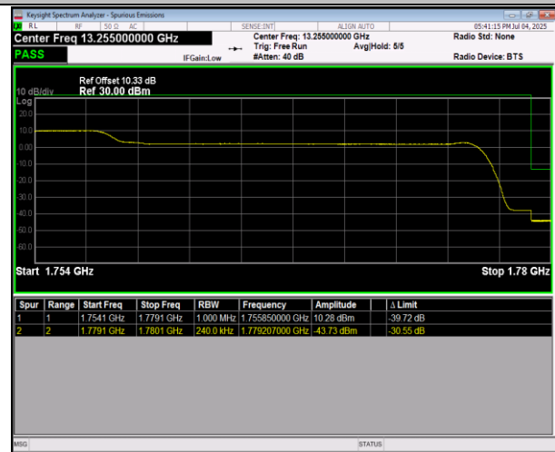
66-66-20MHz-5MHz-QPSK@QPSK-QPSK@QPSK-132072
