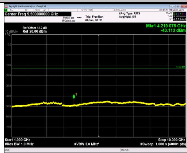
5-5-3MHz-5MHz-QPSK-QPSK-20586-20625-15RB#0-25RB #0-1000~10000MHz-PASS
