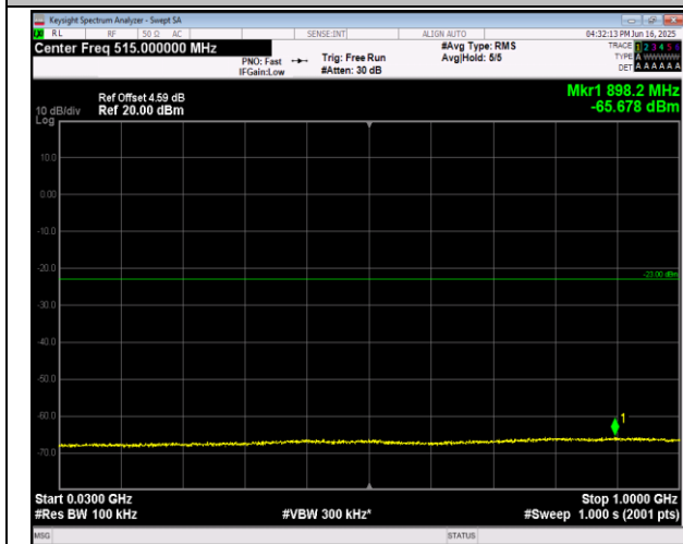
2-2-20MHz-20MHz-QPSK-QPSK-18902-19100-1RB#0-0-1 RB#99-30~1000MHz-PASS
