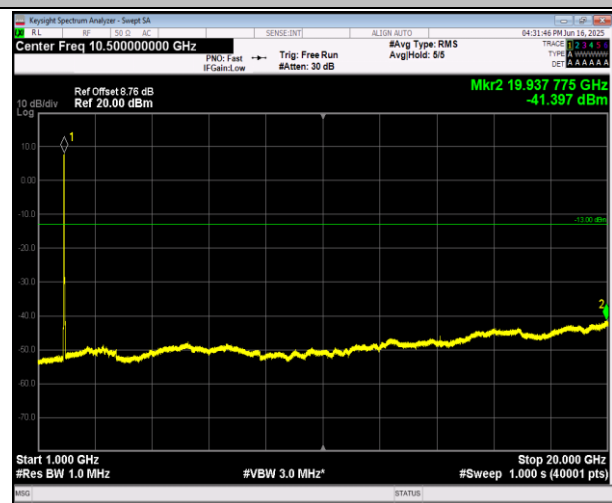
2-2-20MHz-20MHz-QPSK-QPSK-18902-19100-1RB#0-0RB #0-1000~20000MHz-PASS
