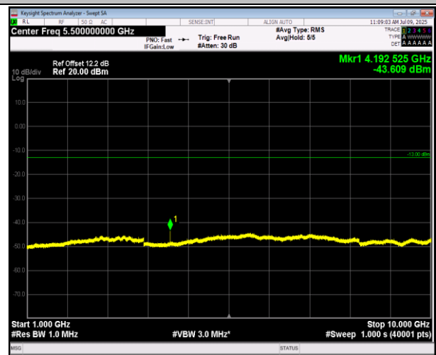
5-5-10MHz-10MHz-QPSK-QPSK-20501-20600-50RB#0-50 RB#0-1000~10000MHz-PASS
