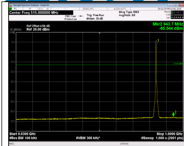
5-5-5MHz-3MHz-QPSK-QPSK-20425-20464-1RB#0-0RB #0-30~1000MHz-PASS
