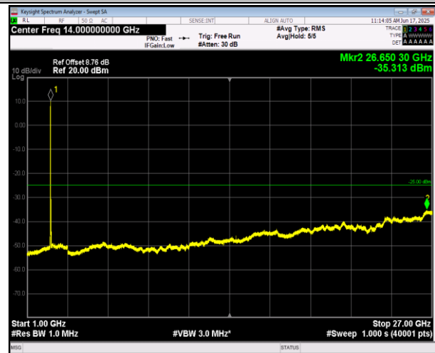
7-7-20MHz-10MHz-QPSK-QPSK-20850-20994-1RB#99-0RB B#0-1000~27000MHz-PASS
