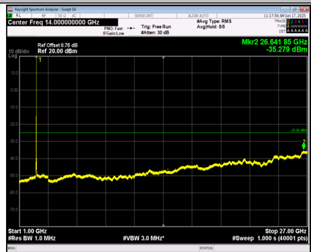
7-7-20MHz-10MHz-QPSK-QPSK-21051-21195-100RB#0-5 ORB#0-1000~27000MHz-PASS
