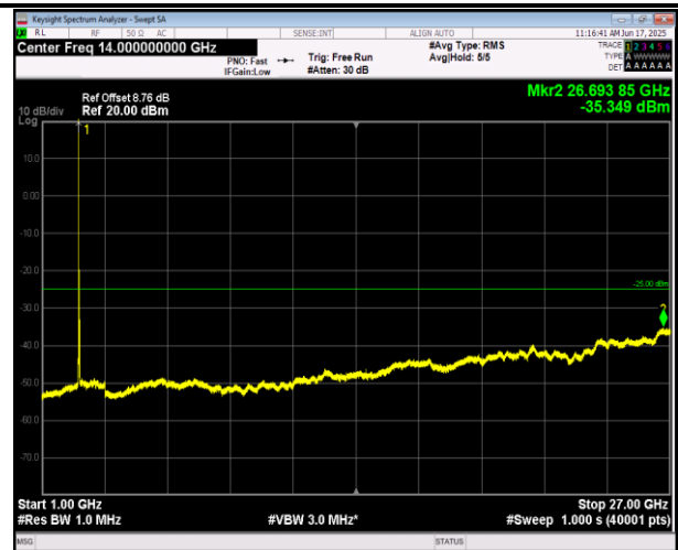
7-7-20MHz-10MHz-QPSK-QPSK-21051-21195-1RB#0-1RB #49-1000~27000MHz-PASS
