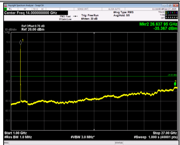
7-7-20MHz-10MHz-QPSK-QPSK-21051-21195-1RB#0-0RB #0-1000~27000MHz-PASS
