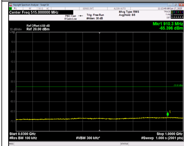
7-7-20MHz-10MHz-QPSK-QPSK-20850-20994-1RB#99-0 RB#0-30~1000MHz-PASS
