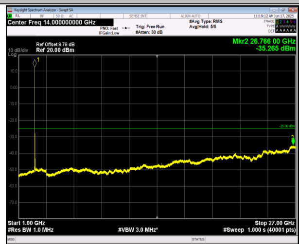
7-7-20MHz-10MHz-QPSK-QPSK-21051-21195-1RB#99-0R B#0-1000~27000MHz-PASS
