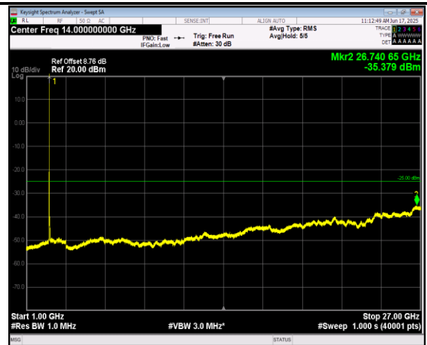
7-7-20MHz-10MHz-QPSK-QPSK-20850-20994-100RB#0-50RB#0-1000~27000MHz-PASS
