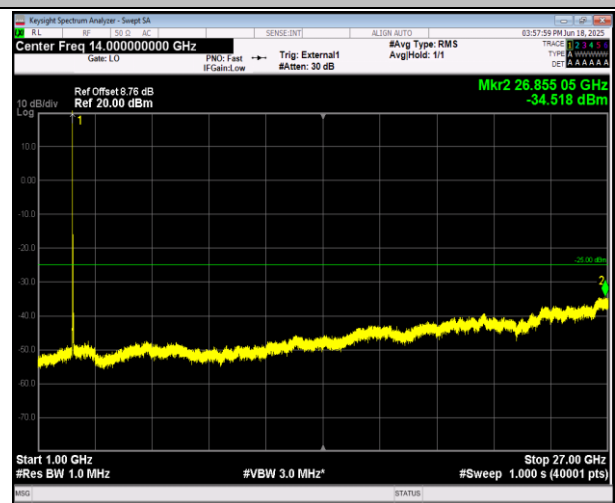
38-38-20MHz-20MHz-QPSK-QPSK-37901-38099-1RB#99-0RB#0-1000~27000MHz-PASS
