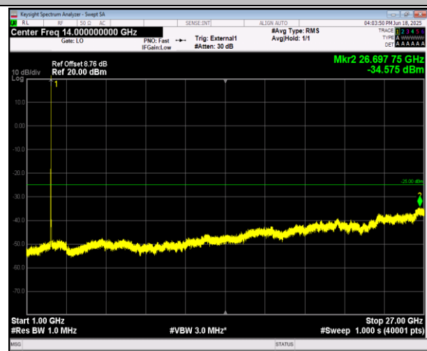
38-38-20MHz-20MHz-QPSK-QPSK-37952-38150-100RB#0 -100RB#0-1000~27000MHz-PASS
