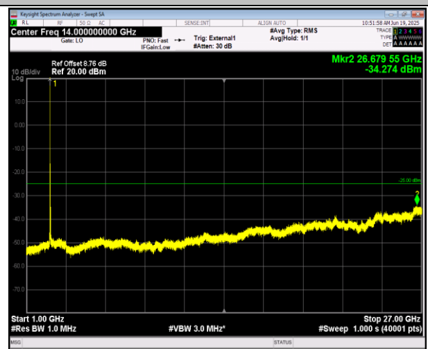
41(2555-2655)-41(2555-2655)-10MHz-15MHz-QPSK-QPS K-40293-40413-1RB#0-1RB#74-1000~27000MHz-PASS
