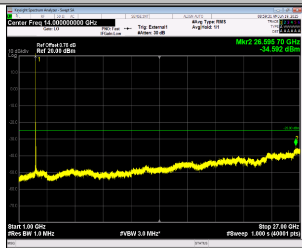
41(2555-2655)-41(2555-2655)-5MHz-20MHz-QPSK-QPSK- 40273-40390-1RB#0-1RB#99-1000~27000MHz-PASS
