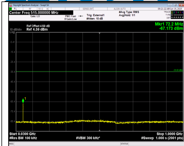
41(2555-2655)-41(2555-2655)-10MHz-15MHz-QPSK-QP SK-40293-40413-1RB#0-ORB#0-30~1000MHz-PASS
