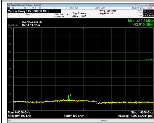
41(2555-2655)-41(2555-2655)-10MHz-15MHz-QPSK-QP SK-40293-40413-1RB#0-1RB#74-30~1000MHz-PASS
