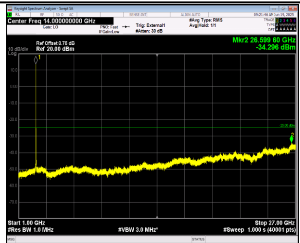
41(2555-2655)-41(2555-2655)-10MHz-15MHz-QPSK-QPS K-40293-40413-1RB#0-ORB#0-1000~27000MHz-PASS
