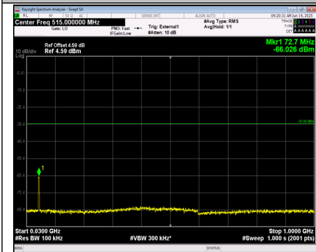
41(2555-2655)-41(2555-2655)-5MHz-20MHz-16QAM-16 QAM-41023-41140-1RB#0-0RB#0-30~1000MHz-PASS
