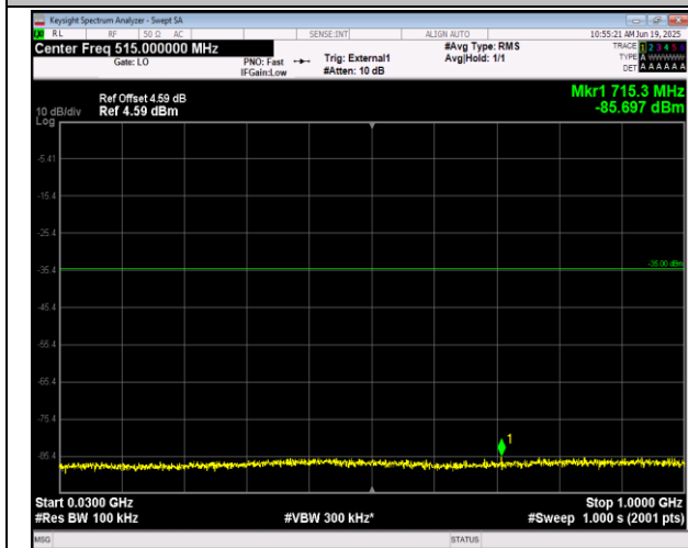
41(2555-2655)-41(2555-2655)-10MHz-15MHz-QPSK-QP SK-40293-40413-1RB#49-ORB#0-30~1000MHz-PASS
