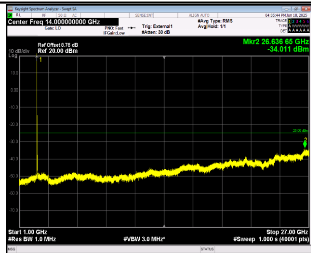
38-38-20MHz-20MHz-QPSK-QPSK-37952-38150-1RB#99- 0RB#0-1000~27000MHz-PASS
