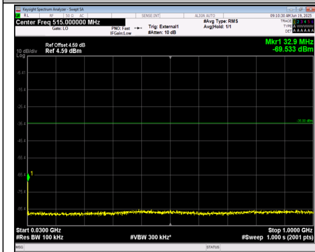
41(2555-2655)-41(2555-2655)-5MHz-20MHz-QPSK-QPS K-40648-40765-1RB#24-0RB#0-30~1000MHz-PASS
