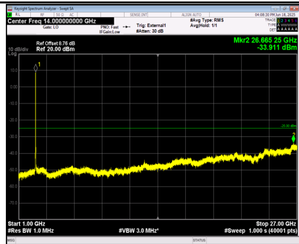
41(2555-2655)-41(2555-2655)-5MHz-20MHz-QPSK-QPSK- 40273-40390-1RB#0-0RB#0-1000~27000MHz-PASS
