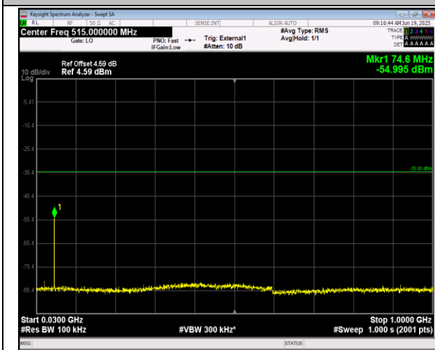
41(2555-2655)-41(2555-2655)-5MHz-20MHz-QPSK-QPS K-41023-41140-25RB#0-100RB#0-30~1000MHz-PASS
