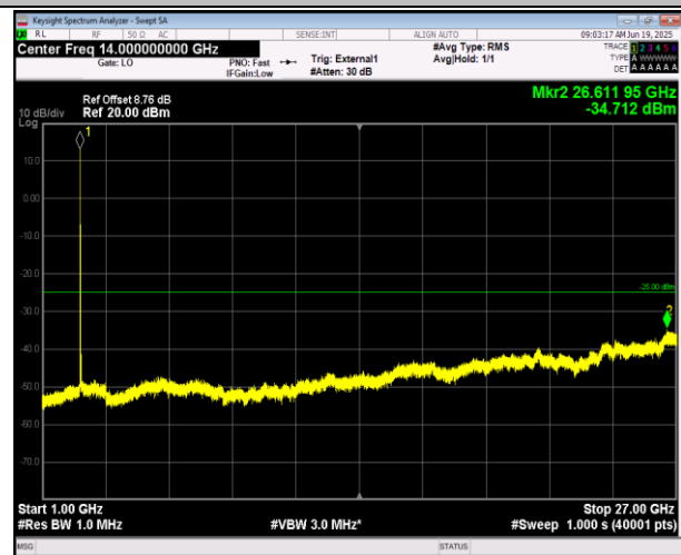
41(2555-2655)-41(2555-2655)-5MHz-20MHz-QPSK-QPSK- 40273-40390-1RB#24-0RB#0-1000~27000MHz-PASS
