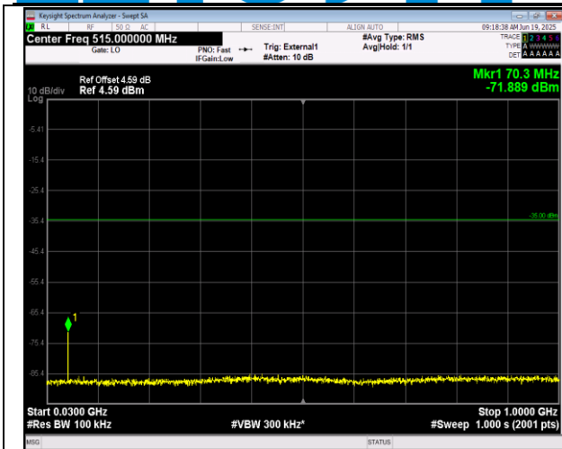
41(2555-2655)-41(2555-2655)-5MHz-20MHz-QPSK-QPS K-41023-41140-1RB#24-0RB#0-30~1000MHz-PASS
